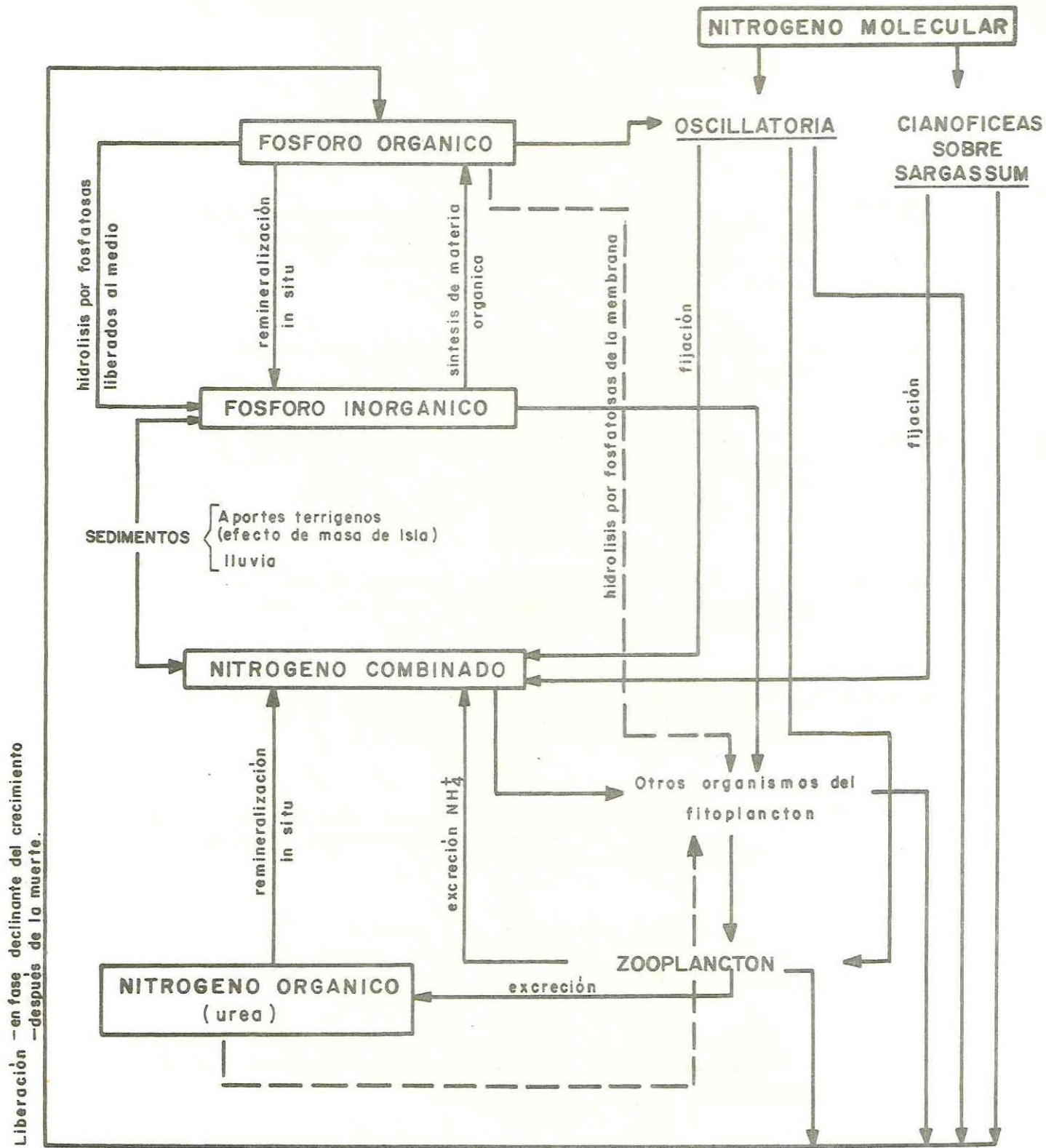
FIGURA.9. FLUJO PROBABLE DE NITROGENO Y FOSFORO EN LA ZONA FOTICA. CRUCERO OCEANO VI - JUNIO 1983.
