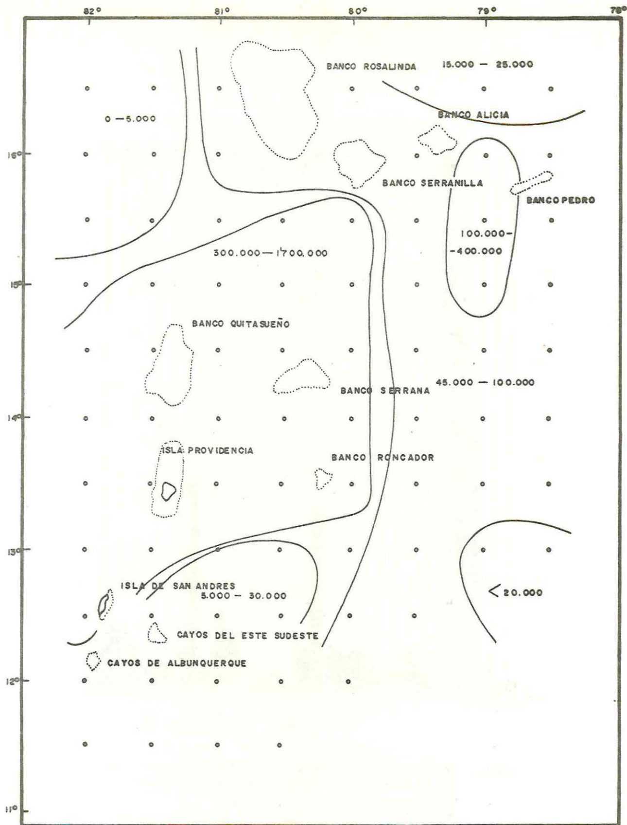
FIGURA. 7. DISTRIBUCION SUPERFICIAL ABUNDANCIA TOTAL DE CIANOFICEAS (cels/m 3 ). CADA COLONIA TIENE APROXIMADAMENTE 20.000 CELULAS. CRUCERO OCEANO VI - JUNIO 1983.
