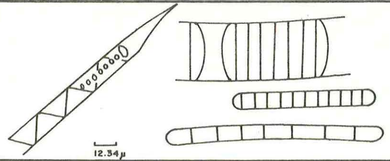
FIGURA. 8. FORMAS CARACTERISTICAS DE LAS ESPECIES FITOPLANCTONICAS EN EL SISTEMA PELAGICO DE PROVIDENCIA Y STA. CATALINA QUE REFLEJAN LA ADAPTACION A LAS CONDICIONES DE ESTRATIFICACION Y BAJO CONTENIDO DE NUTRIENTES.
