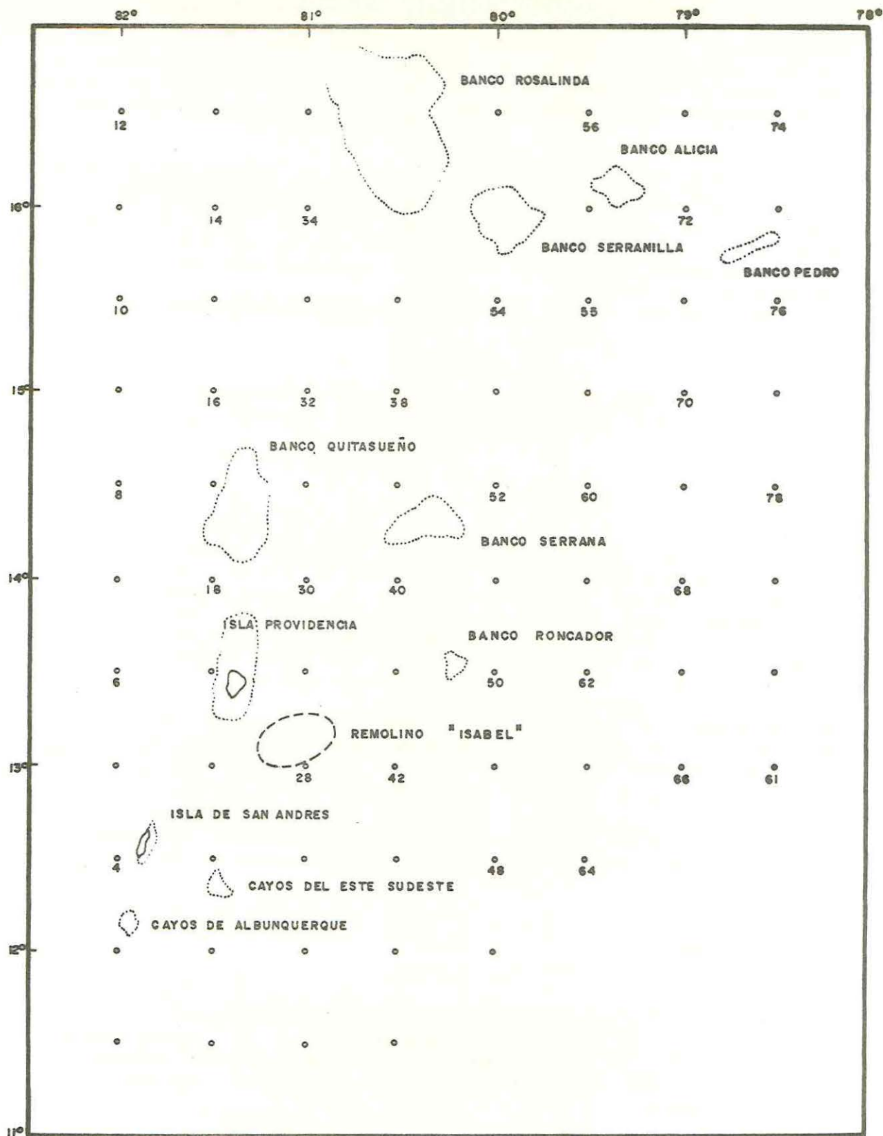
FIGURA 2 ESTACIONES DE MUESTREO Y UBICACION DEL REMOLINO "ISABEL". LAS ESTACIONES NUMERADAS CORRESPONDEN A AQUELLAS EN QUE SE COLECTO FITOPLANCTON. CRUCERO OCEANO VI - JUNIO 1983.
