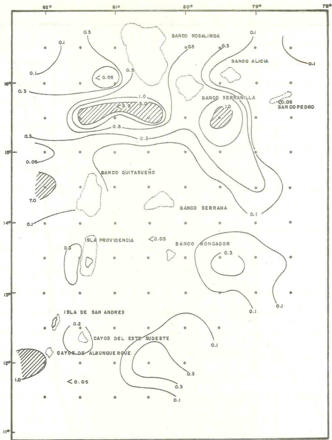
FIGURA 4. DISTRIBUCION SUPERFICIAL NITRATOS ( \mu\text{g-atN-NO}_3^-/\text{lt} ). (MODIFICADO DE MAPA ELABORADO POR EL CIOH.) CRUCERO OCEANO VI - JUNIO 1983.
