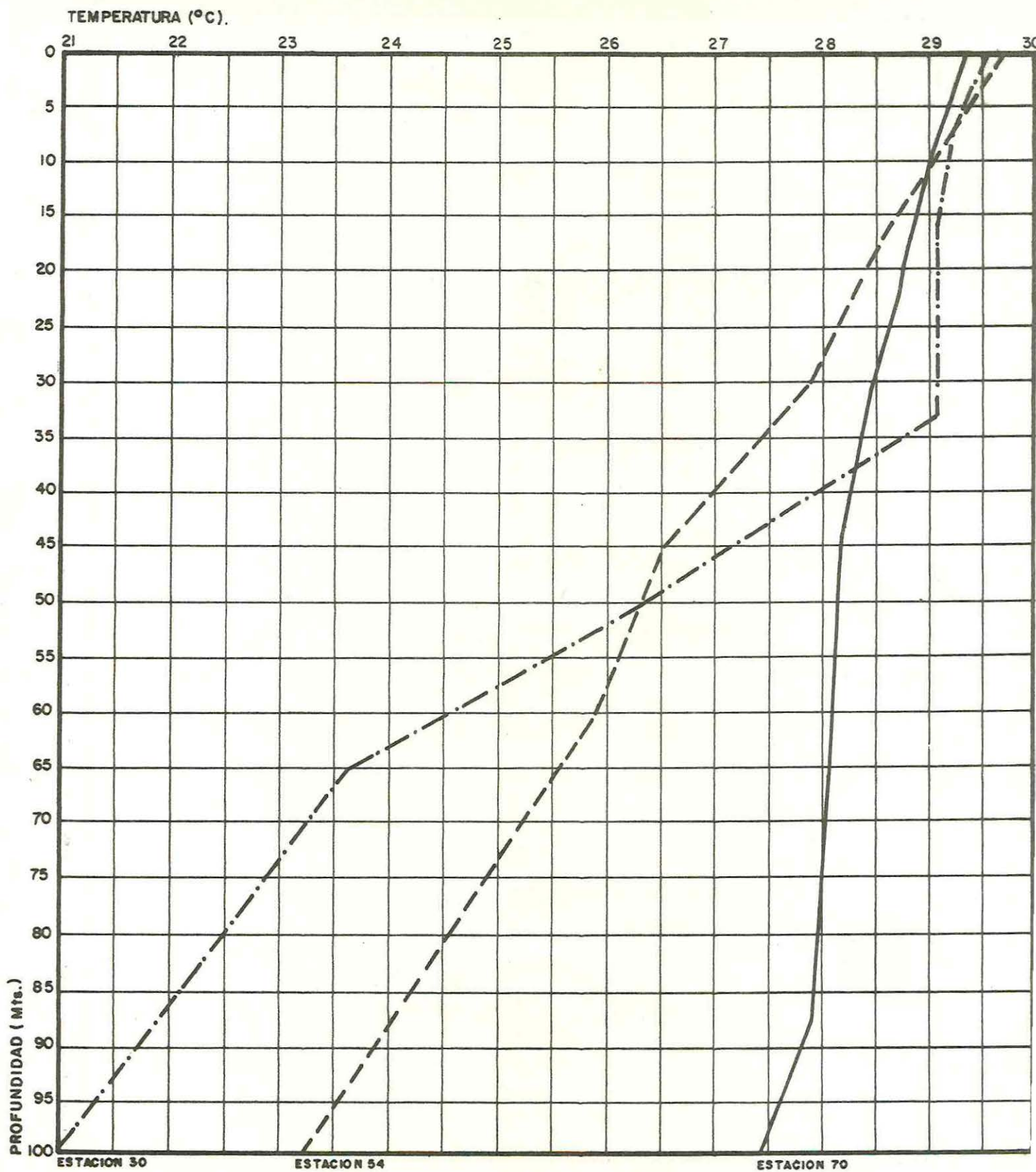
FIGURA 3. PERFILES TIPO DE TEMPERATURA (°C.). (Explicación en el texto). CRUCERO OCEANO VI - JUNIO 1983.
