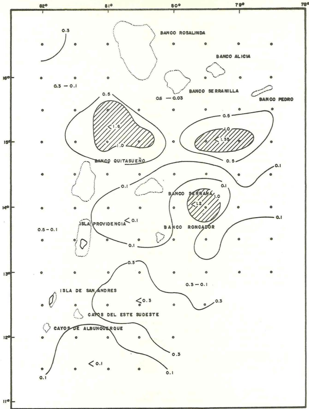
FIGURA 5. DISTRIBUCION SUPERFICIAL FOSFATOS ( \mu\text{g-atP-PO}_4^{3-}/\text{lt.} ). (MODIFICADO DE MAPA ELABORADO POR EL CIOH.).
