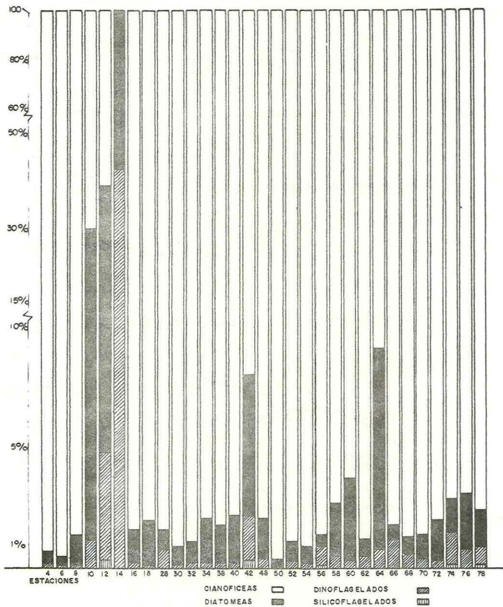
FIGURA. 6. COMPOSICION DEL FITOPLANCTON EXPRESADO COMO PORCENTAJE DEL TOTAL DE CELULAS EN CADA ESTACION. CRUCERO OCEANO VI - JUNIO 1983
