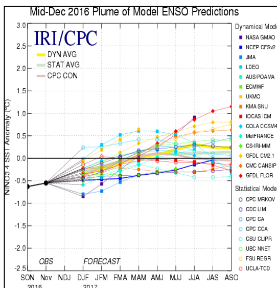
Figura 3. Pronóstico ENSO (Fuente: (IRI/CPC, 2017)).
