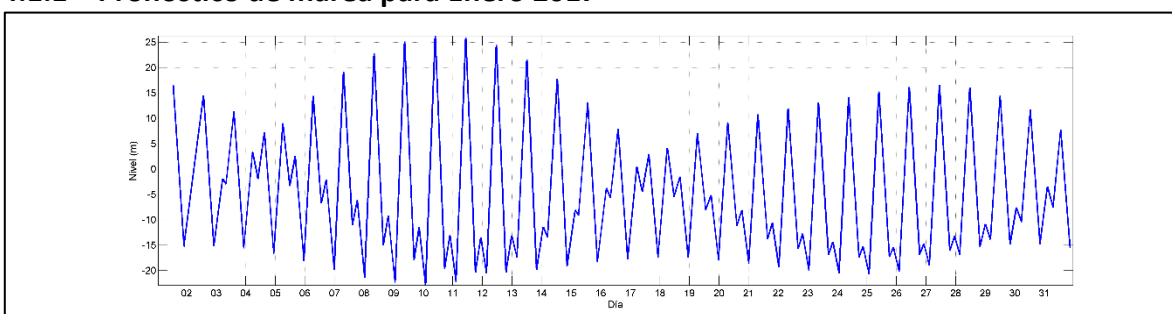
Figura 14. Pronóstico de marea para Enero de 2017, Cartagena. (Torres Parra & Otero Diaz, 2008)
