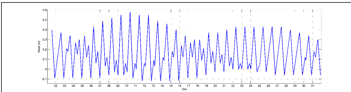
Figura 15. Pronóstico de marea para Enero de 2017 en (Puerto Colombia) Atlántico. (Ideam, 2017)
