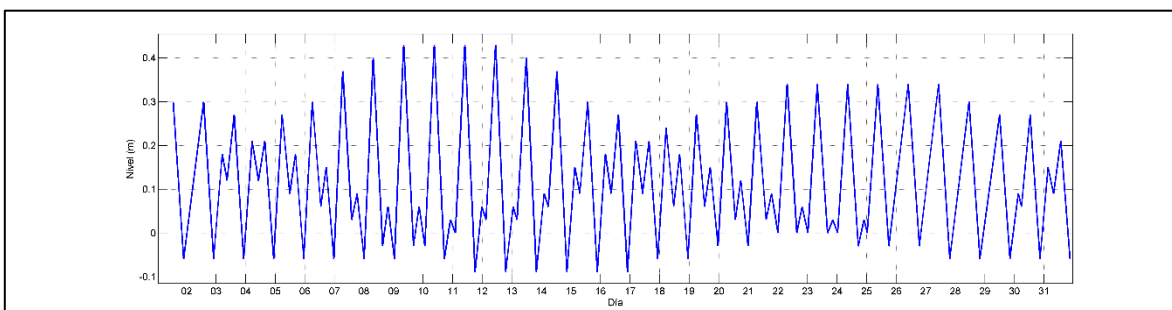
Figura 16. Pronostico de marea para Enero de 2017 en Santa Marta. (Ideam, 2017)
