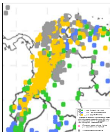
Figura 5. Pronóstico de precipitación para el mes de Enero de 2017 (Fuente: (CIIFEN ( . I., 2017)).
