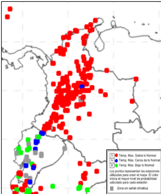
Figura 9. Pronóstico temperatura máxima para Enero de 2017 (Fuente: (CIIFEN (. I., 2017)).
