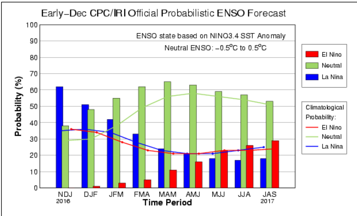
Figura 4. Pronóstico de las condiciones ENSO esperadas para el lapso noviembre de 2016 hasta septiembre de 2017 (Fuente: (IRI/CPC, 2017)).
