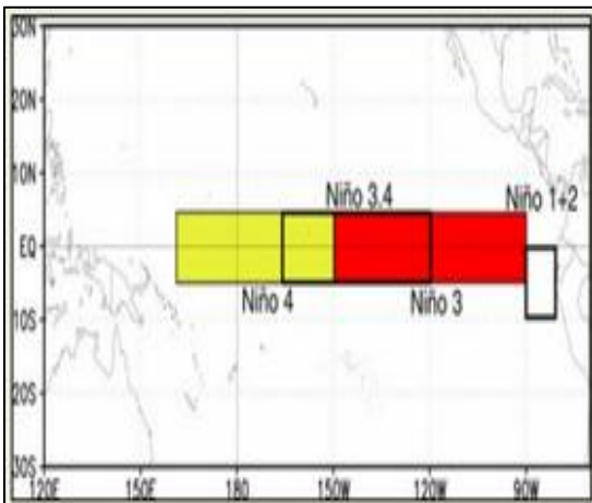
Figura 1. Regiones de "El Niño". (Fuente: (CPC-NCEP, 2017))
