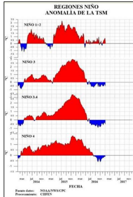
Figura 2. Anomalías TSM en cada una de las regiones de "El Niño" (Fuente: (CPC-NCEP, 2017)).
