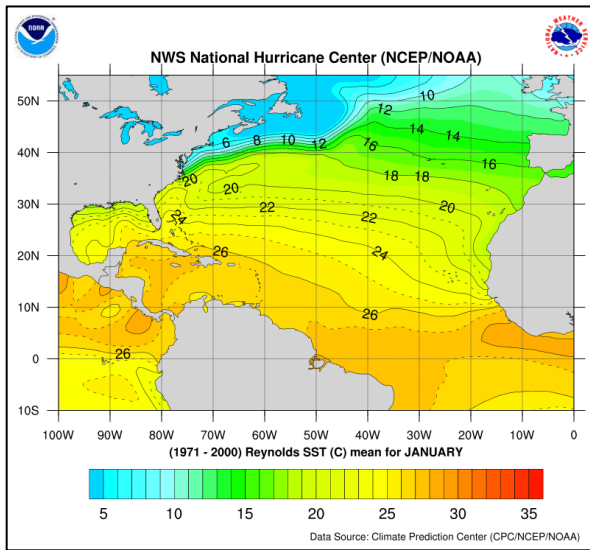
Figura 12. Pronóstico de TSM para Enero de 2017 (Fuente: (NHC, 2017)).
