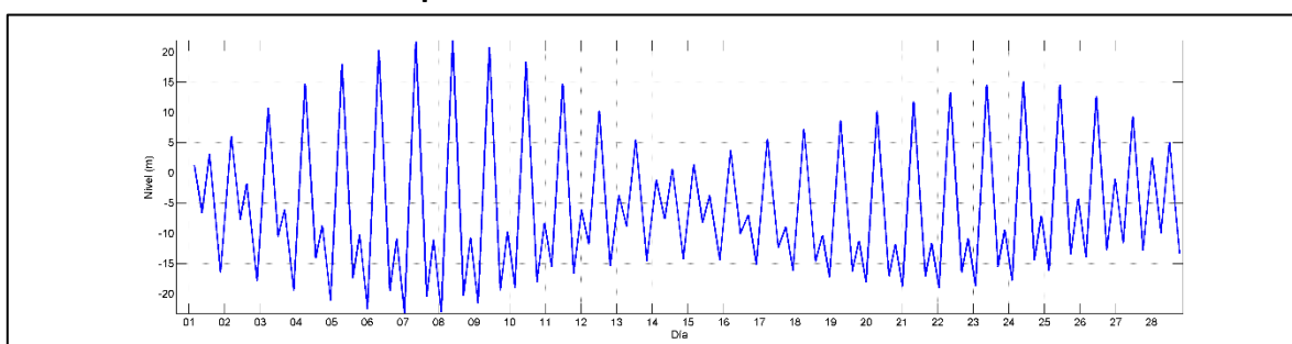
Figura 14. Pronóstico de marea para Febrero de 2017, Cartagena. (Torres Parra & Otero Diaz, 2008)
