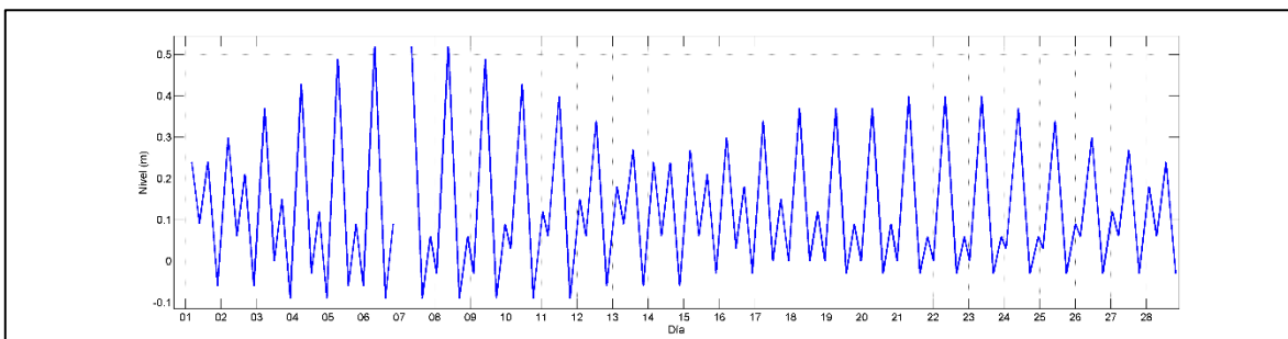
Figura 15. Pronóstico de marea para Febrero de 2017 en (Puerto Colombia) Atlántico. (Ideam, 2017)
