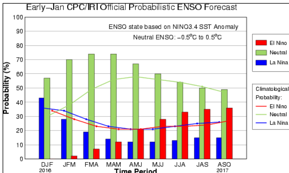
Figura 4. Pronóstico de las condiciones ENSO esperadas para el lapso diciembre de 2016 hasta octubre de 2017 (Fuente: (IRI/CPC, 2017)).
