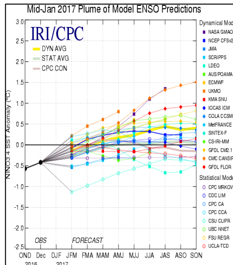
Figura 3. Pronóstico ENSO (Fuente: (IRI/CPC, 2017)).
