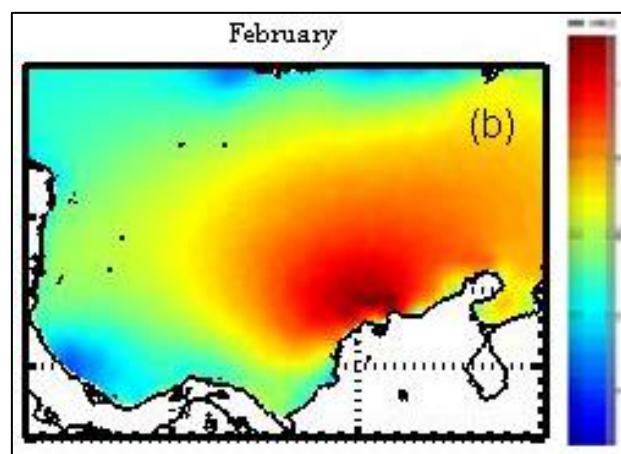
Figura 6. Promedio multianual velocidad del viento (m/s) mes de Febrero. (Appendini, 2014)
