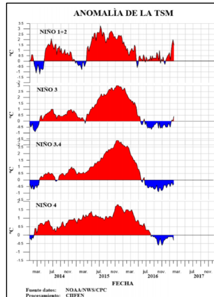
Figura 2. Anomalías TSM en cada una de las regiones de "El Niño" (Fuente: (CPC-NCEP, 2017)).
