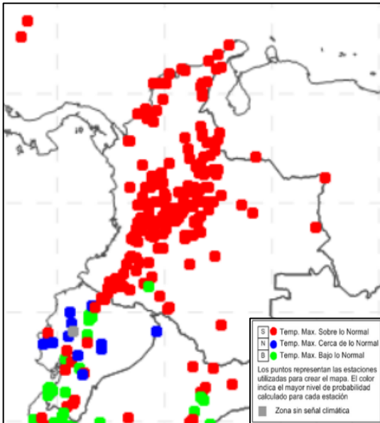
Figura 9. Pronóstico temperatura máxima para Febrero de 2017 (Fuente: (CIIFEN (. I., 2017))).
