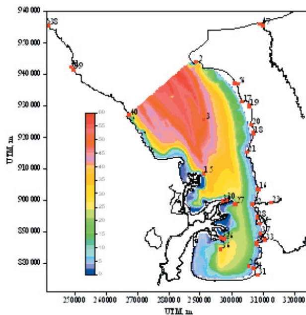
Figura 1. Batimetría del Golfo de Urabá (en metros) en el dominio del modelo y los puntos de mediciones de coliformes fecales, correspondientes a la Tabla 3 (algunos de los puntos de la Tabla 3 se encuentran ubicados fuera de los límites del dominio).
