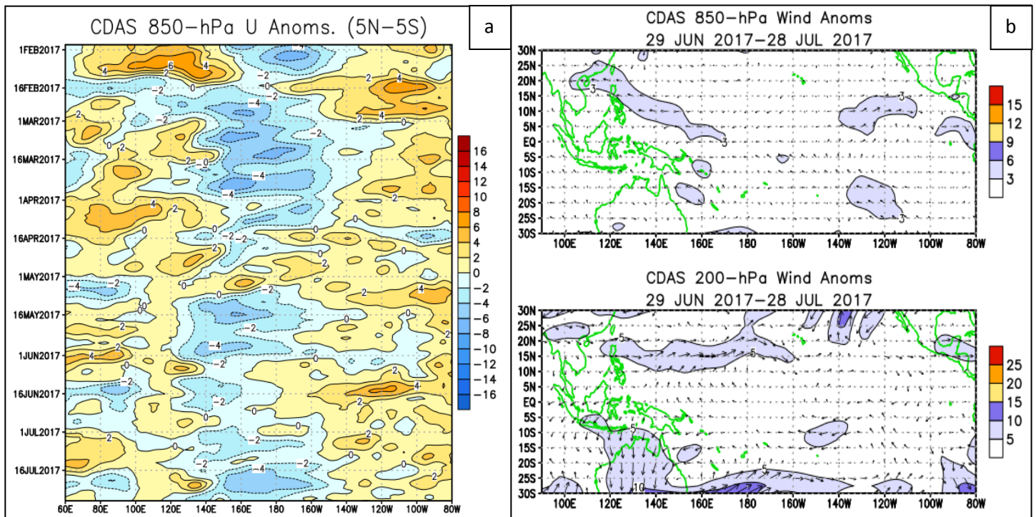
Figura 7. Anomalías campos de vientos sobre el Océano Pacífico Ecuatorial (OPE) para el mes de julio del 2017. Fuente: Climate Prediction Center_ NOAA.
