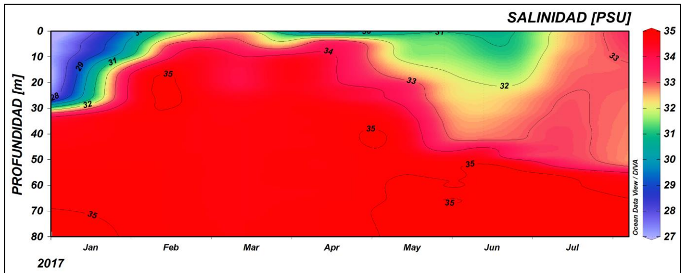
Figura 12. Serie temporal de salinidad del agua en la estación costera No. 5 entre 0 a 80 metros de profundidad, para el periodo comprendido entre enero y julio del 2017. Fuente: CCCP.
