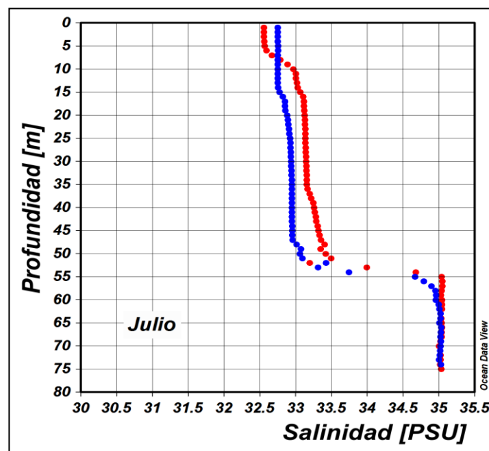
Figura 13. Perfil de salinidad para el mes de julio del 2017 en la estación costera fija de Tumaco. En color rojo se presenta el perfil obtenido en la primera quincena del mes y en azul el realizado a finales del mismo. Fuente: CCCP.
