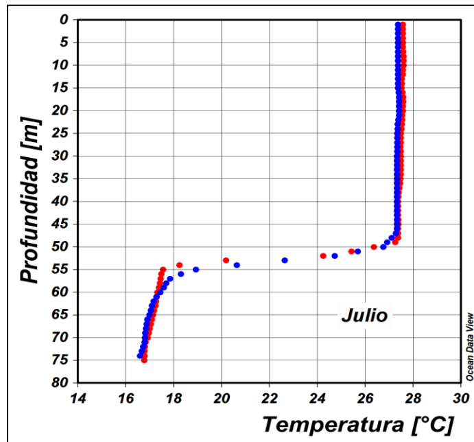
Figura 11. Perfil de temperatura para el mes de julio del 2017 registrado en la estación costera fija de Tumaco. En color rojo se presenta el perfil obtenido en la primera quincena del mes y en azul el realizado a finales del mismo. Fuente: CCCP.
