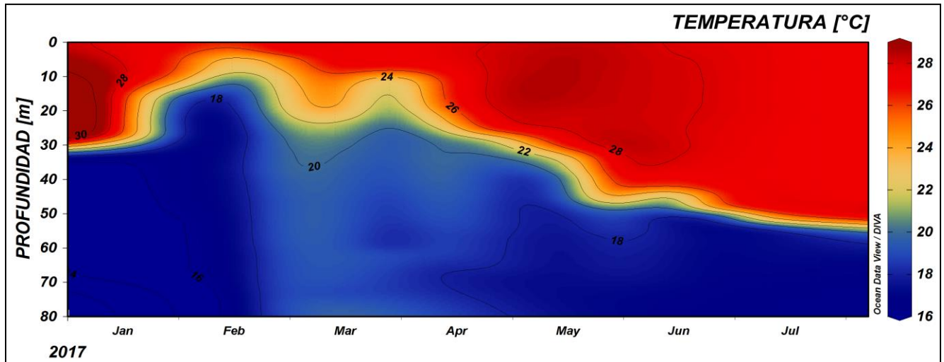
Figura 10. Serie temporal de temperatura del agua en la estación costera fija de Tumaco entre 0 a 80 metros de profundidad, para el periodo comprendido entre enero y julio del 2017. La escala de colores representa la magnitud de la temperatura medida en °C. Fuente: CCCP.
