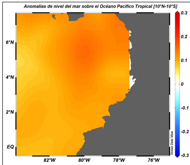
Figura 6. Anomalías de nivel del mar CPC, julio del 2017 (Fuente: Copernicus Marine Service (CMEMS), Procesamiento: CIOHP).
