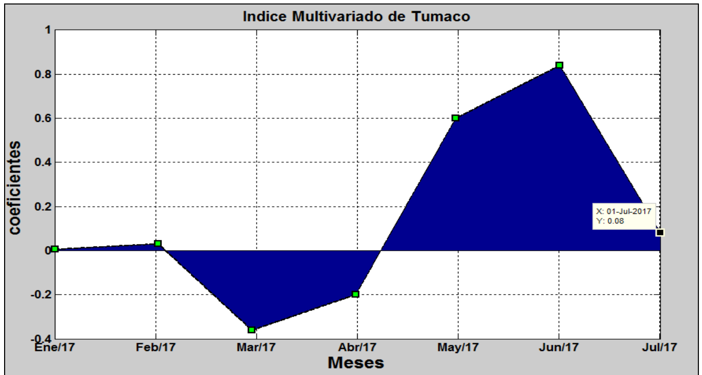
Figura 14. Comportamiento del Índice Multivariado de Tumaco (IMT) para el periodo comprendido entre enero y julio del 2017. Fuente: CCCP.
