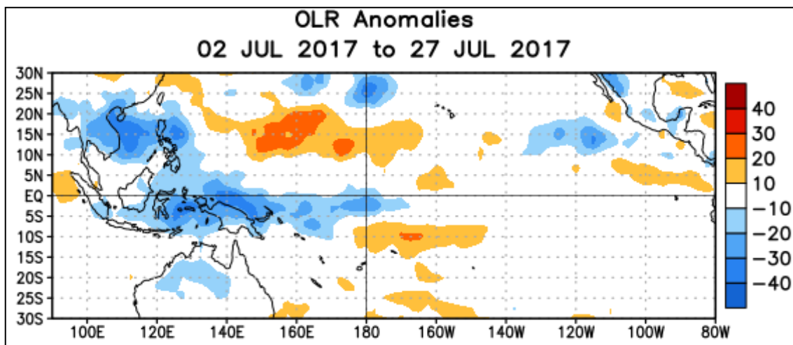
Figura 8. Anomalías Radiación de Onda Larga (OLR, por sus siglas en inglés) Para el mes de julio del 2017. La escala de colores representa la magnitud de las anomalías en W/m^2 . Fuente: Climate Prediction Center- NOAA.
