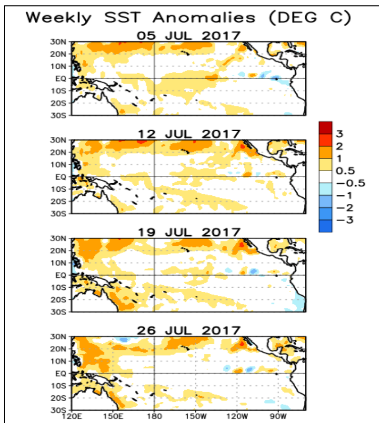
Figura 3. Anomalías semanales de TSM en el Océano Pacífico Tropical para el periodo comprendido entre el 05 y el 26 de julio del 2017. Fuente: Climate Prediction Center-NOAA.
