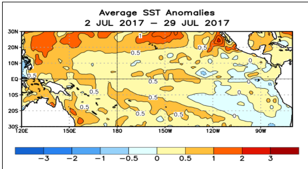
Figura 2. Anomalías de TSM en el Océano Pacífico Tropical para el periodo comprendido entre el 02 de julio y el 29 de julio del 2017. La escala de colores representa la magnitud en °C. Fuente: Climate Prediction Center - NOAA.
