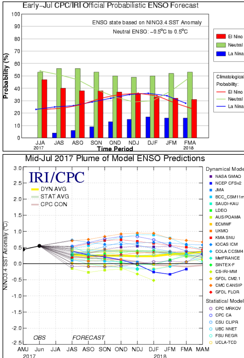
Figura 15. Predicción modelos estadísticos y dinámicos de condiciones ENOS 13 de julio del 2017. (Fuente: IRI/CPC).
