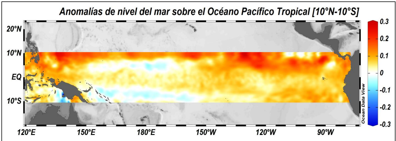
Figura 5. Anomalías de nivel del mar Océano Pacífico Tropical para el mes de julio del 2017. La escala de colores representa la magnitud media en metros (m) (Fuente: Copernicus Marine Service (CMEMS), Procesamiento: CIOHP).
