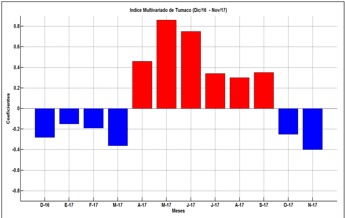
Figura 14. Comportamiento del Índice Multivariado de Tumaco (IMT) para el periodo comprendido entre diciembre del 2016 y noviembre del 2017. Fuente: CCCP.
