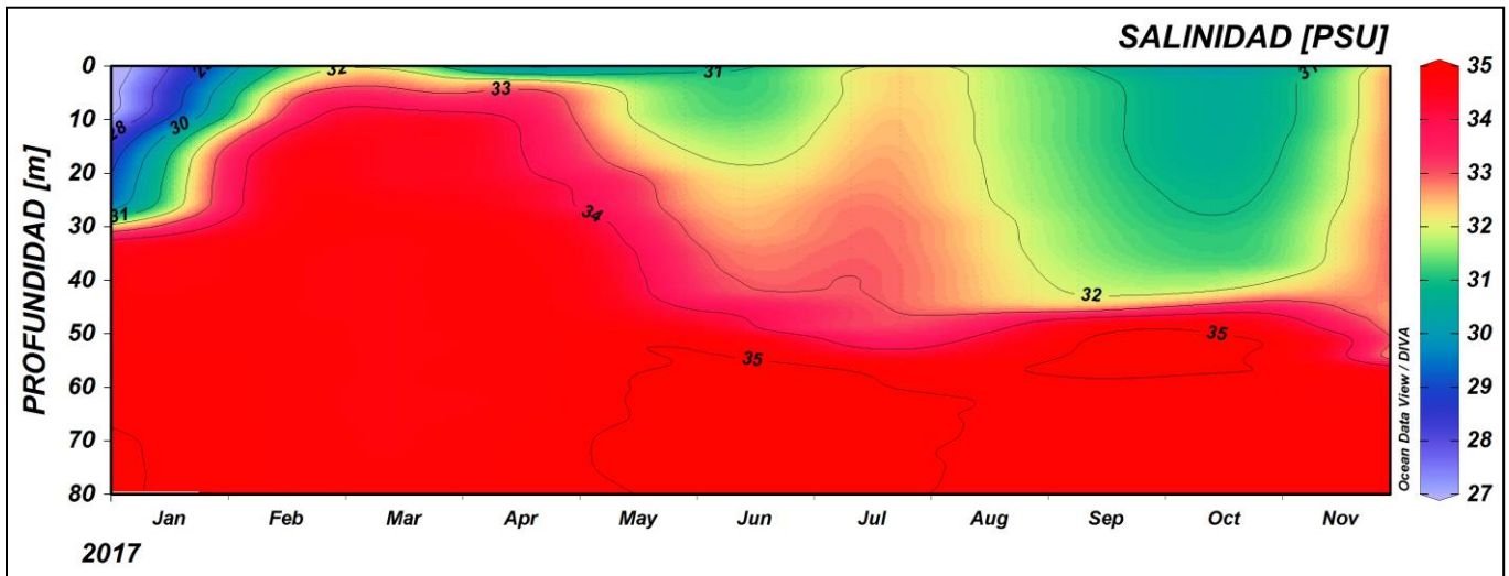
Figura 12. Serie temporal de salinidad del agua en la estación costera fija de Tumaco entre 0 a 80 metros de profundidad, para el periodo de comprendido entre enero y noviembre del 2017. Fuente: CCCP.
