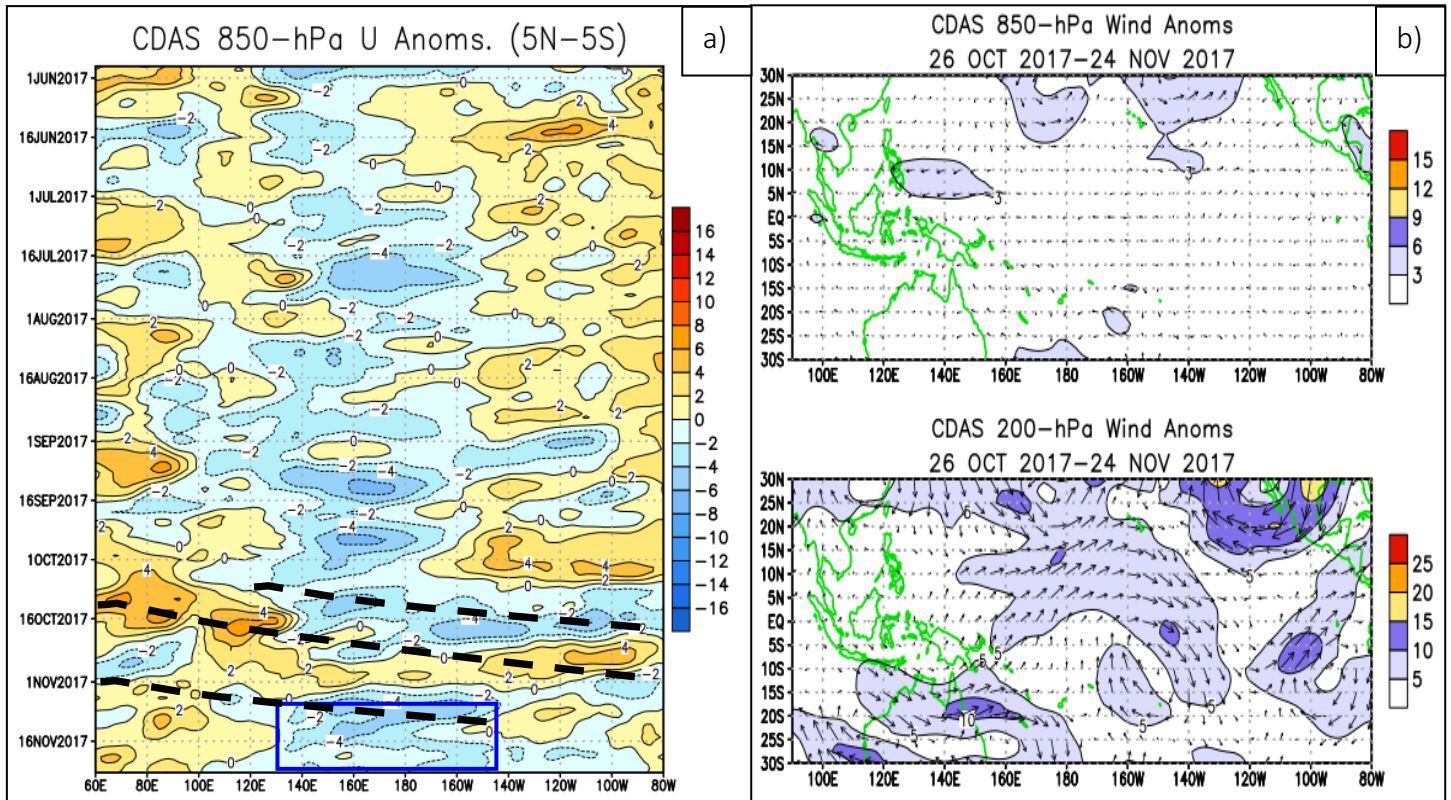
Figura 7. Anomalías campos de vientos sobre el Océano Pacífico Ecuatorial (OPE) para el mes de noviembre del 2017. Fuente: Climate Prediction Center_ NOAA.
