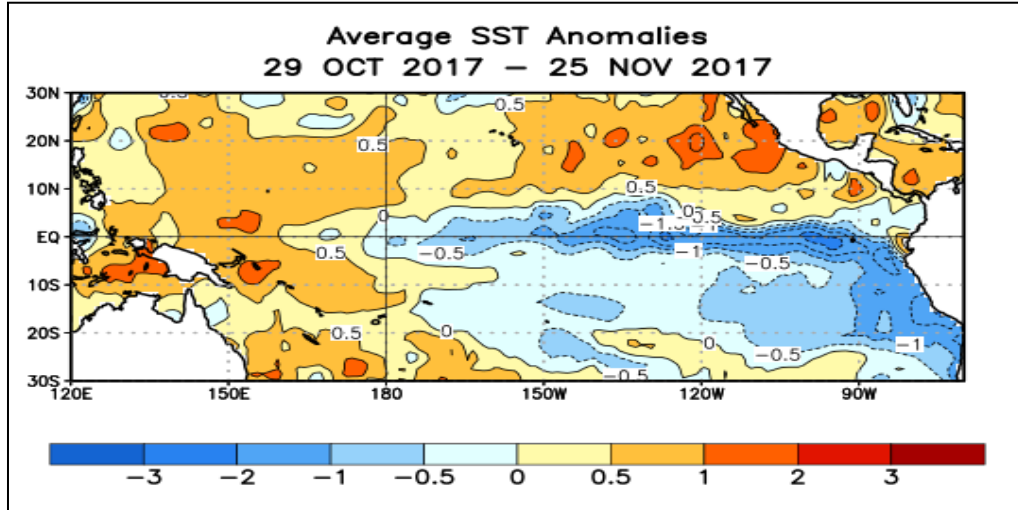
Figura 2. Anomalías de TSM en el Océano Pacífico Tropical para el periodo comprendido entre el 29 de octubre y el 25 de noviembre del 2017. La escala de colores representa la magnitud en °C. Fuente: Climate Prediction Center - NOAA.
