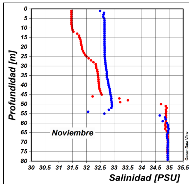
Figura 13. Perfil de salinidad para el mes de noviembre del 2017 en la estación costera fija de Tumaco. En color rojo se presenta el perfil obtenido en la primera quincena del mes y en azul el realizado a finales del mismo. Fuente: CCCP.
