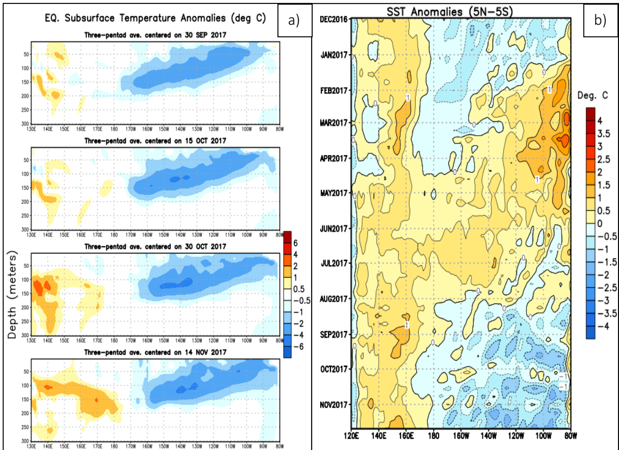
Figura 1. Evolución de las anomalías de temperatura subsuperficial (a) en el Océano Pacífico Ecuatorial (OPE) y superficiales (b) entre latitudes 5°S y 5°N para el periodo comprendido entre el 30 de septiembre y el 14 de noviembre del 2017. La escala de colores representa la magnitud de las anomalías en °C. Fuente: Climate Prediction Center-NOAA.
