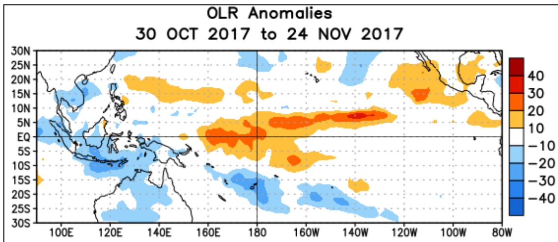
Figura 8. Anomalías Radiación de Onda Larga (OLR, por sus siglas en inglés) Para el mes de noviembre del 2017. La escala de colores representa la magnitud de las anomalías en W/m^2 . Fuente: Climate Prediction Center- NOAA.
