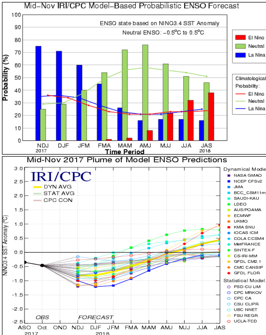
Figura 15. Predicción modelos estadísticos y dinámicos de condiciones ENOS 20 de noviembre del 2017. (Fuente: IRI/CPC).
