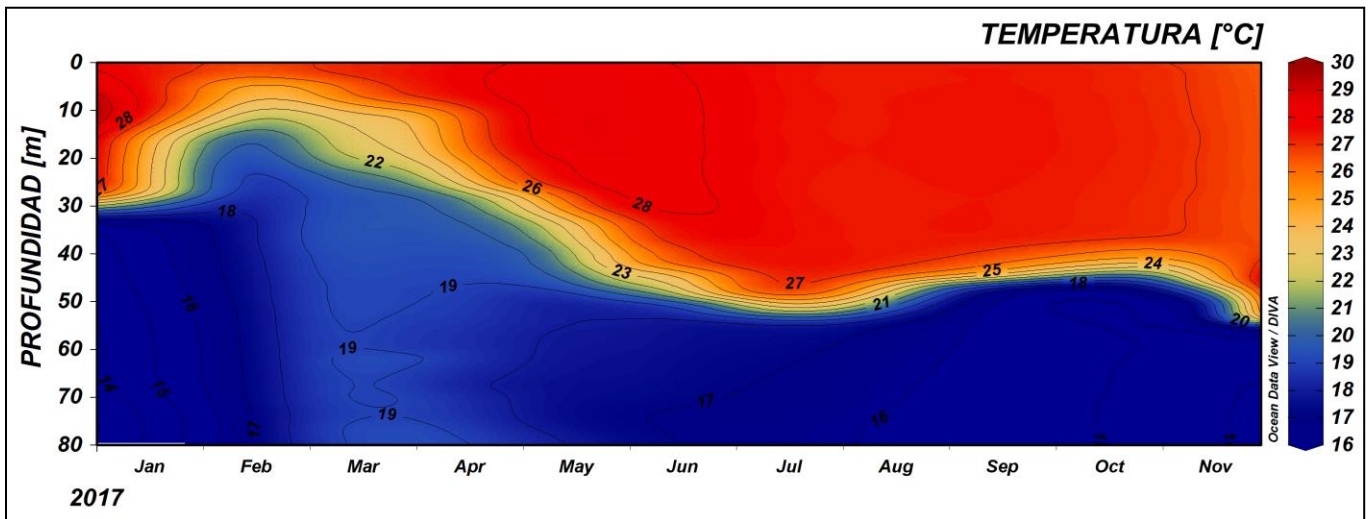
Figura 10. Serie temporal de temperatura del agua en la estación costera fija de Tumaco entre 0 a 80 metros de profundidad, para el periodo de comprendido entre enero y noviembre del 2017. La escala de colores representa la magnitud de la temperatura medida en °C. Fuente: CCCP.
