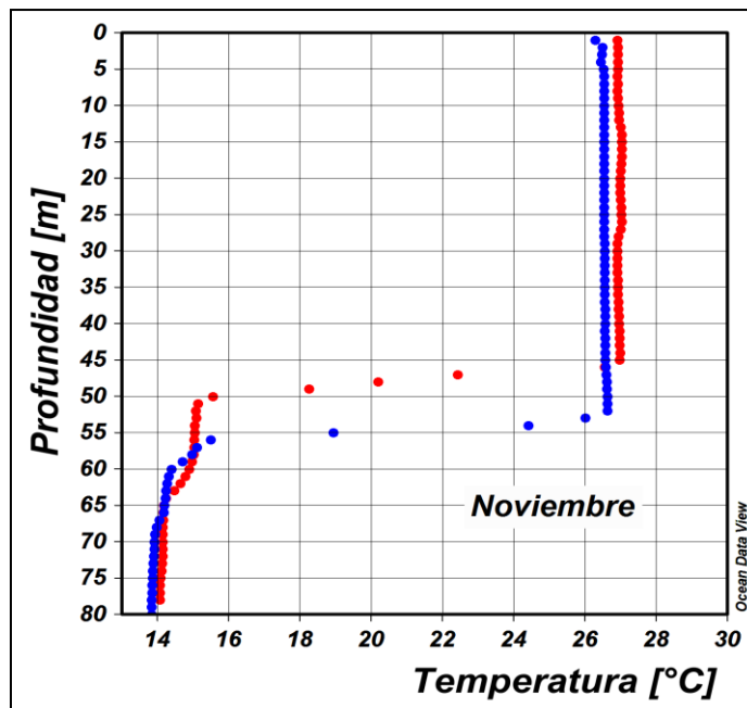
Figura 11. Perfil de temperatura para el mes de noviembre del 2017 registrado en la estación costera fija de Tumaco. En color rojo se presenta el perfil obtenido en la primera quincena del mes y en azul el realizado a finales del mismo. Fuente: CCCP.
