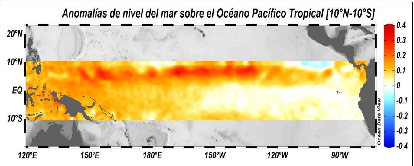
Figura 5. Anomalías de nivel del mar Océano Pacífico Tropical para el mes de noviembre del 2017. La escala de colores representa la magnitud media en metros (m) (Fuente: Copernicus Marine Service (CMEMS), Procesamiento: CIOHP).
