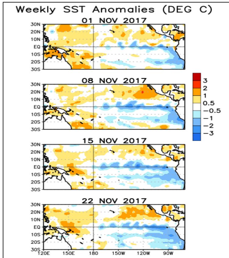
Figura 3. Anomalías semanales de TSM en el Océano Pacífico Tropical para el periodo comprendido entre el 01 y el 22 de noviembre del 2017. Fuente: Climate Prediction Center-NOAA.
