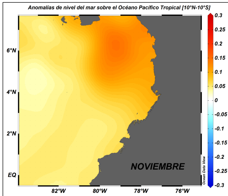
Figura 6. Anomalías de nivel del mar CPC, noviembre del 2017 (Fuente: Copernicus Marine Service (CMEMS), Procesamiento: CIOHP).
