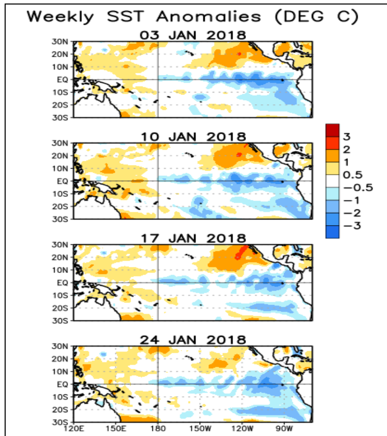
Figura 3. Anomalías semanales de TSM en el Océano Pacífico Tropical para el periodo comprendido entre el 03 y el 24 de enero del 2018. Fuente: Climate Prediction Center-NOAA.
