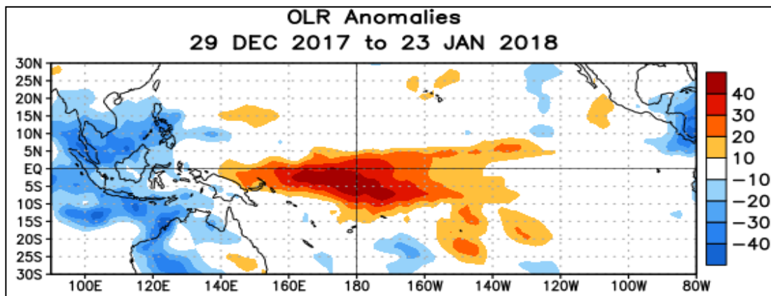
Figura 8. Anomalías Radiación de Onda Larga (OLR, por sus siglas en inglés) Para el mes de enero del 2018. La escala de colores representa la magnitud de las anomalías en W/m^2 . Fuente: Climate Prediction Center-NOAA.
