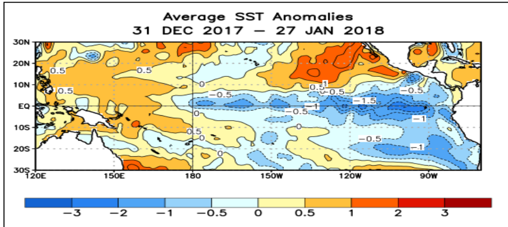
Figura 2. Anomalías de TSM en el Océano Pacífico Tropical para el periodo comprendido entre el 31 de diciembre del 2017 y el 27 de enero del 2018. La escala de colores representa la magnitud en ^{\circ}\text{C} . Fuente: Climate Prediction Center – NOAA.
