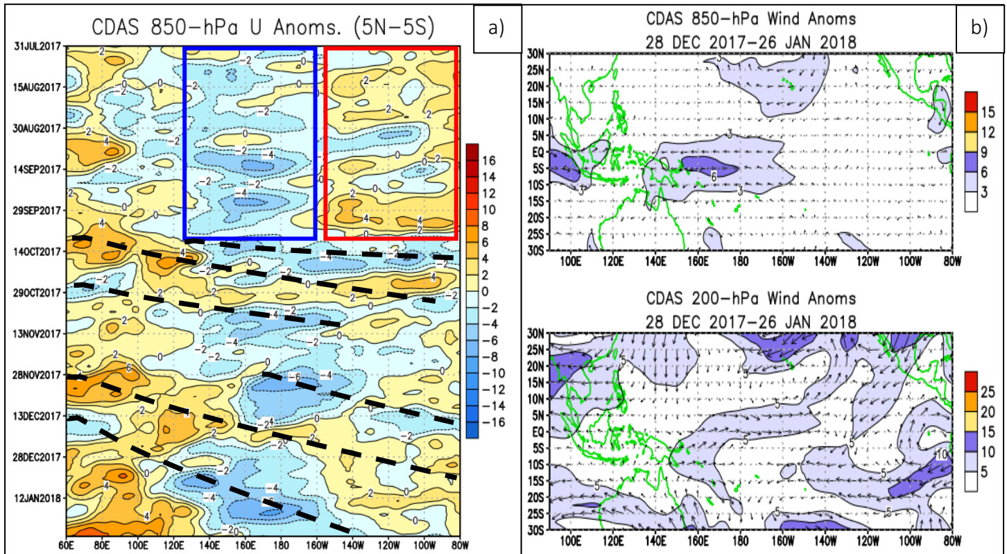
Figura 7. Anomalías campos de vientos sobre el Océano Pacífico Ecuatorial (OPE) para el mes de enero del 2018. Fuente: Climate Prediction Center-NOAA.
