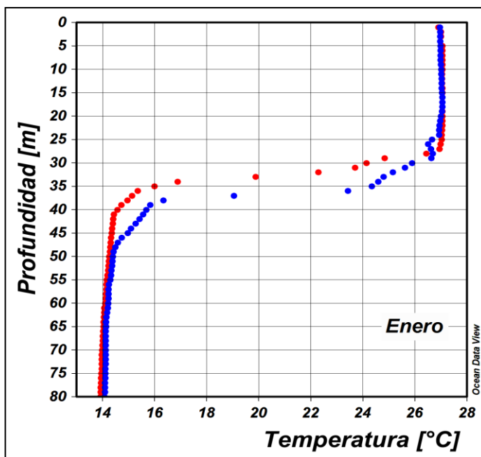
Figura 11. Perfil de temperatura para el mes de enero del 2018 registrado en la estación costera fija de Tumaco. En color rojo se presenta el perfil obtenido en la primera quincena del mes y en azul el realizado a finales del mismo. Fuente: CCCP.
