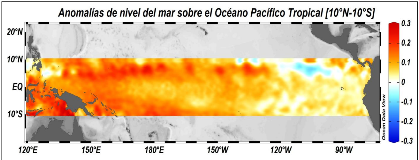
Figura 5. Anomalías de nivel del mar Océano Pacífico Tropical para el mes de enero del 2018. La escala de colores representa la magnitud media en metros (m) (Fuente: Copernicus Marine Service (CMEMS), Procesamiento: CIOHP).
