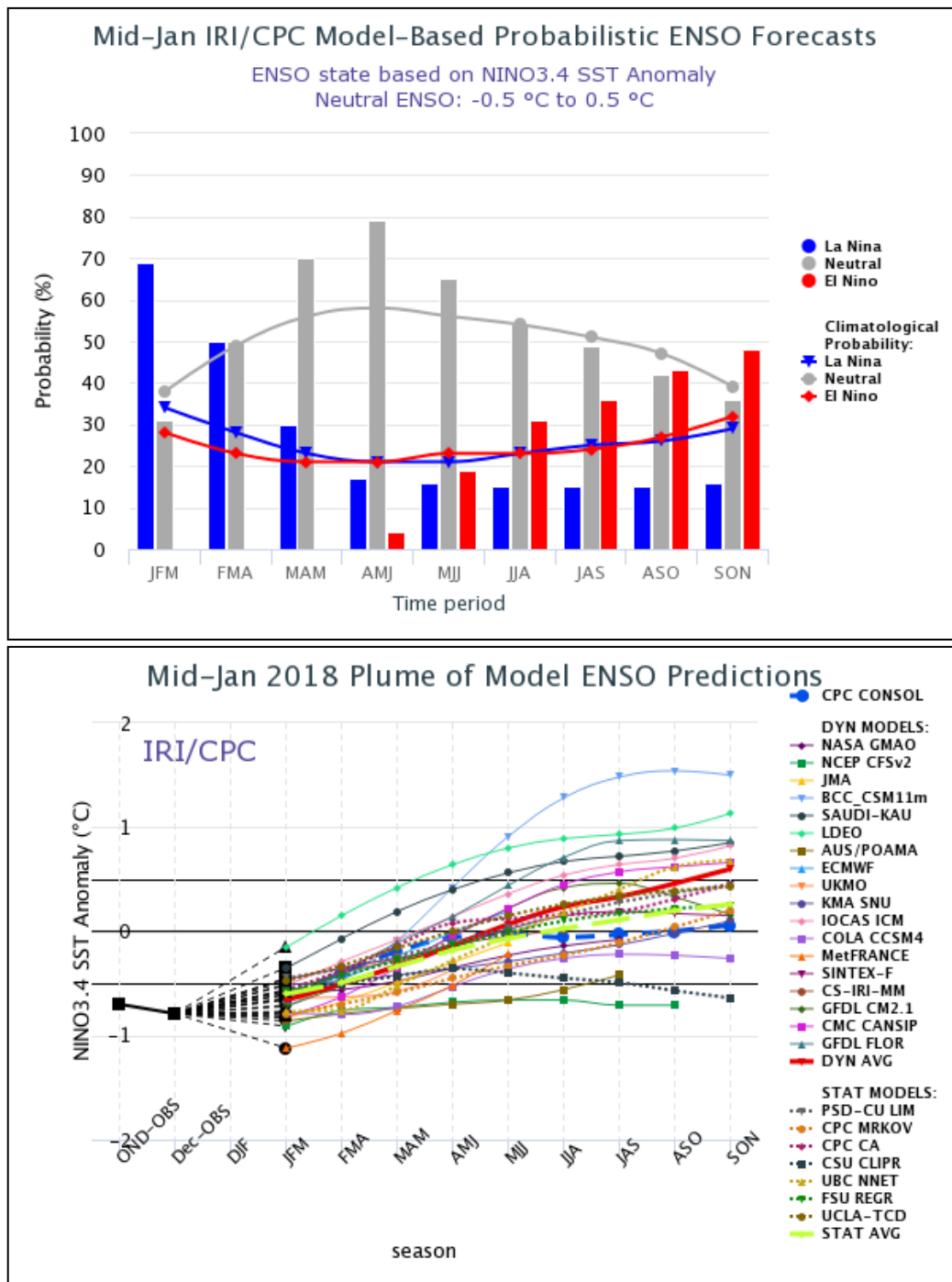
Figura 15. Predicción modelos estadísticos y dinámicos de condiciones ENOS 19 de enero del 2018. (Fuente: IRI/CPC).
