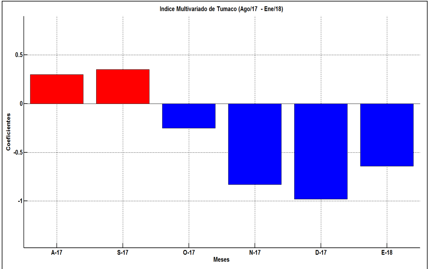
Figura 14. Comportamiento del Índice Multivariado de Tumaco (IMT) para el periodo comprendido entre agosto del 2017 y enero del 2018. Fuente: CCCP.
