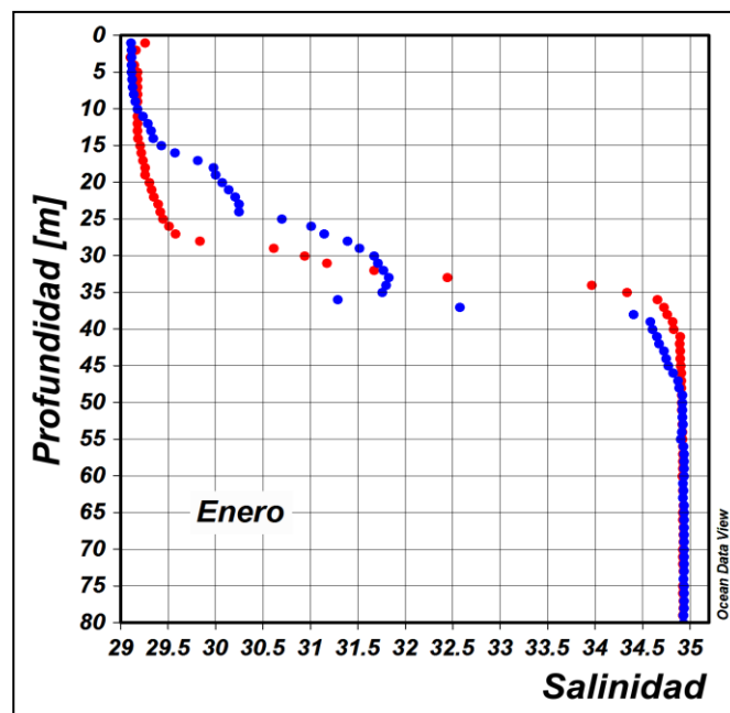
Figura 13. Perfil de salinidad para el mes de enero del 2018 en la estación costera fija de Tumaco. En color rojo se presenta el perfil obtenido en la primera quincena del mes y en azul el realizado a finales del mismo. Fuente: CCCP.
