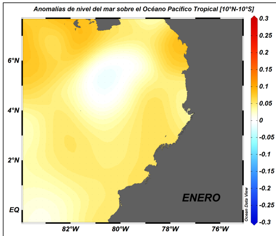
Figura 6. Anomalías de nivel del mar CPC, enero del 2018 (Fuente: Copernicus Marine Service (CMEMS), Procesamiento: CIOHP).
