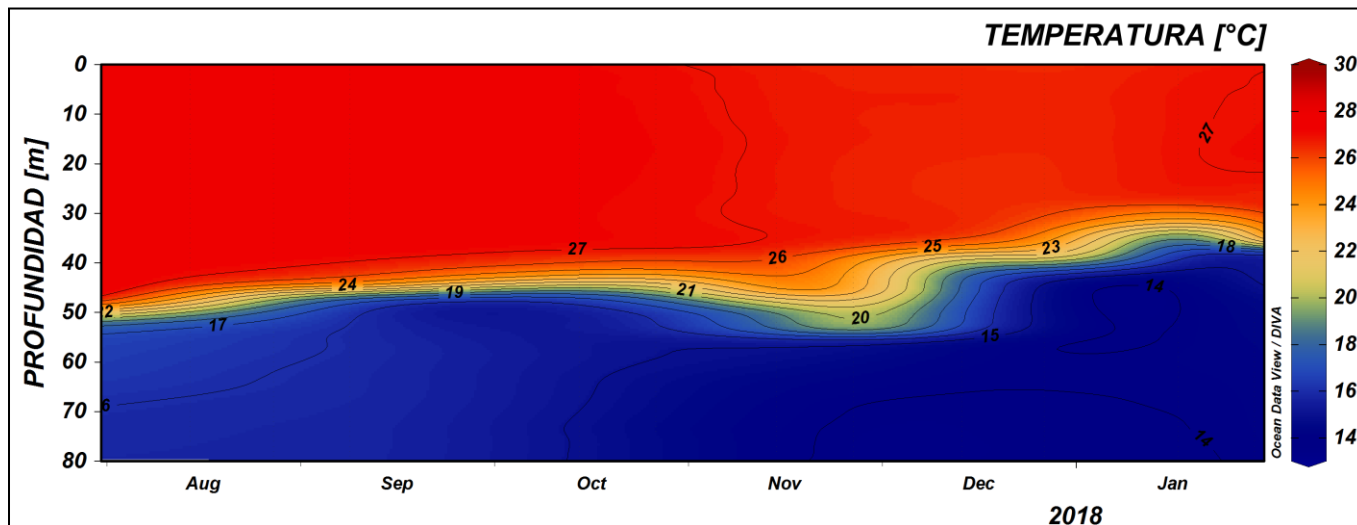
Figura 10. Serie temporal de temperatura del agua en la estación costera fija de Tumaco entre 0 a 80 metros de profundidad, para el periodo de comprendido entre agosto del 2017 y enero del 2018. La escala de colores representa la magnitud de la temperatura medida en °C. Fuente: CCCP.
