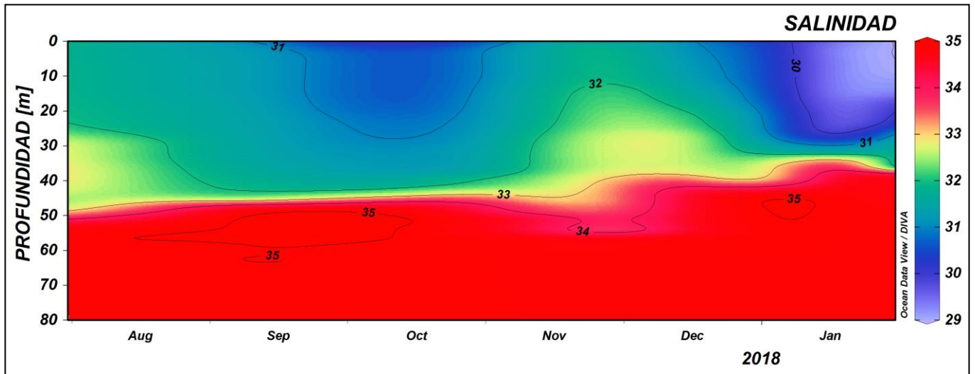
Figura 12. Serie temporal de salinidad del agua en la estación costera fija de Tumaco entre 0 a 80 metros de profundidad, para el periodo de comprendido entre agosto del 2017 y enero del 2018. Fuente: CCCP.
