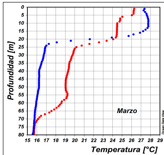
Figura 12. Perfil de temperatura para el mes de marzo del 2018 registrado en la estación costera fija de Tumaco. En color rojo se presenta el perfil obtenido en la primera quincena del mes y en azul el realizado a finales del mismo. Fuente: CCCP.
