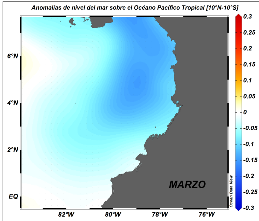
Figura 6. Anomalías de nivel del mar CPC, marzo del 2018 (Fuente: Copernicus Marine Service (CMEMS), Procesamiento: CIOHP).
