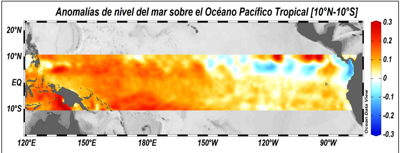
Figura 5. Anomalías de nivel del mar Océano Pacífico Tropical para el mes de marzo del 2018. La escala de colores representa la magnitud media en metros (m) (Fuente: Copernicus Marine Service (CMEMS), Procesamiento: CIOHP).
