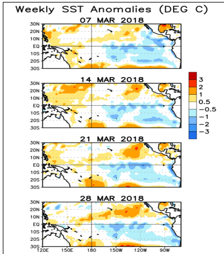
Figura 3. Anomalías semanales de TSM en el Océano Pacífico Tropical para el periodo comprendido entre el 07 y el 28 de marzo del 2018. Fuente: Climate Prediction Center-NOAA.
