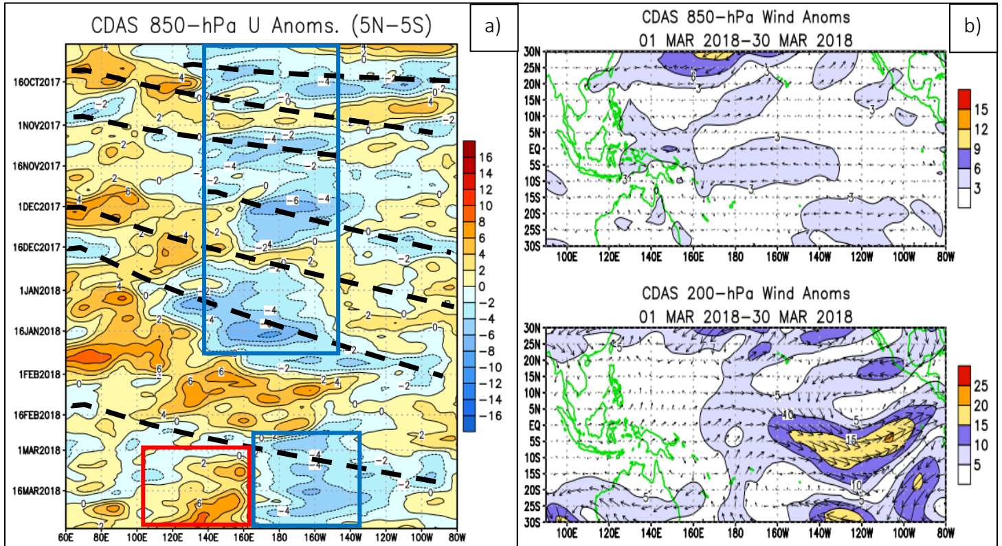
Figura 7. Anomalías campos de vientos sobre el Océano Pacífico Ecuatorial (OPE) para el periodo comprendido entre el 01 y el 30 de marzo del 2018. Fuente: Climate Prediction Center-NOAA.
