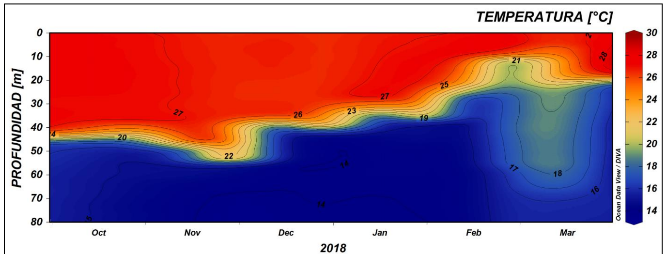
Figura 11. Serie temporal de temperatura del agua en la estación costera fija de Tumaco entre 0 a 80 metros de profundidad, para el periodo comprendido entre octubre del 2017 y marzo del 2018. La escala de colores representa la magnitud de la temperatura medida en °C. Fuente: CCCP.
