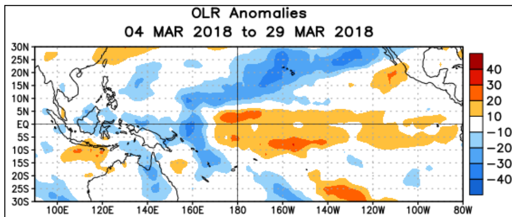
Figura 8. Anomalías Radiación de Onda Larga (OLR, por sus siglas en inglés) Para el periodo comprendido entre el 04 y el 29 de marzo del 2018. La escala de colores representa en W/m^2 . Fuente: Climate Prediction Center-NOAA.
