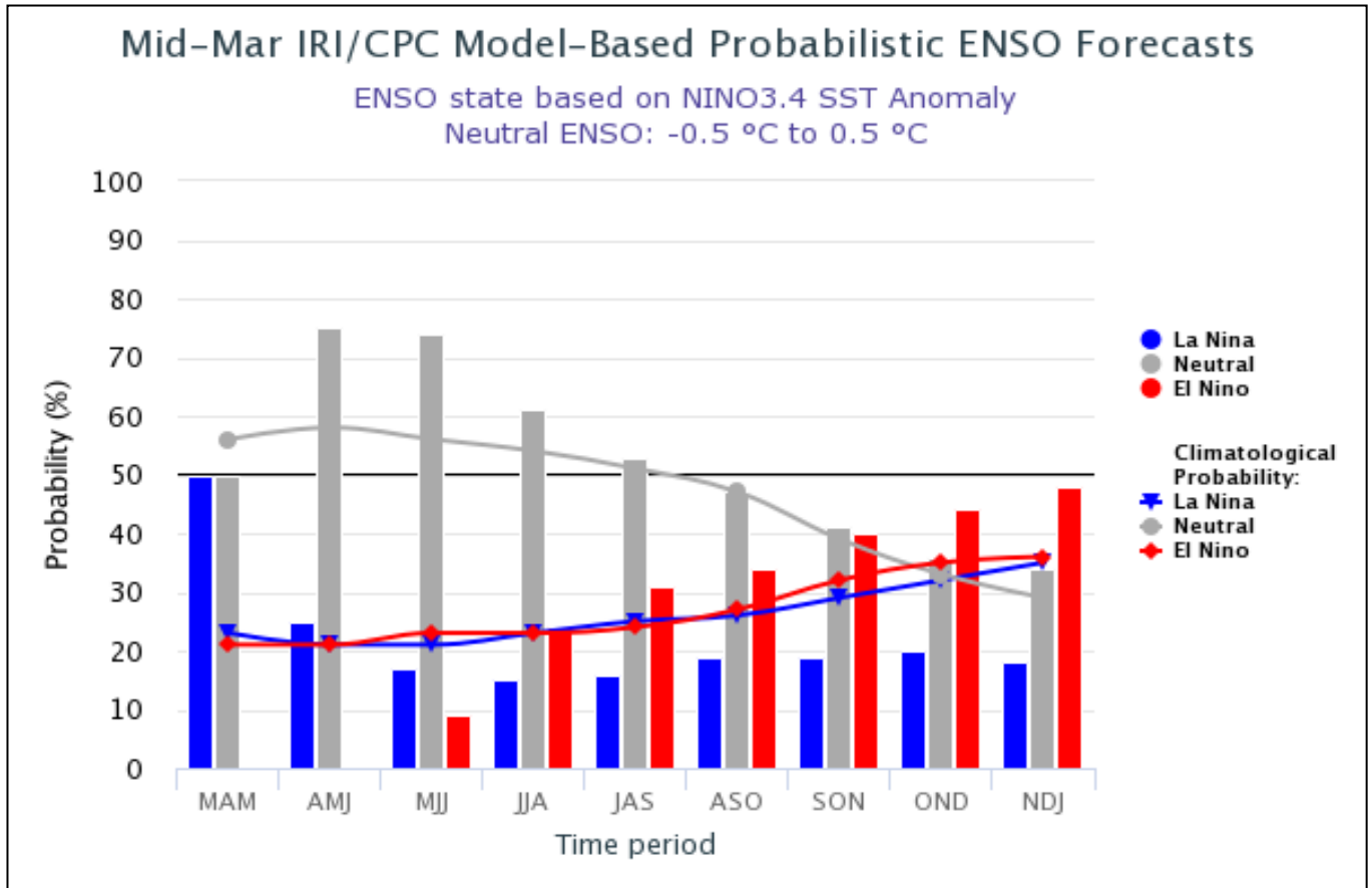
Figura 16. Predicción modelos estadísticos y dinámicos de condiciones ENOS 19 de marzo del 2018. (Fuente: IRI/CPC).
