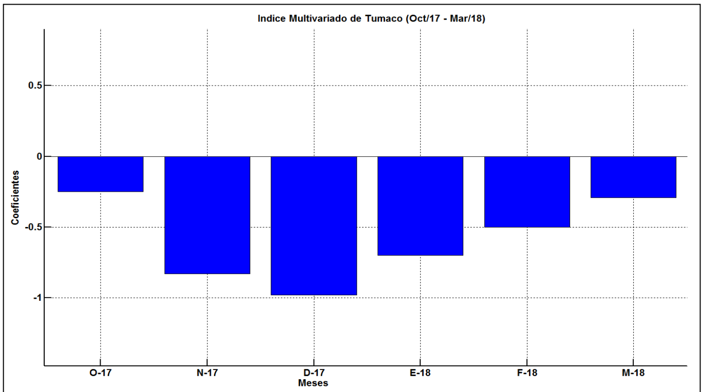
Figura 15. Comportamiento del Índice Multivariado de Tumaco (IMT) para el periodo comprendido entre octubre del 2017 y marzo del 2018. Fuente: CCCP.
