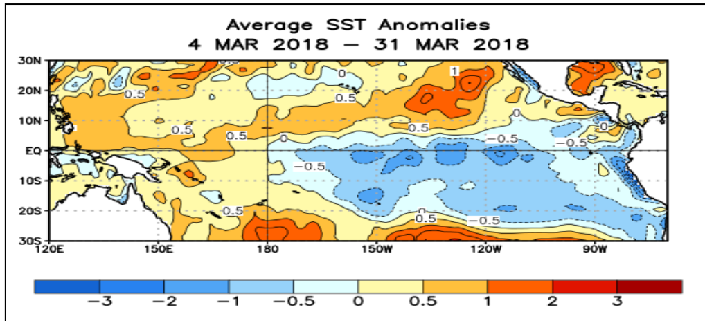
Figura 2. Anomalías de TSM en el Océano Pacífico Tropical para el periodo comprendido entre el 04 y el 31 de marzo del 2018. La escala de colores representa la magnitud en ^{\circ}\text{C} . Fuente: Climate Prediction Center – NOAA.
