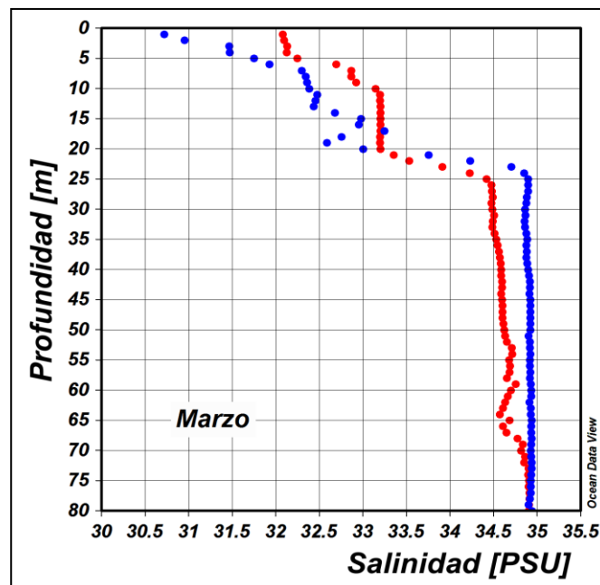
Figura 14. Perfil de salinidad para el mes de marzo del 2018 en la estación costera fija de Tumaco. En color rojo se presenta el perfil obtenido en la primera quincena del mes y en azul el realizado a finales del mismo. Fuente: CCCP.
