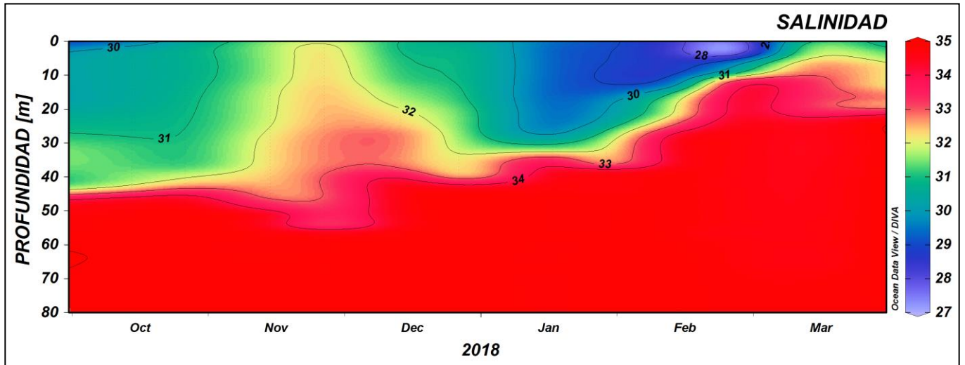
Figura 13. Serie temporal de salinidad del agua en la estación costera fija de Tumaco entre 0 a 80 metros de profundidad, para el periodo de comprendido entre octubre del 2017 y marzo del 2018. Fuente: CCCP.
