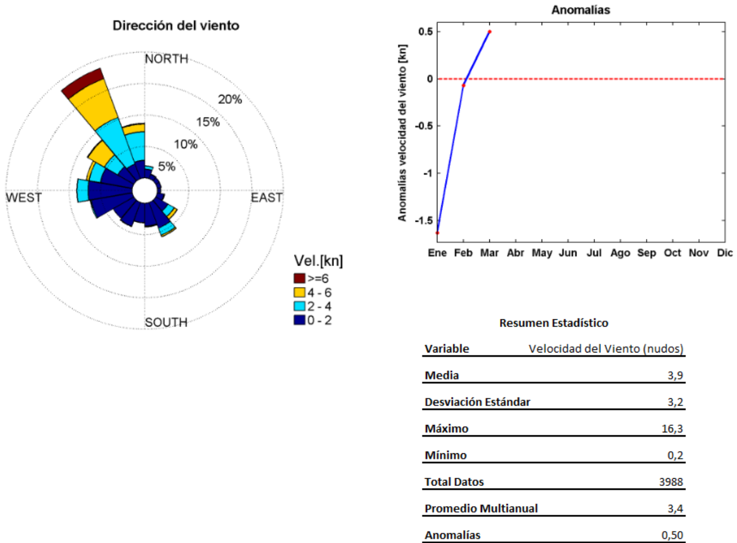
Figura 5. Distribución de frecuencia de la dirección, velocidad, anomalía velocidad y resumen estadístico del viento en Bahía Solano.
