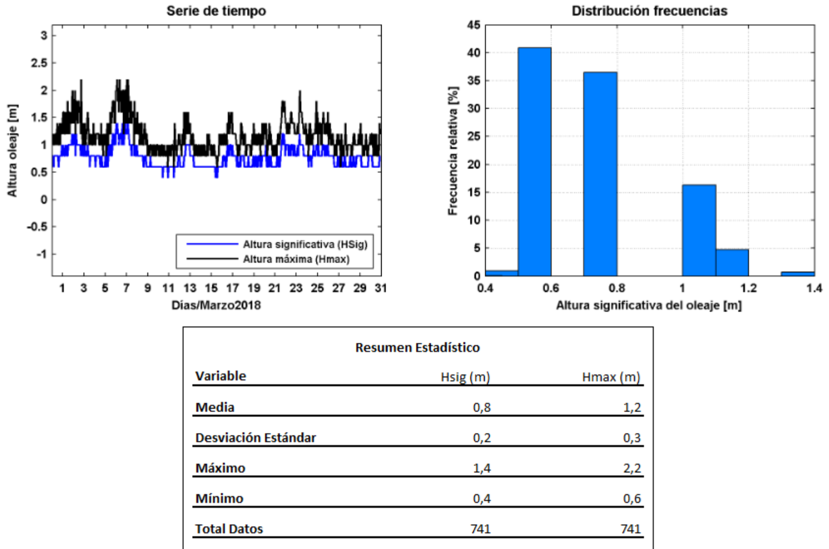
Figura 20. Serie de tiempo, histograma de frecuencia y resumen estadístico mensual de la altura significativa y máxima del oleaje, Bahía Solano.
