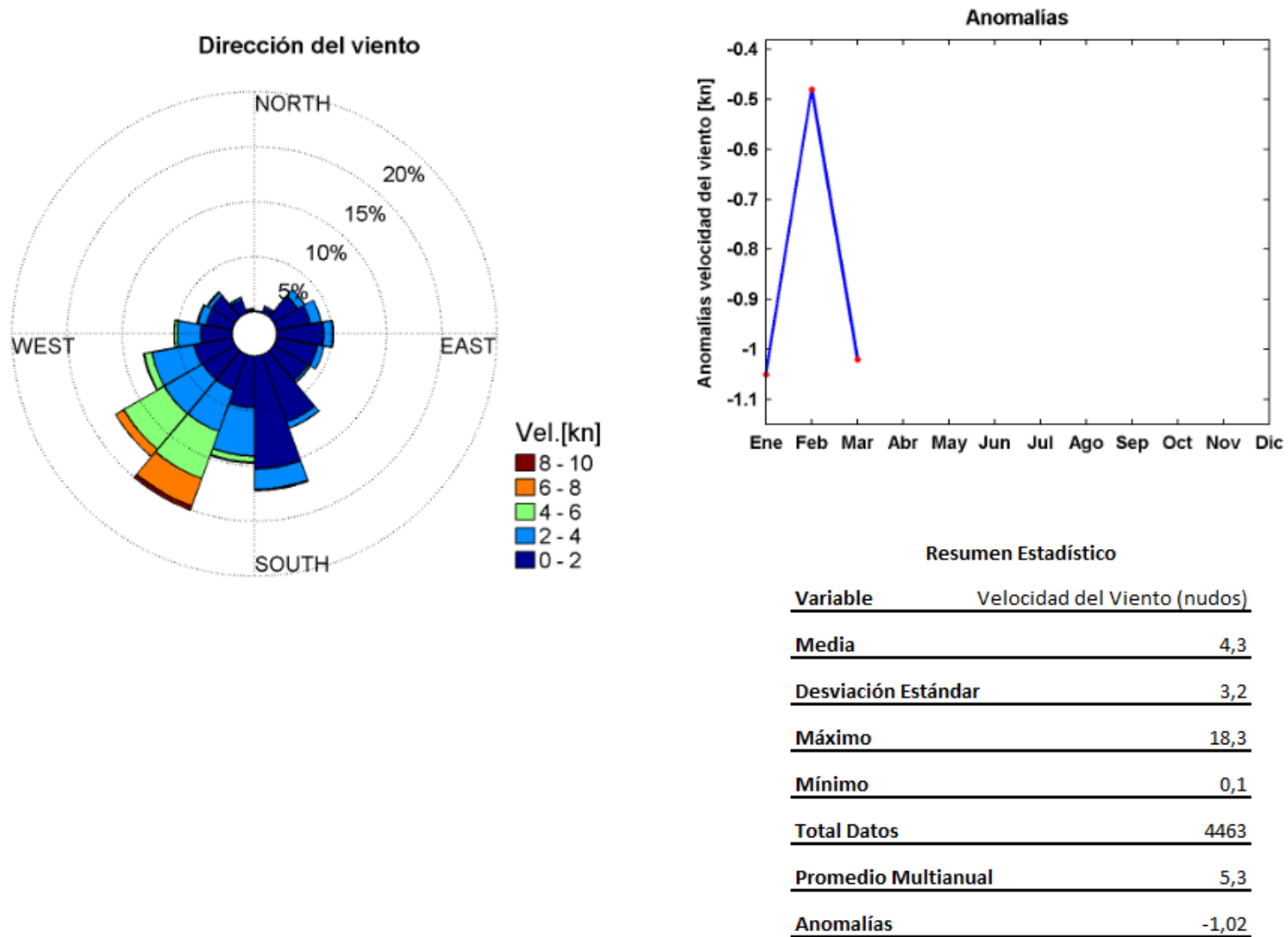
Figura 11. Distribución de frecuencia de la dirección, velocidad, anomalía velocidad y resumen estadístico del viento en Buenaventura.
