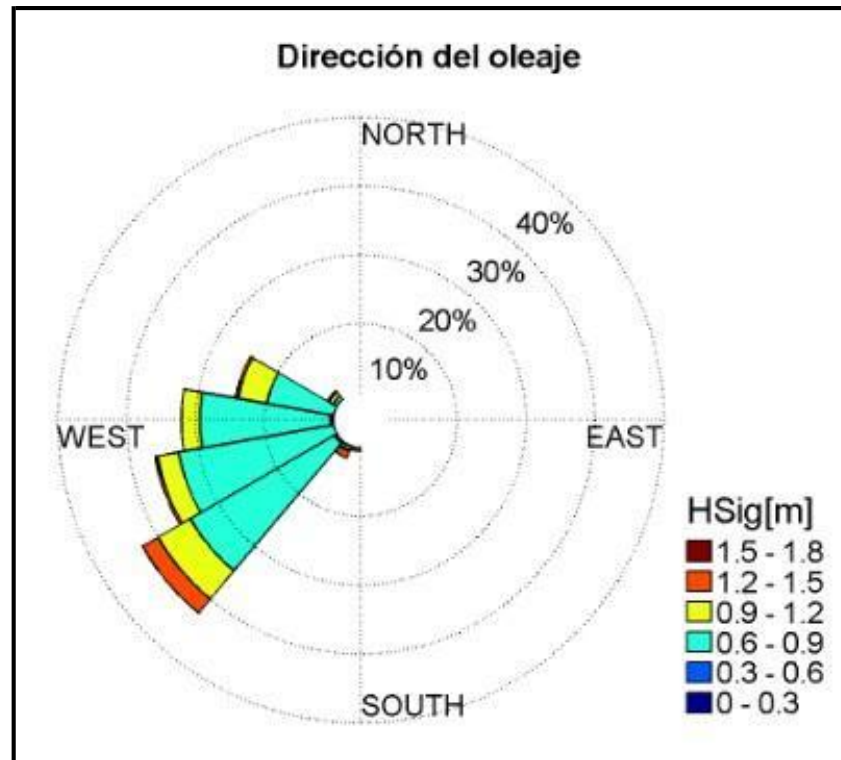
Figura 19. Distribución de frecuencia de la dirección del oleaje, Bahía Solano.
