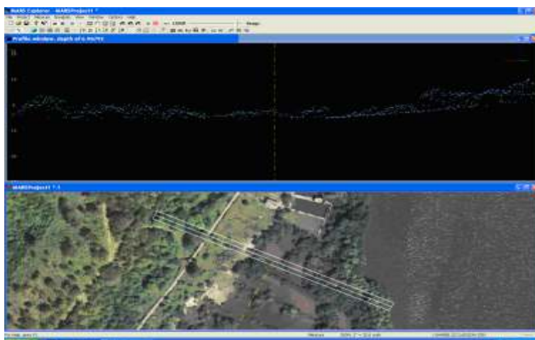
Figura 12. Perfil N° 2, del área de estudio. Sector Media Tapa, Cartagena- Colombia.
