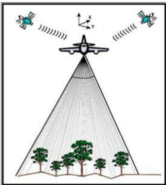
Figura 2. Modo de Operación del sensor LIDAR a bordo de una plataforma, aerotransportada.
