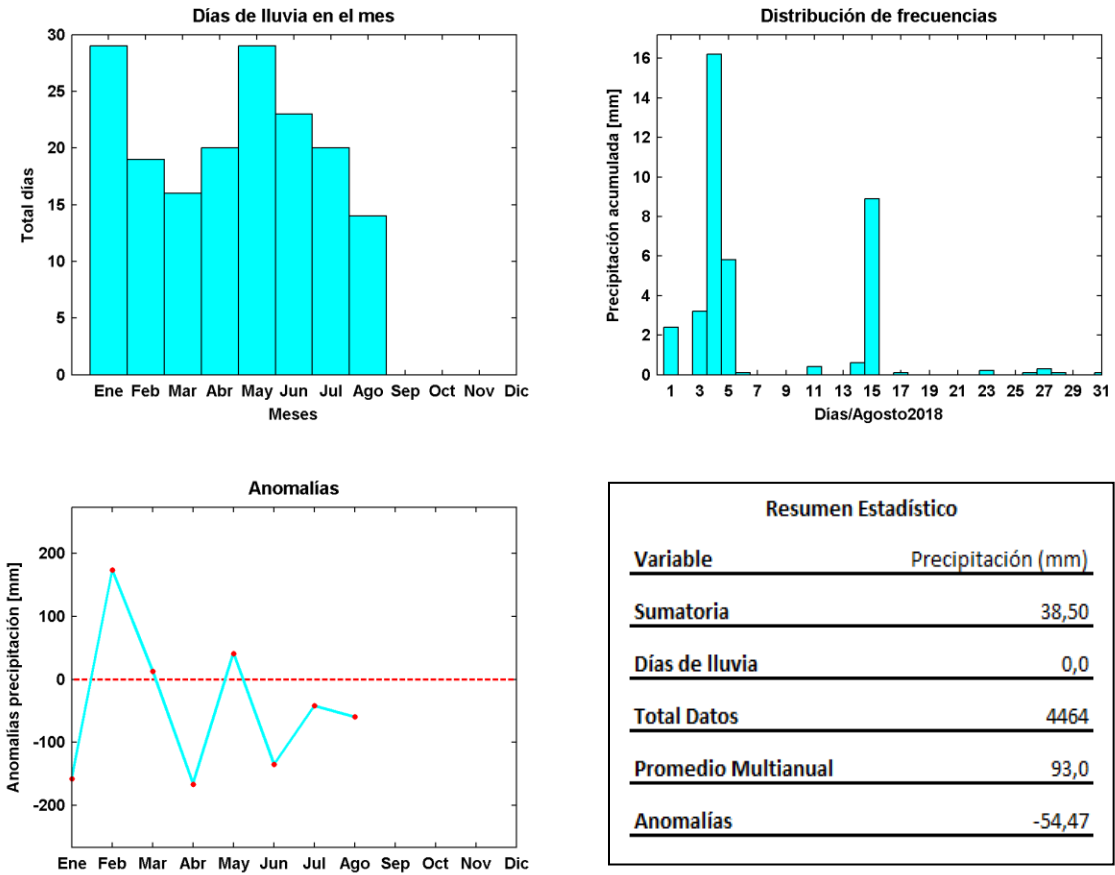
Figura 17. Días de lluvia, sumatoria precipitación acumulada, anomalía y resumen estadístico mensual de la precipitación en Tumaco
