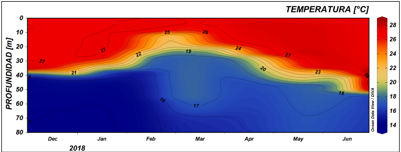
Figura 11. Serie temporal de temperatura del agua en la estación costera fija de Tumaco entre 0 a 80 metros de profundidad, para el periodo de comprendido entre diciembre del 2017 y junio del 2018. La escala de colores representa la magnitud de la temperatura medida en °C. Fuente: CCCP.
