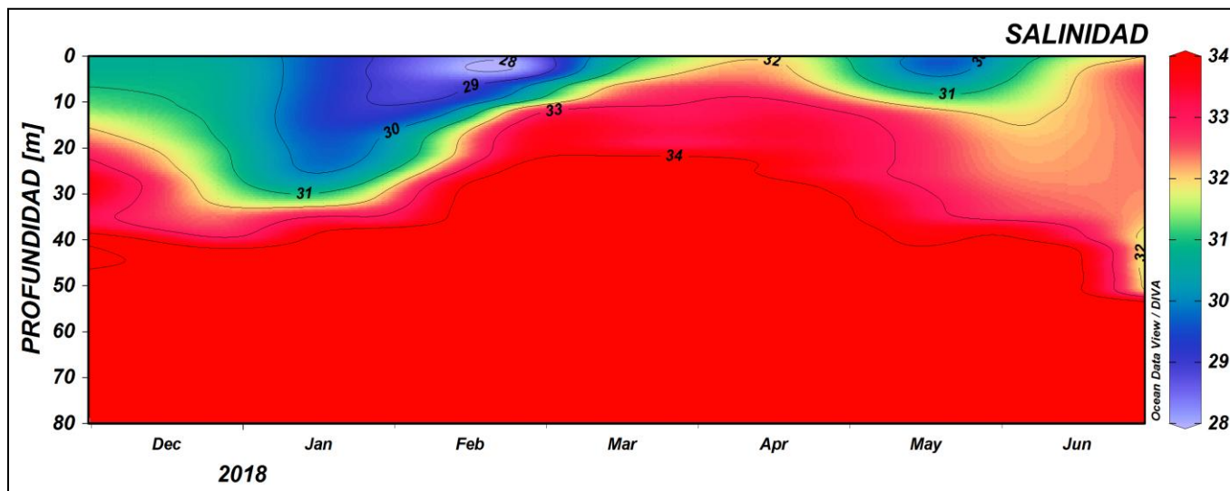
Figura 13. Serie temporal de salinidad del agua en la estación costera fija de Tumaco entre 0 a 80 metros de profundidad, para el periodo de comprendido entre diciembre del 2017 y junio del 2018. Fuente: CCCP.
