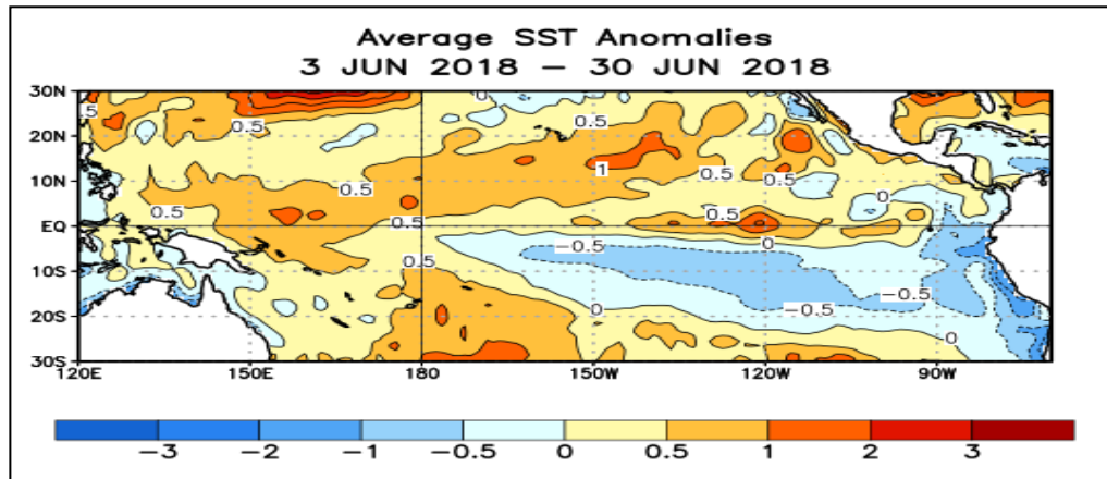
Figura 2. Anomalías de TSM en el Océano Pacífico Tropical para el periodo comprendido entre el 03 de junio y el 30 de junio del 2018. La escala de colores representa la magnitud en °C. Fuente: Climate Prediction Center – NOAA.
