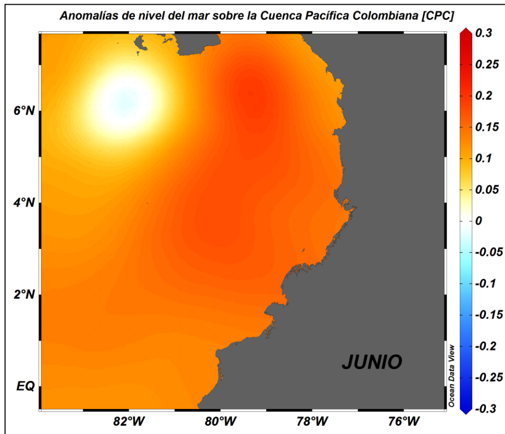
Figura 6. Anomalías de nivel del mar CPC, junio del 2018 (Fuente: Copernicus Marine Service (CMEMS), Procesamiento: CIOHP).
