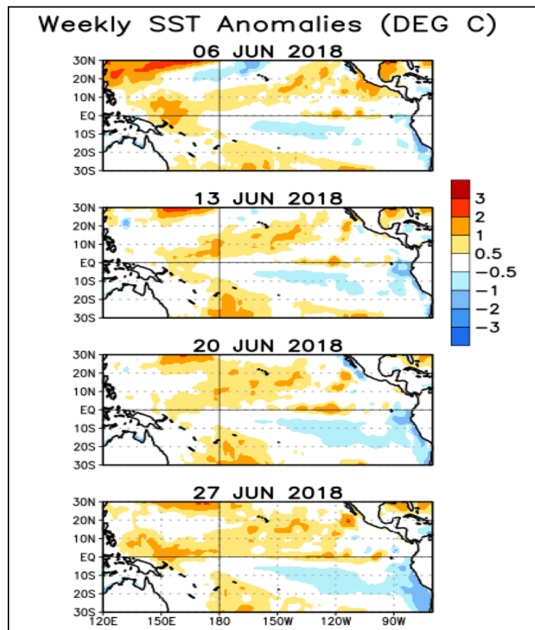
Figura 3. Anomalías semanales de TSM en el Océano Pacífico Tropical para el periodo comprendido entre el 06 y el 30 de junio del 2018. Fuente: Climate Prediction Center-NOAA.
