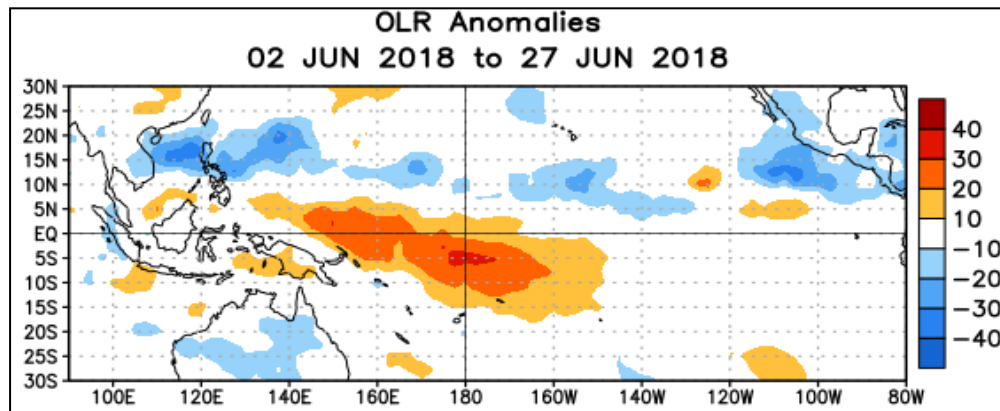
Figura 8. Anomalías Radiación de Onda Larga (OLR, por sus siglas en inglés) Para el periodo comprendido entre el 02 y el 27 de junio del 2018. La escala de colores representa en W/m 2 . Fuente: Climate Prediction Center-NOAA.
