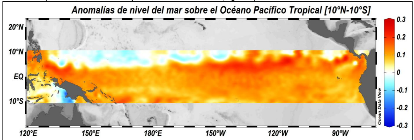
Figura 5. Anomalías de nivel del mar Océano Pacífico Tropical para el mes de junio del 2018. La escala de colores representa la magnitud media en metros (m) (Fuente: Copernicus Marine Service (CMEMS), Procesamiento: CIOHP).
