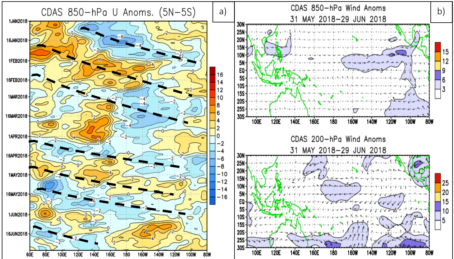
Figura 7. Anomalías campos de vientos sobre el Océano Pacífico Ecuatorial (OPE) para el periodo comprendido entre el 31 de mayo y el 29 de junio del 2018. Fuente: Climate Prediction Center-NOAA.
