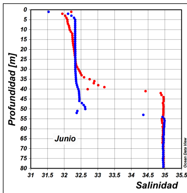
Figura 14. Perfil de salinidad para el mes de junio del 2018 en la estación costera fija de Tumaco. En color rojo se presenta el perfil obtenido en la primera quincena del mes y en azul el realizado a finales del mismo. Fuente: CCCP.
