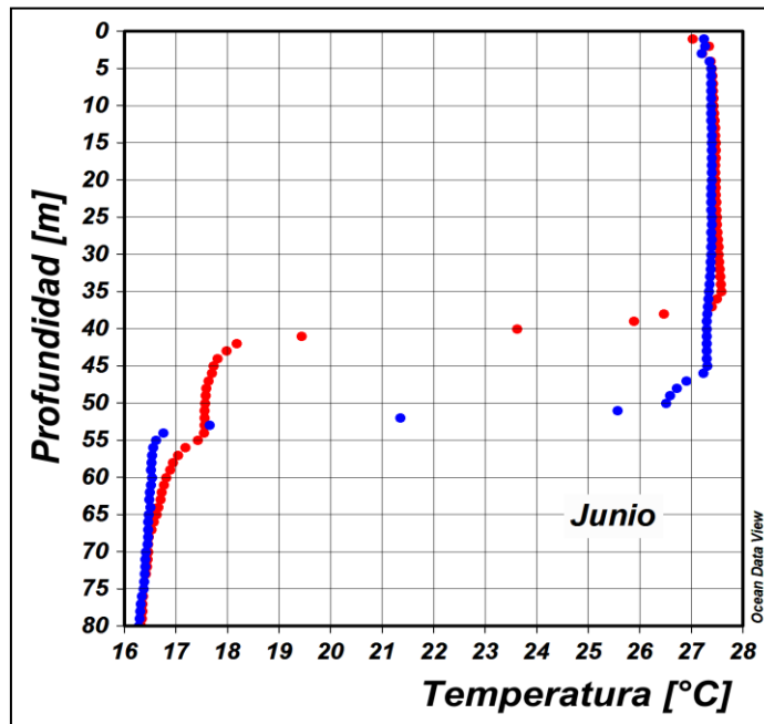
Figura 12. Perfil de temperatura para el mes de junio del 2018 registrado en la estación costera fija de Tumaco. En color rojo se presenta el perfil obtenido en la primera quincena del mes y en azul el realizado a finales del mismo. Fuente: CCCP.
