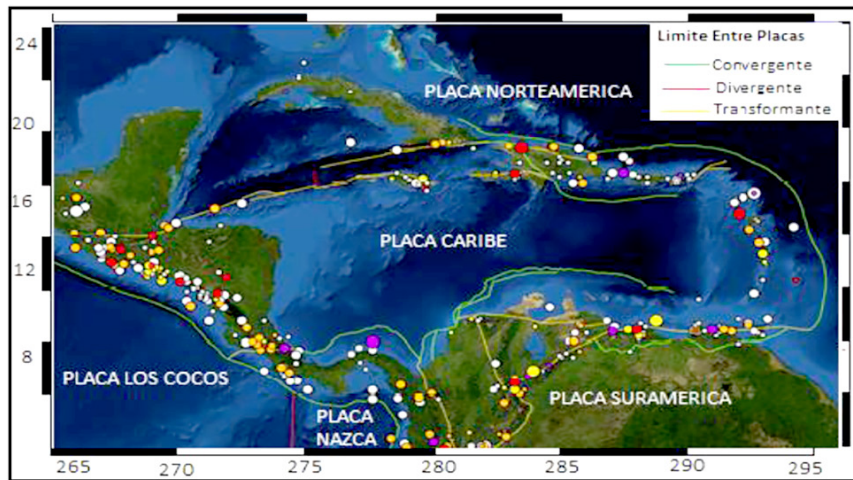
Figura 3. Tsunamis en el mar Caribe con línea de frontera entre placas (NOAA, 2015). Todos los sismos en el mar Caribe de los catálogos National Oceanic and Atmospheric Administration (NOAA), The Global Centroid-Moment-Tensor (CMT) e Incorporated Research Institutions for Seismology (IRIS).
