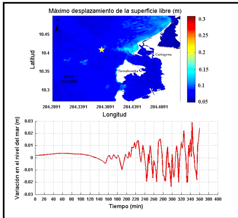
Figura 12. Resultado de escenario generador de tsunami de origen regional ubicado en Swan, con magnitud Mw 7.3 para la población de Cartagena.
