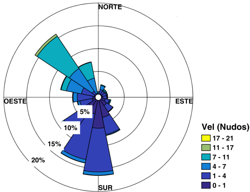
Figura 20. Distribución del régimen de viento en Coveñas.
