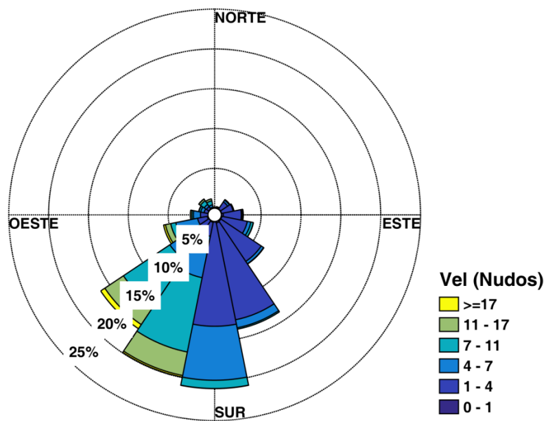
Figura 23. Distribución del régimen de viento en Turbo.
