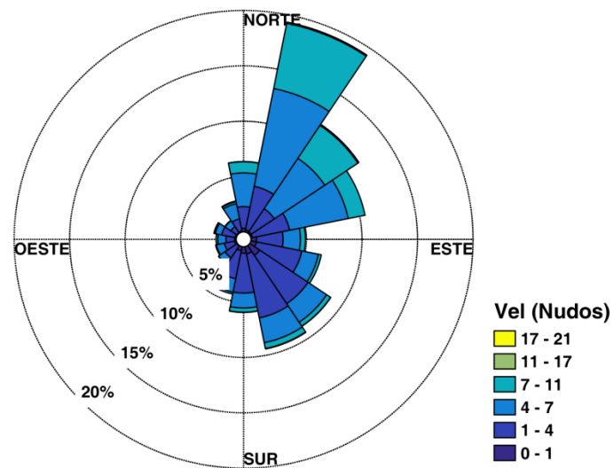
Figura 4. Distribución del régimen de viento en Providencia.
