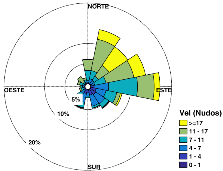
Figura 8. Distribución del régimen de viento en Ballenas.
