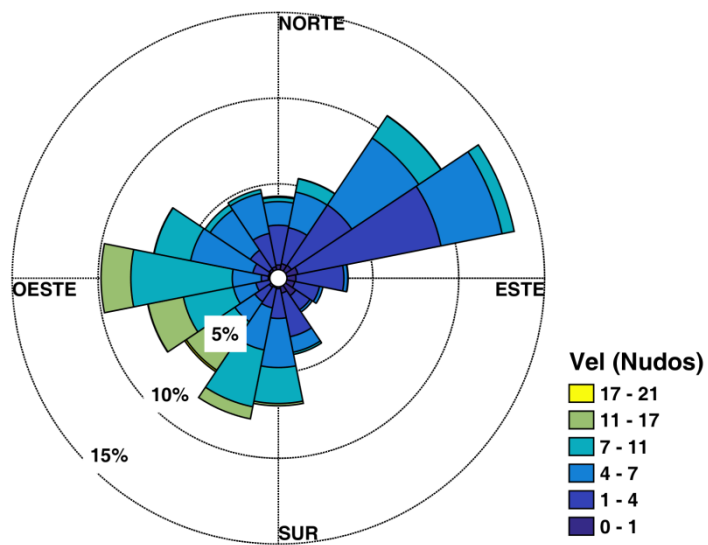
Figura 16. Distribución del régimen de viento en Cartagena.
