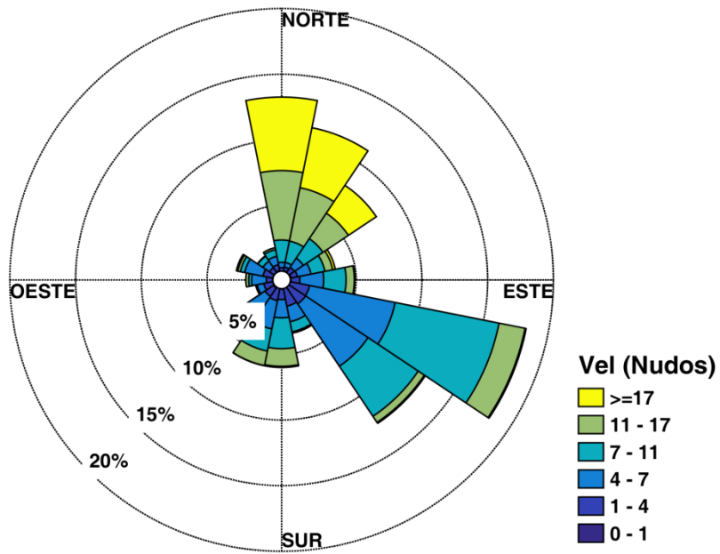
Figura 14. Distribución del régimen de viento en Santa Marta.
