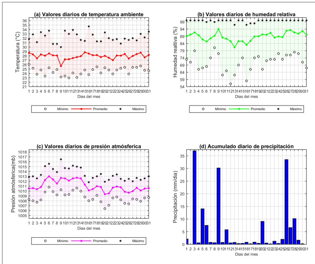
Figura 19. Comportamiento mensual de la presión atmosférica, temperatura del aire, acumulado de precipitación y humedad relativa en Coveñas.
