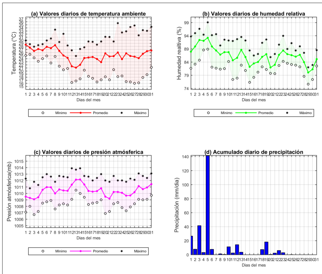
Figura 9. Comportamiento mensual de la presión atmosférica, temperatura del aire, acumulado de precipitación y humedad relativa en Puerto Estrella.
