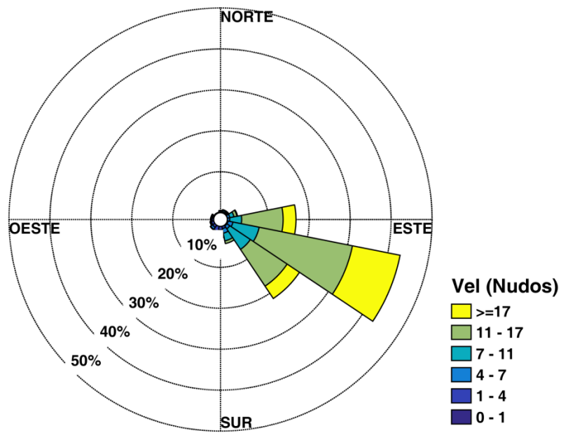
Figura 10. Distribución del régimen de viento en Puerto Estrella.
