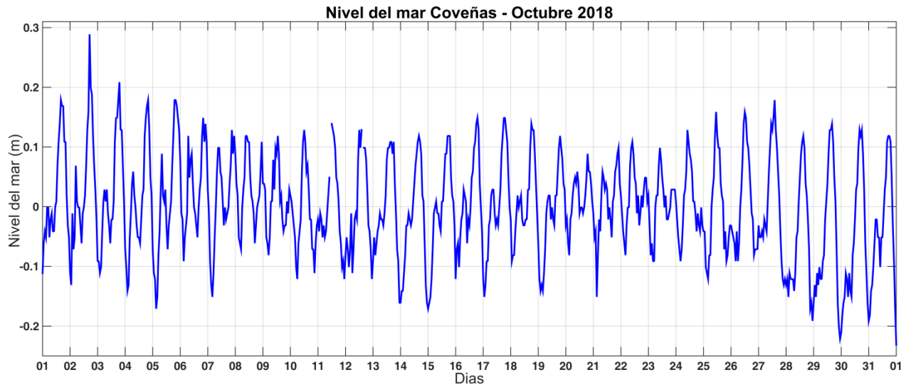
Figura 21. Comportamiento del nivel del mar en Coveñas.
