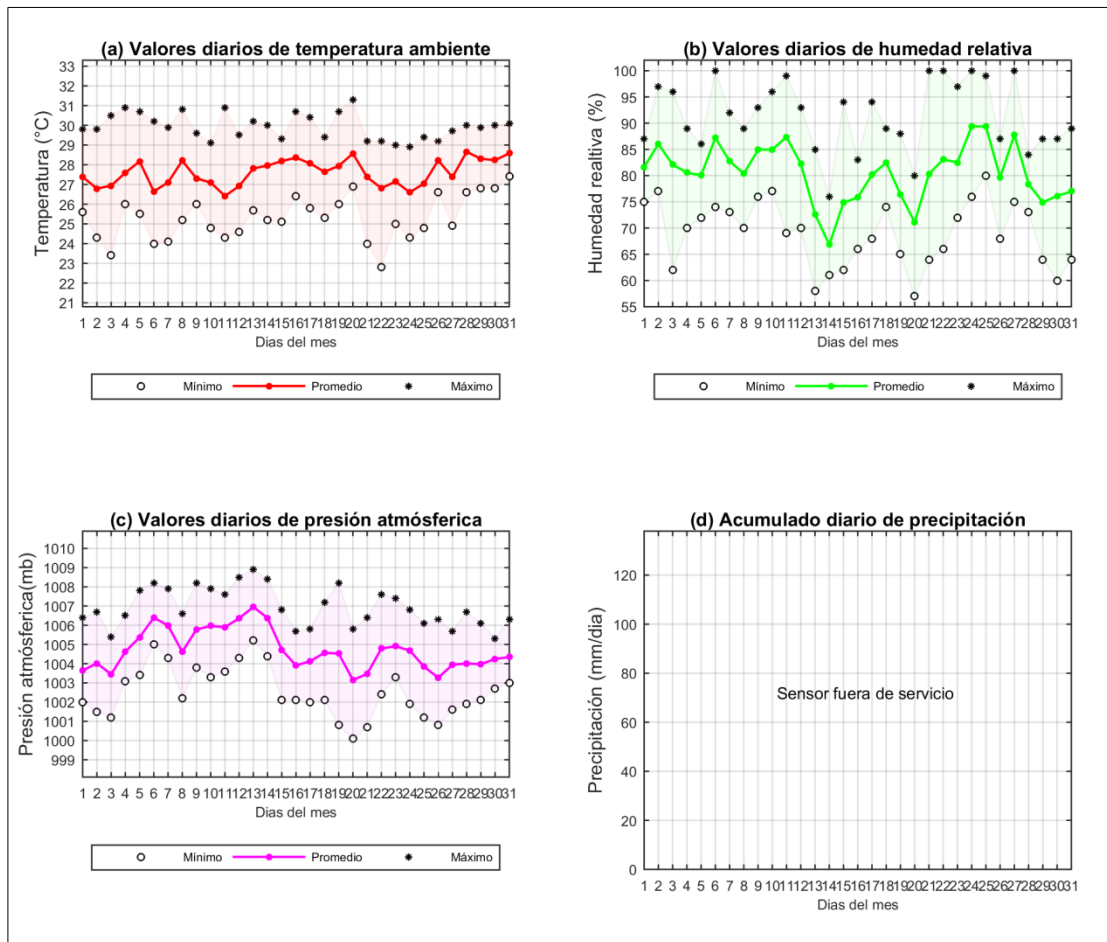
Figura 13. Comportamiento mensual de la presión atmosférica, temperatura del aire, acumulado de precipitación y humedad relativa en Santa Marta.
