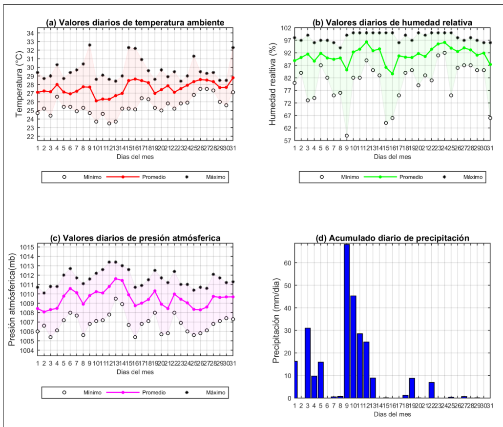
Figura 7. Comportamiento mensual de la presión atmosférica, temperatura del aire, acumulado de precipitación y humedad relativa en Ballenas.
