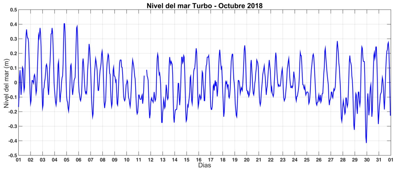
Figura 24. Comportamiento del nivel del mar en Turbo.
