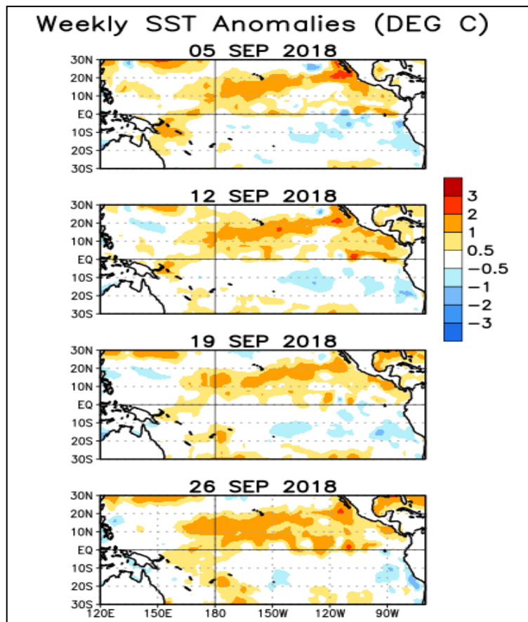
Figura 3. Anomalías semanales de TSM en el Océano Pacífico Tropical para el periodo comprendido entre el 05 y el 26 de Septiembre del 2018. Fuente: Climate Prediction Center-NOAA.
