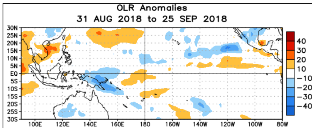
Figura 8. Anomalías Radiación de Onda Larga (OLR, por sus siglas en inglés) Para el periodo comprendido entre el 31 de agosto y el 25 de Septiembre del 2018. La escala de colores representa en W/m^2 . Fuente: Climate Prediction Center-NOAA.
