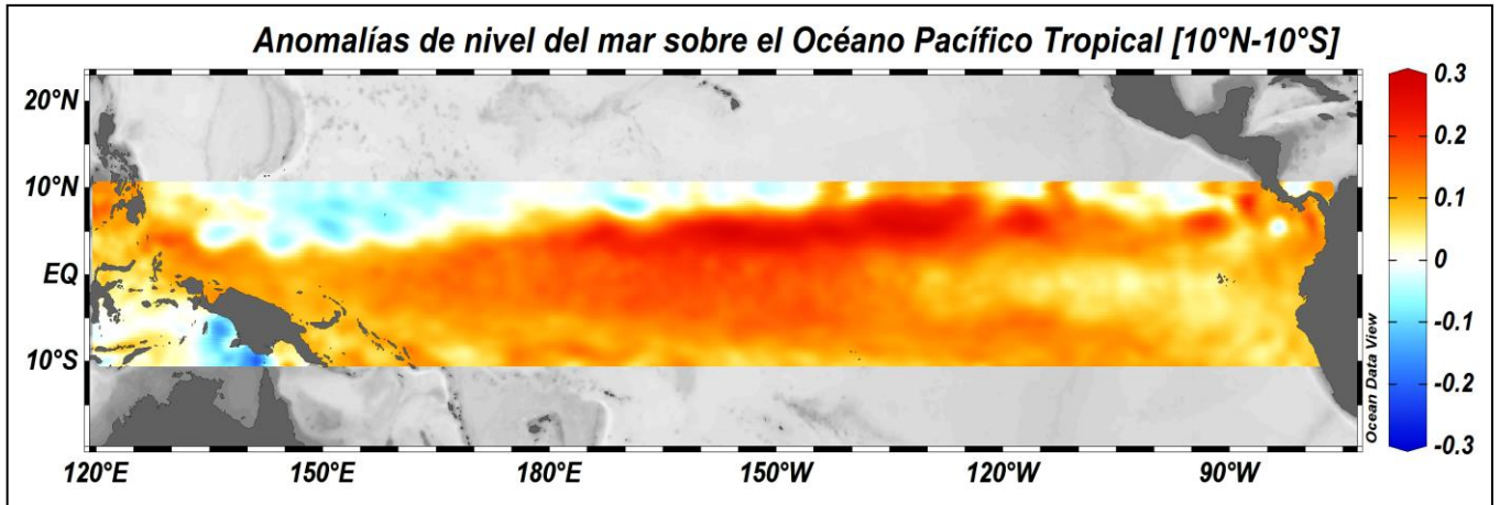
Figura 5. Anomalías de nivel del mar Océano Pacífico Tropical para el mes de Septiembre del 2018. La escala de colores representa la magnitud media en metros (m) (Fuente: Copernicus Marine Service (CMEMS), Procesamiento: CIOHP).
