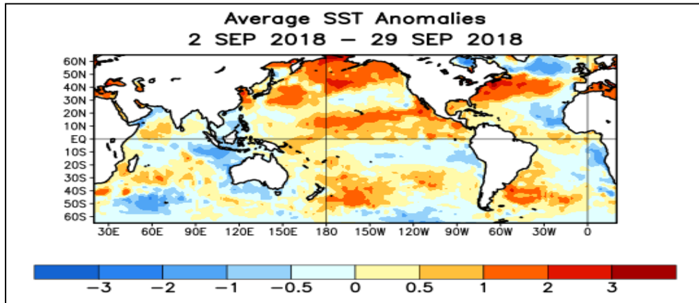
Figura 2. Anomalías de TSM en el Océano Pacífico Tropical para el periodo comprendido entre el 02 de Septiembre y el 29 de septiembre del 2018. La escala de colores representa la magnitud en °C. Fuente: Climate Prediction Center – NOAA.
