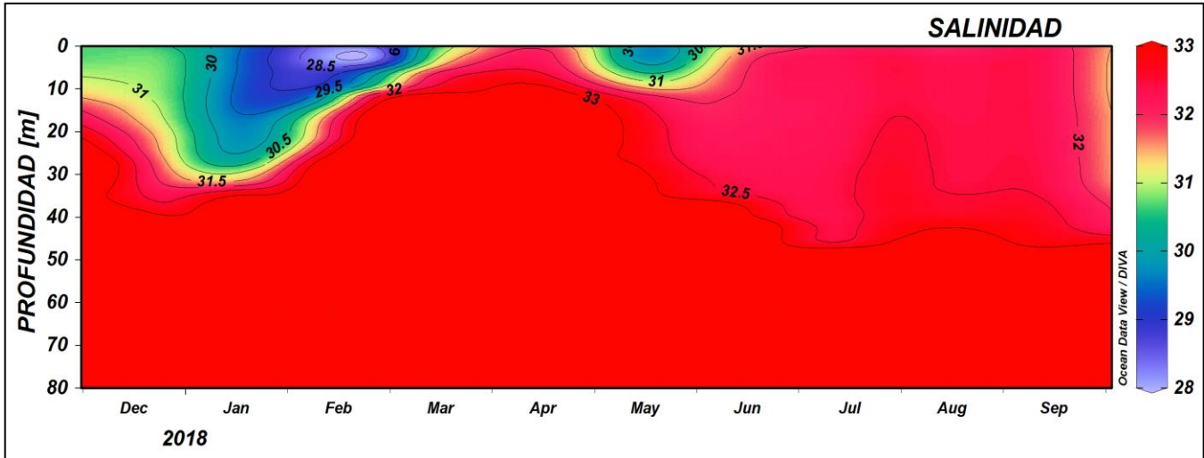
Figura 13. Serie temporal de salinidad del agua en la estación costera fija de Tumaco entre 0 a 80 metros de profundidad, para el periodo de comprendido entre diciembre del 2017 y Septiembre del 2018. Fuente: CCCP.
