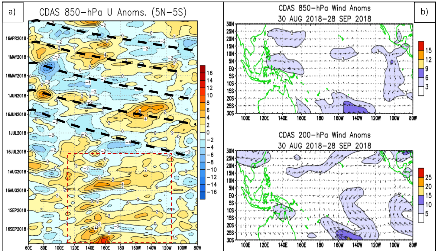
Figura 7. Anomalías campos de vientos sobre el Océano Pacífico Ecuatorial (OPE) para el periodo comprendido entre el 30 de agosto al 28 Septiembre del 2018. Fuente: Climate Prediction Center-NOAA.
