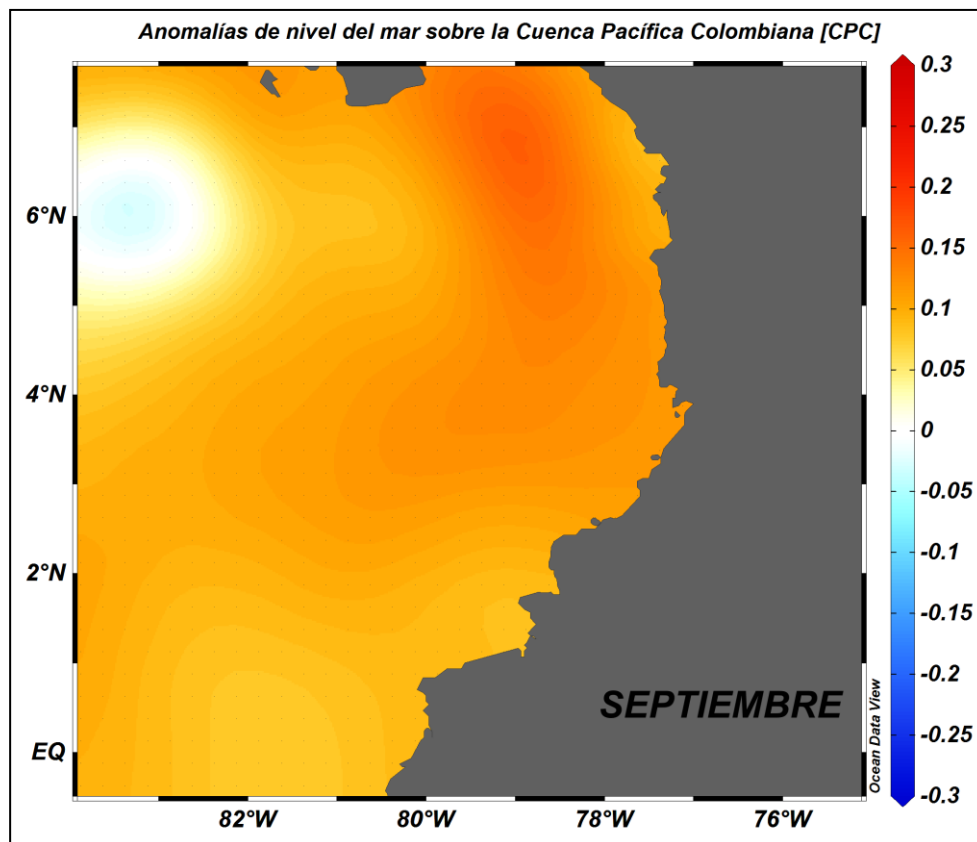
Figura 6. Anomalías de nivel del mar CPC, Septiembre del 2018 (Fuente: Copernicus Marine Service (CMEMS), Procesamiento: CIOHP).
