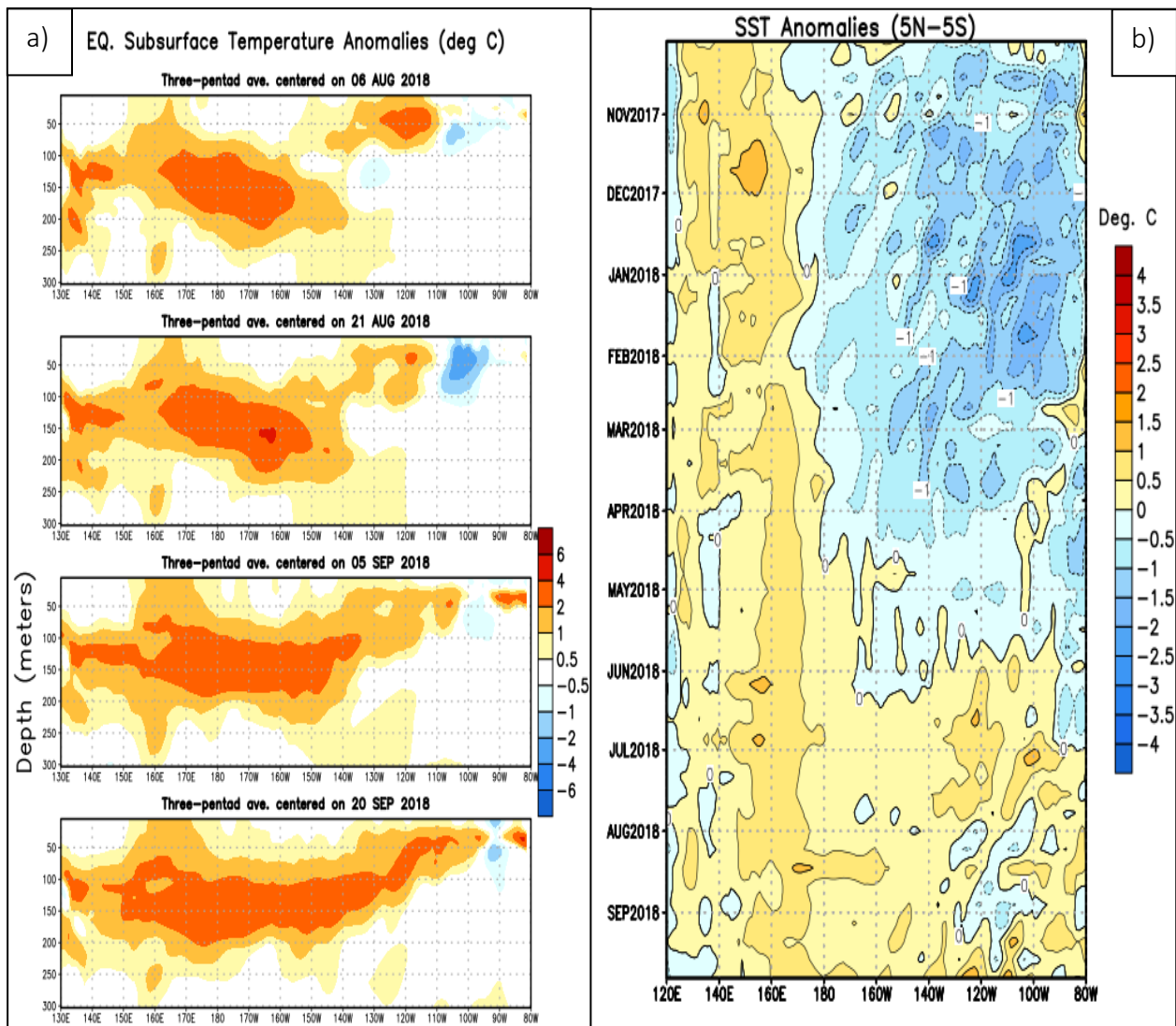
Figura 1. Evolución de las anomalías de temperatura subsuperficial (a) en el Océano Pacífico Ecuatorial (OPE) y superficiales (b) entre latitudes 5°S y 5°N para el periodo comprendido entre el 06 de agosto y el 20 de Septiembre del 2018. La escala de colores representa la magnitud de las anomalías en °C. Fuente: Climate Prediction Center-NOAA.
