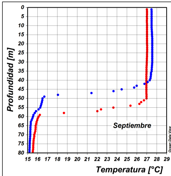
Figura 12. Perfil de temperatura para el mes de Septiembre del 2018 registrado en la estación costera fija de Tumaco. En color rojo se presenta el perfil obtenido en la primera quincena del mes y en azul el realizado a finales del mismo. Fuente: CCCP.
