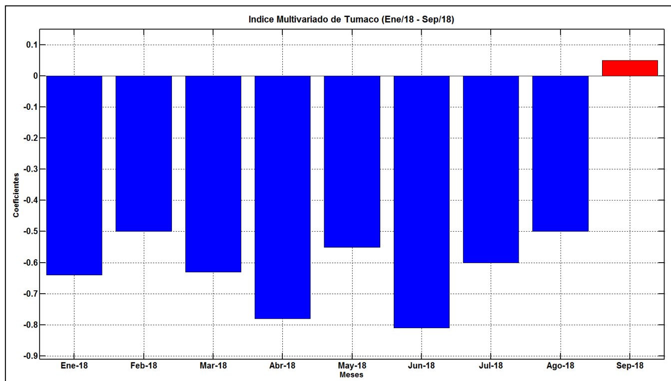
Figura 15. Comportamiento del Índice Multivariado de Tumaco (IMT) para el periodo comprendido entre enero y Septiembre del 2018. Fuente: CCCP.
