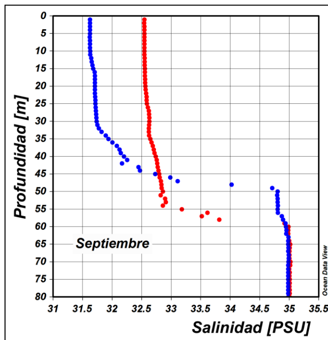
Figura 14. Perfil de salinidad para el mes de Septiembre del 2018 en la estación costera fija de Tumaco. En color rojo se presenta el perfil obtenido en la primera quincena del mes y en azul el realizado a finales del mismo. Fuente: CCCP.
