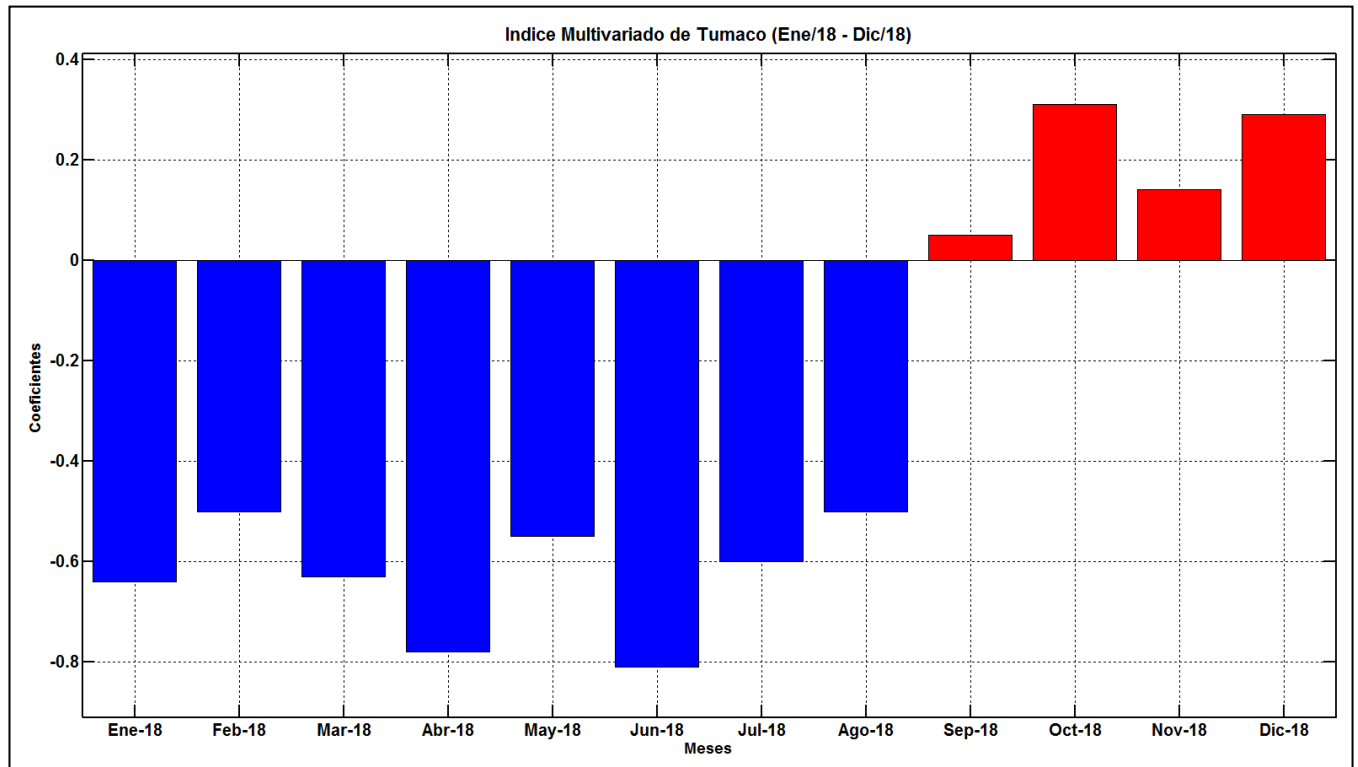
Figura 15. Comportamiento del Índice Multivariado de Tumaco (IMT) para el periodo comprendido entre enero y Diciembre del 2018. Fuente: CCCP.
