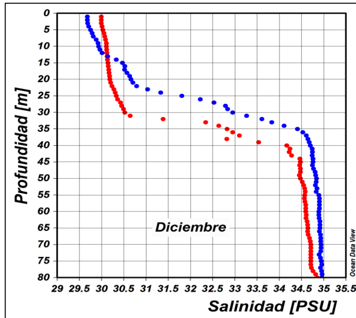
Figura 14. Perfil de salinidad para el mes de Diciembre del 2018 en la estación costera fija de Tumaco. En color rojo se presenta el perfil obtenido en la primera quincena del mes y en azul el realizado a finales del mismo. Fuente: CCCP.
