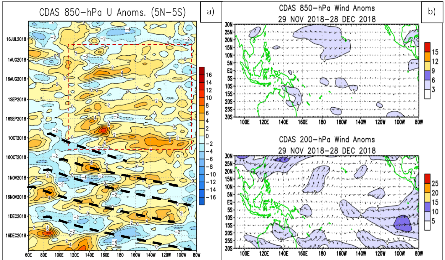
Figura 7. Anomalías campos de vientos sobre el Océano Pacífico Ecuatorial (OPE) para el periodo comprendido entre el 29 de Noviembre al 28 Diciembre del 2018. Fuente: Climate Prediction Center-NOAA.
