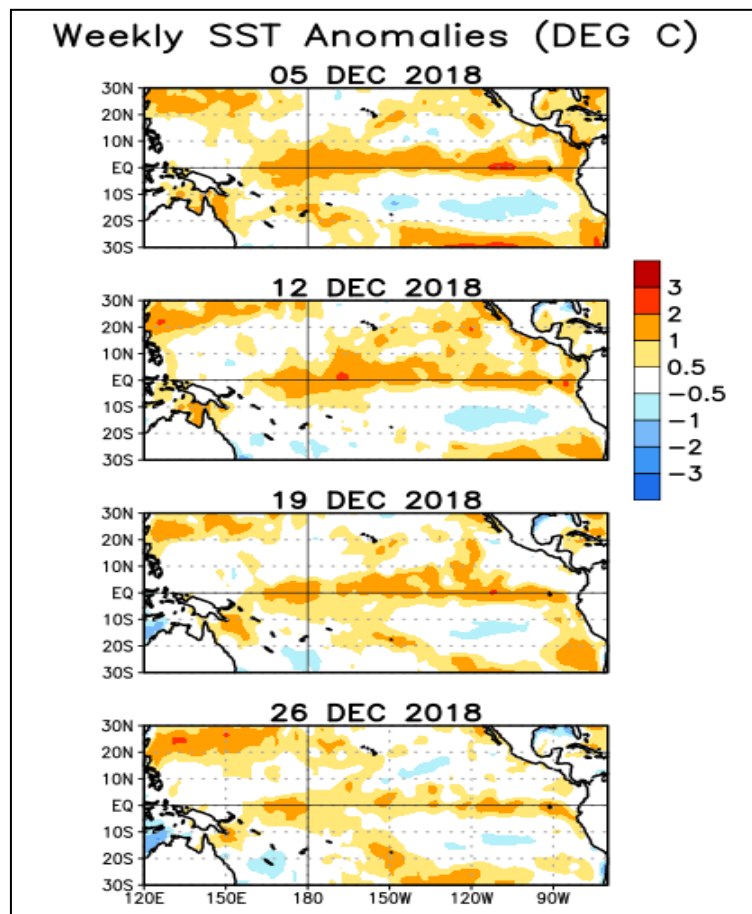
Figura 3. Anomalías semanales de TSM en el Océano Pacífico Tropical para el periodo comprendido entre el 05 y el 26 de Diciembre del 2018. Fuente: Climate Prediction Center-NOAA.
