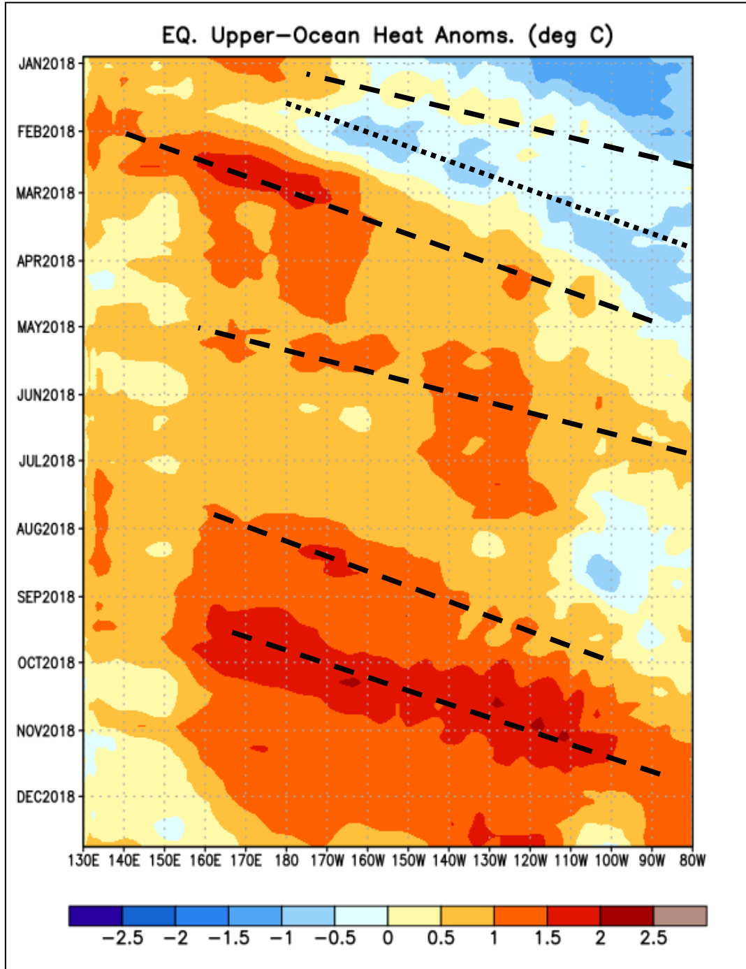
Figura 9. Evolución de las Ondas Oceánicas Kelvin de Hundimiento y Afloramiento, en el Océano Pacífico Ecuatorial (OPE). La escala de colores representa la magnitud de las anomalías en °C. Fuente: Climate Prediction Center-NOAA.
