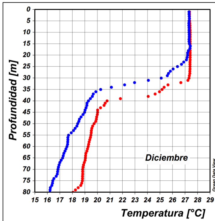
Figura 12. Perfil de temperatura para el mes de Diciembre del 2018 registrado en la estación costera fija de Tumaco. En color rojo se presenta el perfil obtenido en la primera quincena del mes y en azul el realizado a finales del mismo. Fuente: CCCP
