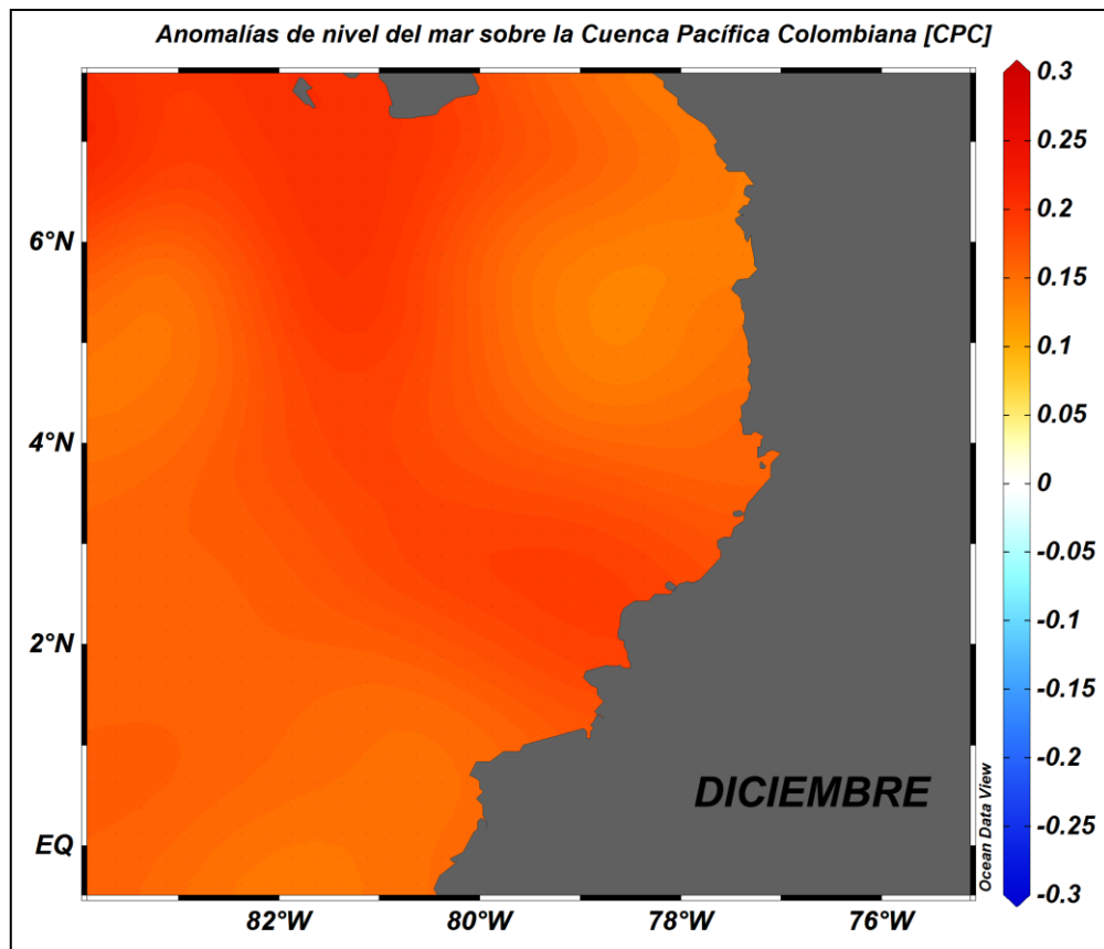
Figura 6. Anomalías de nivel del mar CPC, Diciembre del 2018 (Fuente: Copernicus Marine Service (CMEMS), Procesamiento: CIOHP).
