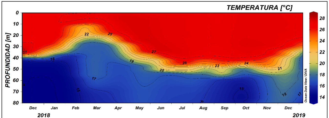
Figura 11. Serie temporal de temperatura del agua en la estación costera fija de Tumaco entre 0 a 80 metros de profundidad, para el periodo comprendido entre diciembre del 2017 y Diciembre del 2018. La escala de colores representa la magnitud de la temperatura medida en °C. Fuente: CCCP.
