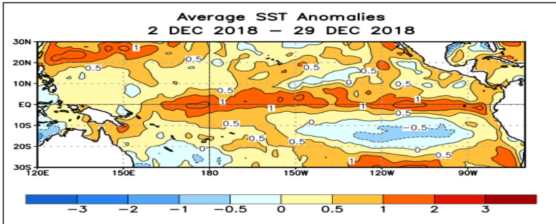
Figura 2. Anomalías de TSM en el Océano Pacífico Tropical para el periodo comprendido entre el 02 y el 29 de Diciembre del 2018. La escala de colores representa la magnitud en °C. Fuente: Climate Prediction Center – NOAA.
