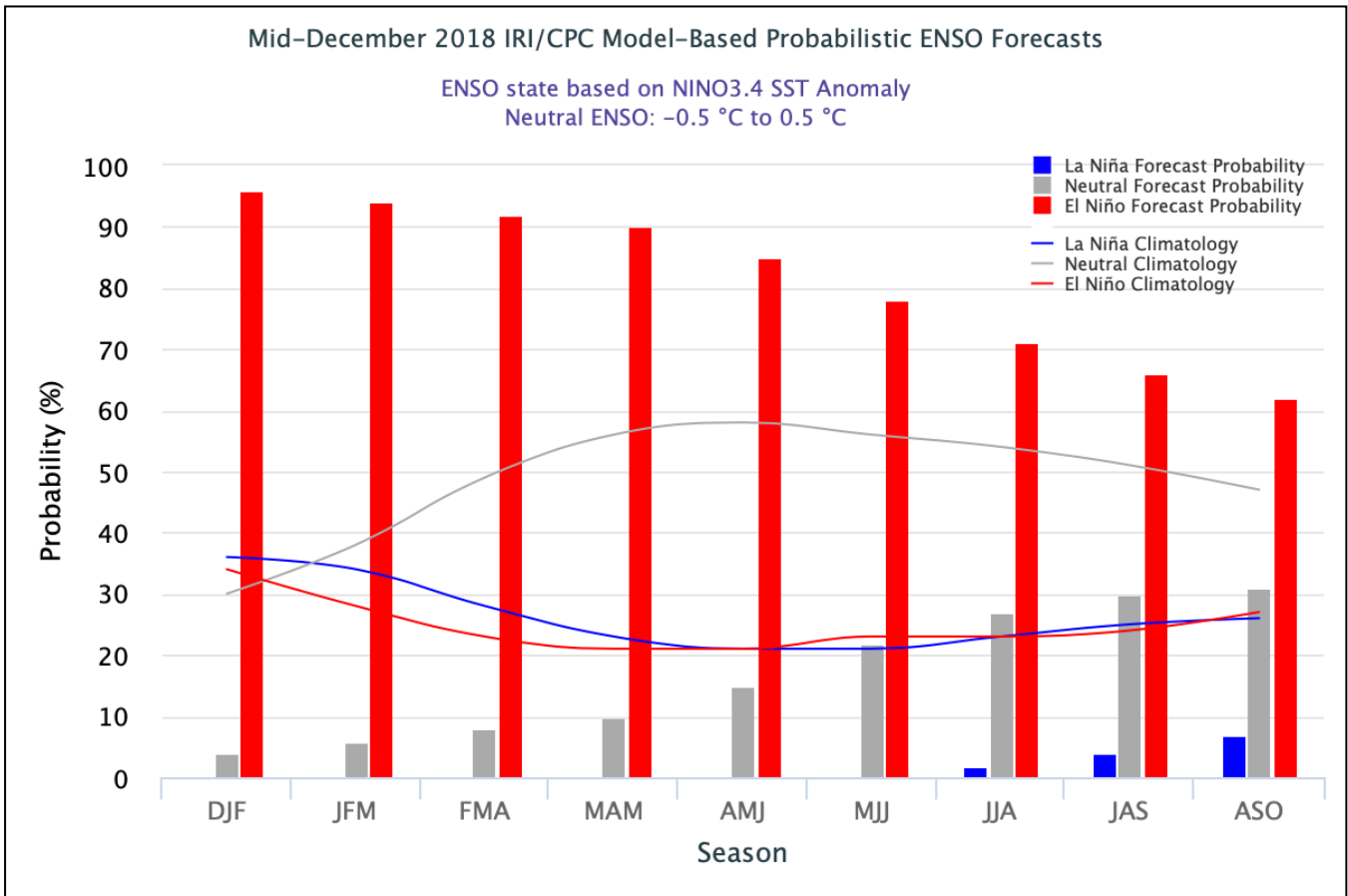
Figura 16. Predicción modelos estadísticos y dinámicos de condiciones ENOS Diciembre del 2018. (Fuente: IRI/CPC).
