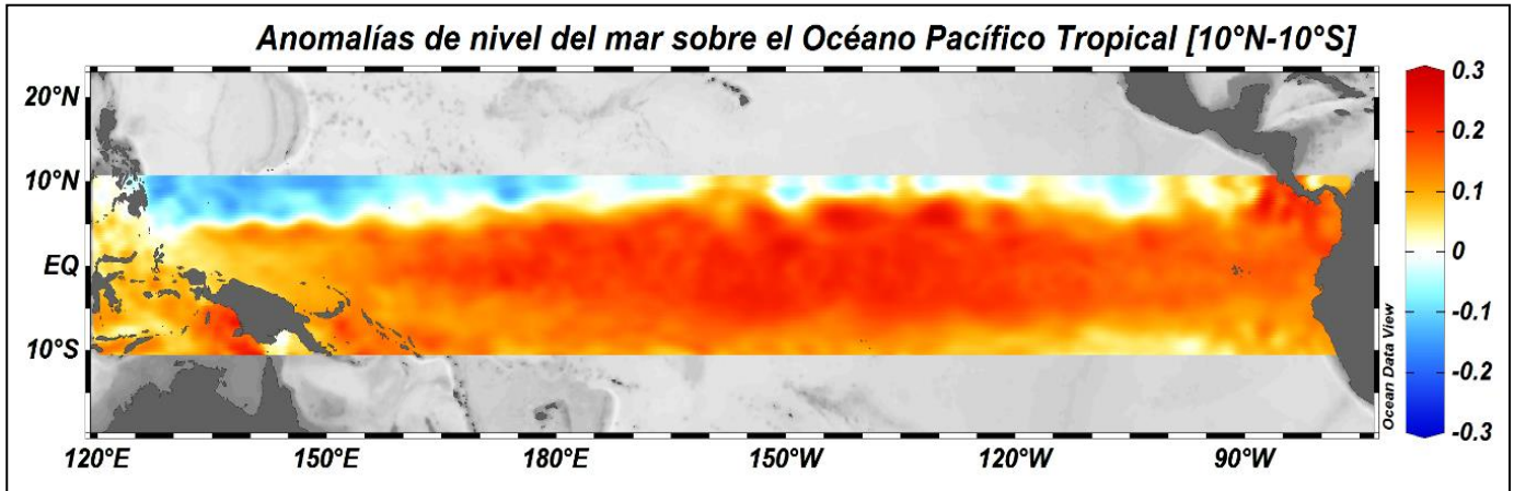
Figura 5. Anomalías de nivel del mar Océano Pacífico Tropical para el mes de Diciembre del 2018. La escala de colores representa la magnitud media en metros (m) (Fuente: Copernicus Marine Service (CMEMS), Procesamiento: CIOHP).
