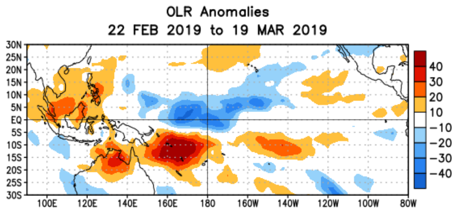
Figura 8. Anomalías Radiación de Onda Larga (OLR, por sus siglas en inglés) Para el periodo comprendido entre el 22 de febrero al 19 de marzo del 2019. La escala de colores representa en W/m^2 . Fuente: Climate Prediction Center-NOAA.
