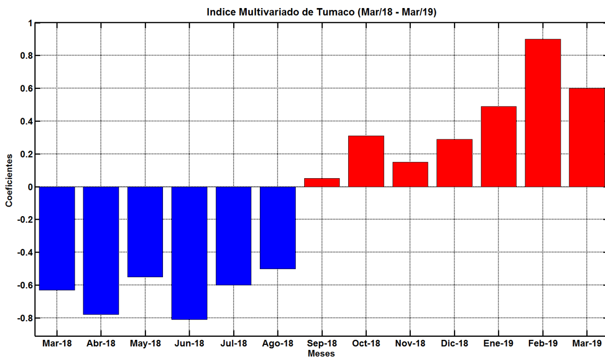
Figura 13. Comportamiento del Índice Multivariado de Tumaco (IMT) para el periodo comprendido entre marzo del 2018 y marzo del 2019. Fuente: CCCP.
