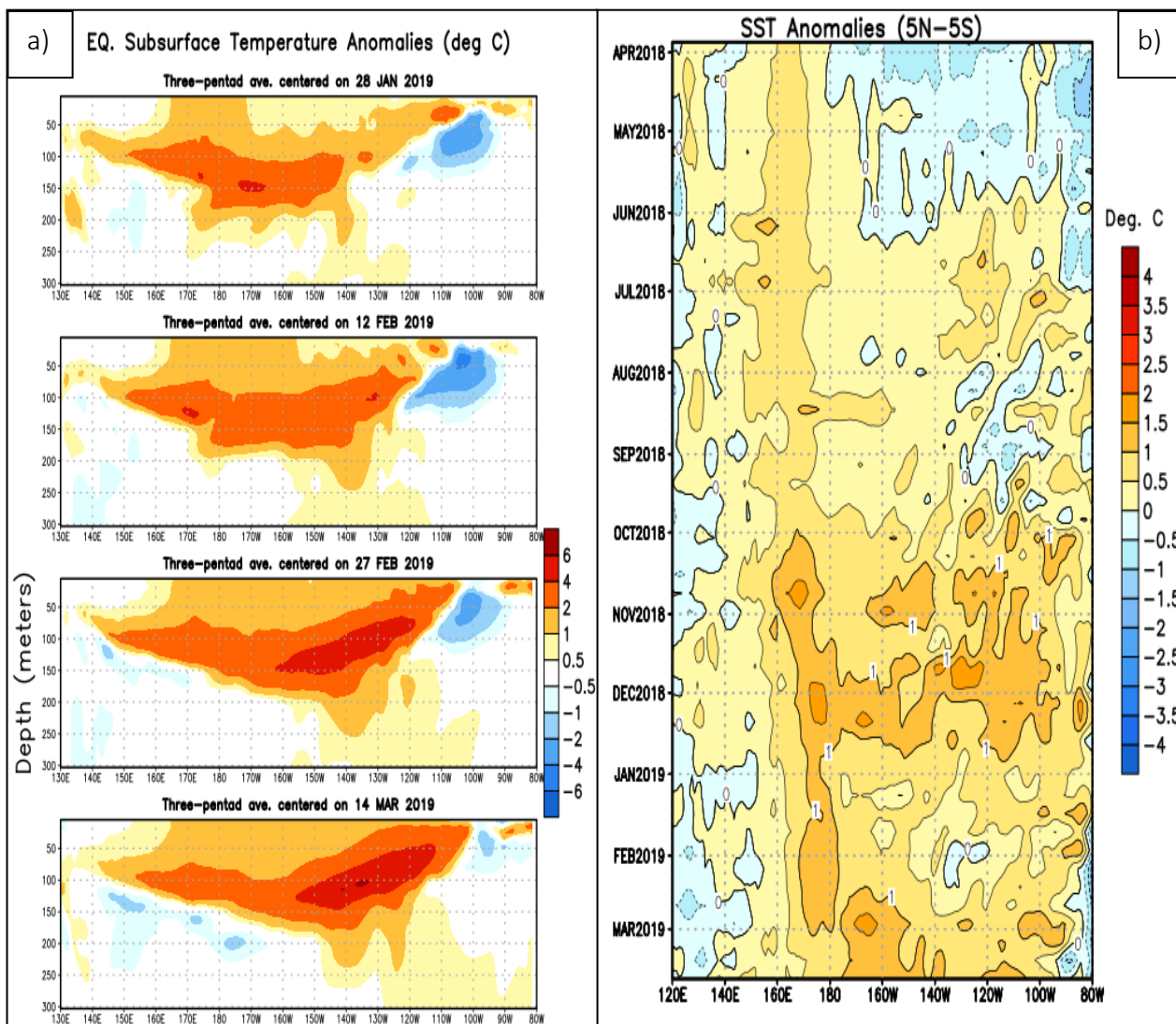
Figura 1. Evolución de las anomalías de temperatura subsuperficial (a) en el Océano Pacífico Ecuatorial (OPE) y superficiales (b) entre latitudes 5°S y 5°N para el periodo comprendido entre el 28 de enero y el 14 de marzo de 2019. La escala de colores representa la magnitud de las anomalías en °C. Fuente: Climate Prediction Center-NOAA.
