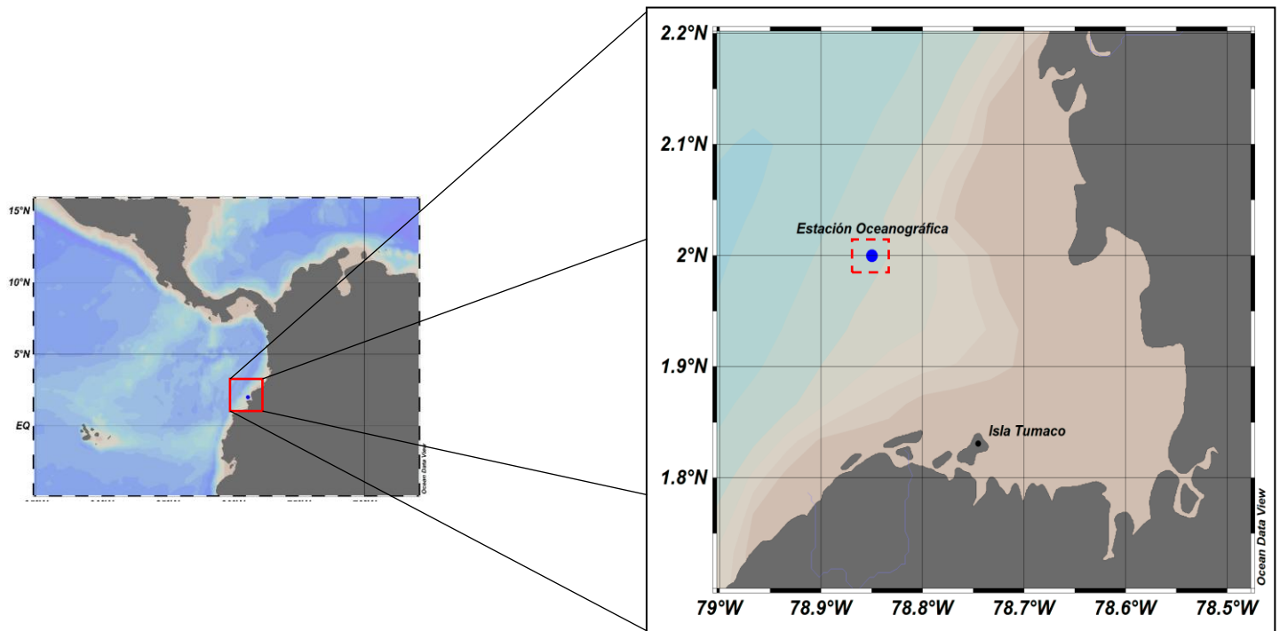
Figura 10. Ubicación geográfica de la estación costera fija de Tumaco en el Pacífico colombiano ( 02^{\circ}00'00''\text{N} - 78^{\circ}48'00''\text{W} ). Fuente ODV.
