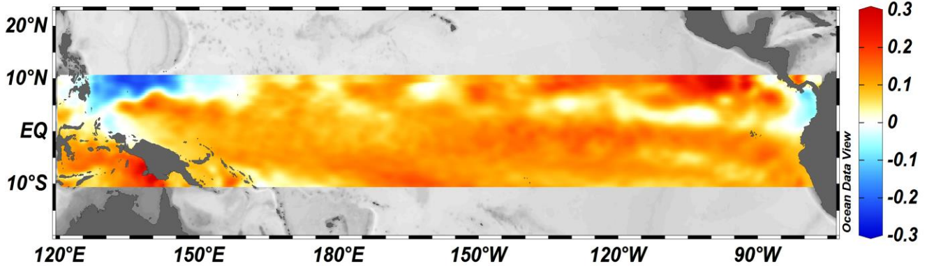
Figura 5. Anomalías de nivel del mar Océano Pacífico Tropical para el mes de marzo del 2019. La escala de colores representa la magnitud media en metros (m) (Fuente: Copernicus Marine Service (CMEMS), Procesamiento: CIOHP).
