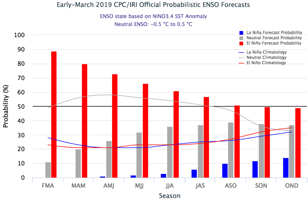
Figura 14. Predicción modelos estadísticos y dinámicos de condiciones IRI ENOS 12 de marzo del 2019. (Fuente: IRI/CPC).
