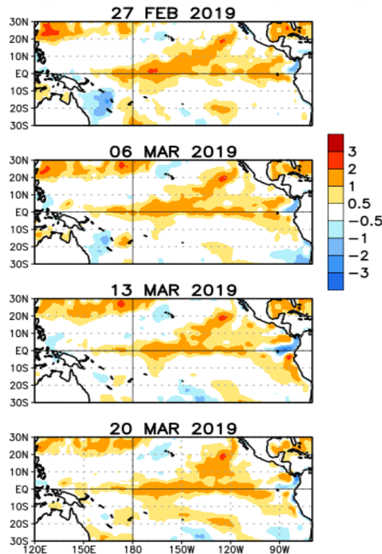
Figura 3. Anomalías semanales de TSM en el Océano Pacífico Tropical para el periodo comprendido entre el 27 de febrero y el 20 de marzo del 2019. Fuente: Climate Prediction Center-NOAA.
