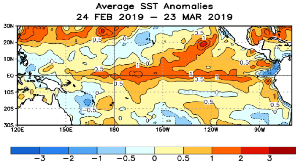
Figura 2. Anomalías de TSM en el Océano Pacífico Tropical para el periodo comprendido entre el 24 de febrero y el 23 de marzo del 2019. La escala de colores representa la magnitud en °C. Fuente: Climate Prediction Center – NOAA.
