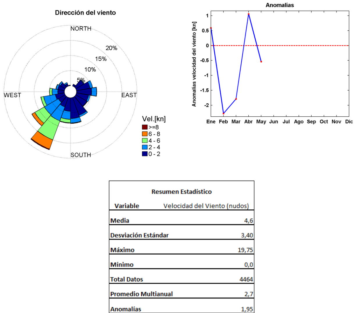
Figura 12. Distribución de frecuencia de la dirección, velocidad, anomalía velocidad y resumen estadístico del viento en Buenaventura.
