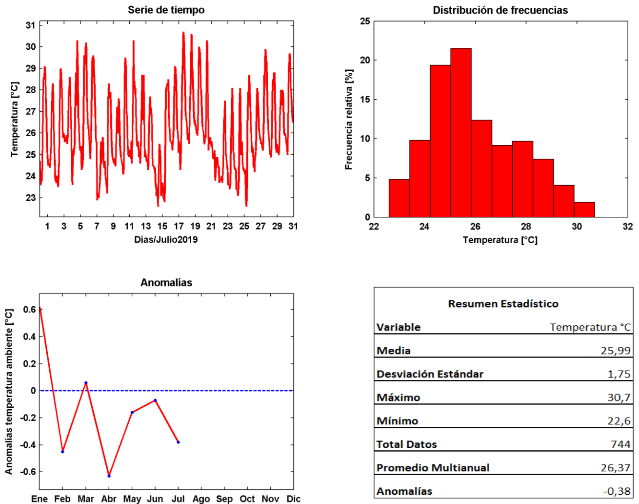
Figura 2. Serie de tiempo, histograma de frecuencia, anomalía y resumen estadístico mensual de la temperatura ambiente en Bahía Solano.
