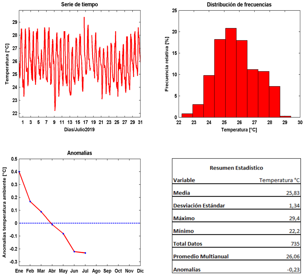
Figura 13. Serie de tiempo, histograma de frecuencia, anomalía y resumen estadístico mensual de la temperatura ambiente en Tumaco.
