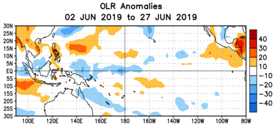
Figura 8. Anomalías Radiación de Onda Larga (OLR, por sus siglas en inglés) Para el periodo comprendido entre el 02 y el 27 de junio del 2019. La escala de colores representa en W/m^2 . Fuente: Climate Prediction Center-NOAA.
