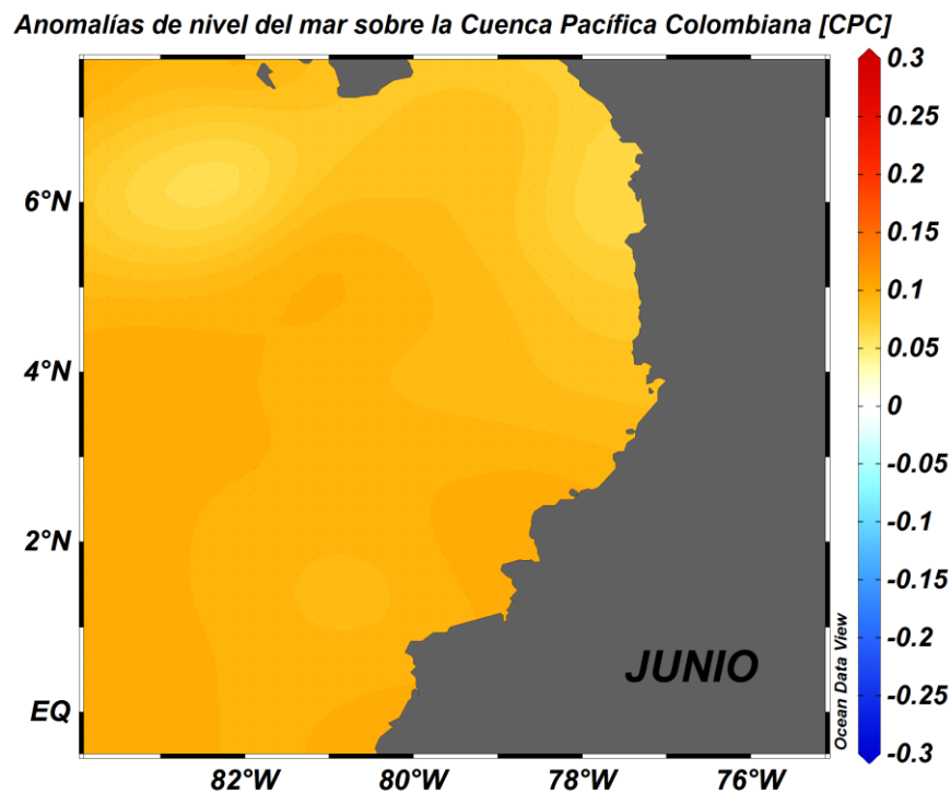
Figura 6. Anomalías de nivel del mar CPC, junio del 2019 (Fuente: Copernicus Marine Service (CMEMS), Procesamiento: CIOHP).
