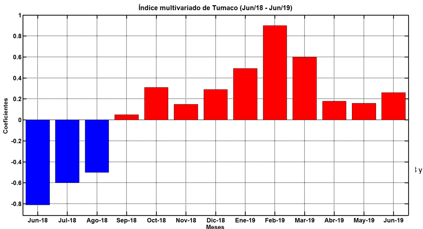
Figura 13 Comportamiento del Índice Multivariado de Tumaco (IMT) para el periodo comprendido entre junio del 2018 y junio del 2019. Fuente: CCCP.
