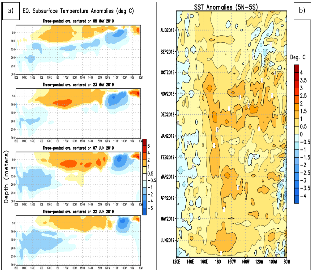
Figura 1. Evolución de las anomalías de temperatura subsuperficial (a) en el Océano Pacífico Ecuatorial (OPE) y superficiales (b) entre latitudes 5°S y 5°N para el periodo comprendido entre el 08 de mayo al 22 de junio de 2019. La escala de colores representa la magnitud de las anomalías en °C. Fuente: Climate Prediction Center-NOAA.
