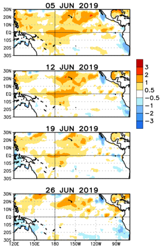
Figura 3. Anomalías semanales de TSM en el Océano Pacífico Tropical para el periodo comprendido del 05 al 26 de junio del 2019. Fuente: Climate Prediction Center-NOAA.
