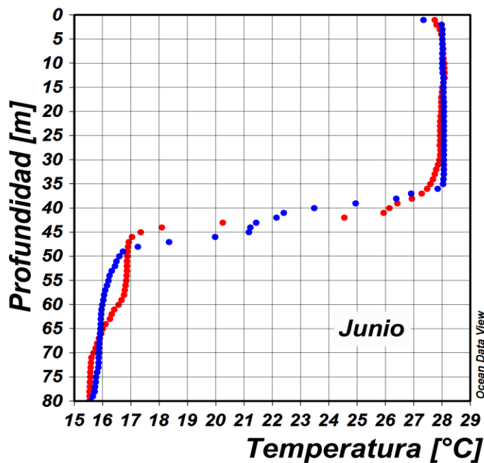
Figura 12. Perfil de temperatura para el mes de junio del 2019 registrado en la estación costera fija de Tumaco. En color rojo se presenta el perfil obtenido en la primera quincena del mes y en azul el realizado a finales del mismo. Fuente: CCCP.
