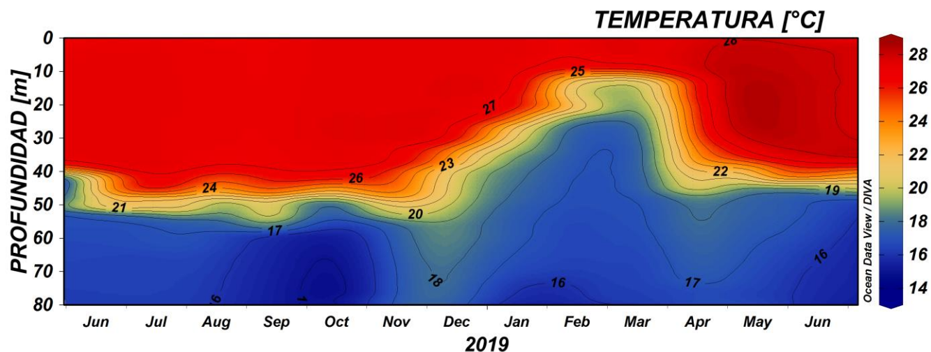
Figura 11. Serie temporal de temperatura del agua en la estación costera fija de Tumaco entre 0 a 80 metros de profundidad, para el periodo comprendido entre junio del 2018 y junio del 2019. La escala de colores representa la magnitud de la temperatura medida en °C. Fuente: CCCP.
