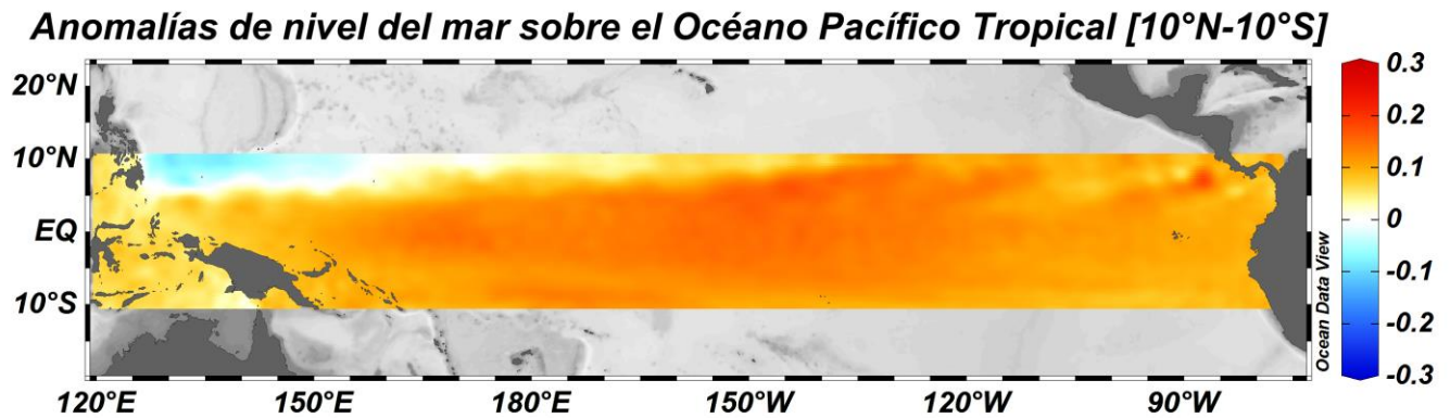
Figura 5. Anomalías de nivel del mar Océano Pacífico Tropical para el mes de junio del 2019. La escala de colores representa la magnitud media en metros (m) (Fuente: Copernicus Marine Service (CMEMS), Procesamiento: CIOHP).
