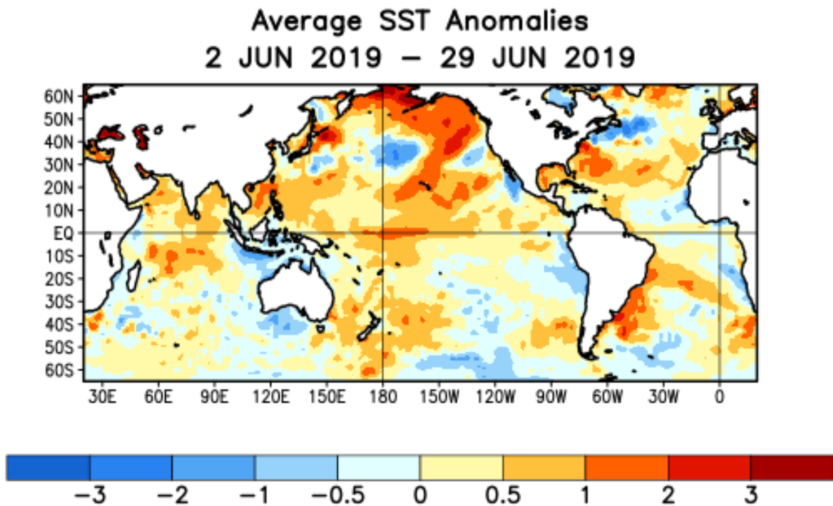
Figura 2. Anomalías de TSM en el Océano Pacífico Tropical para el periodo comprendido entre el 2 al 29 de junio del 2019. La escala de colores representa la magnitud en °C. Fuente: Climate Prediction Center – NOAA.
