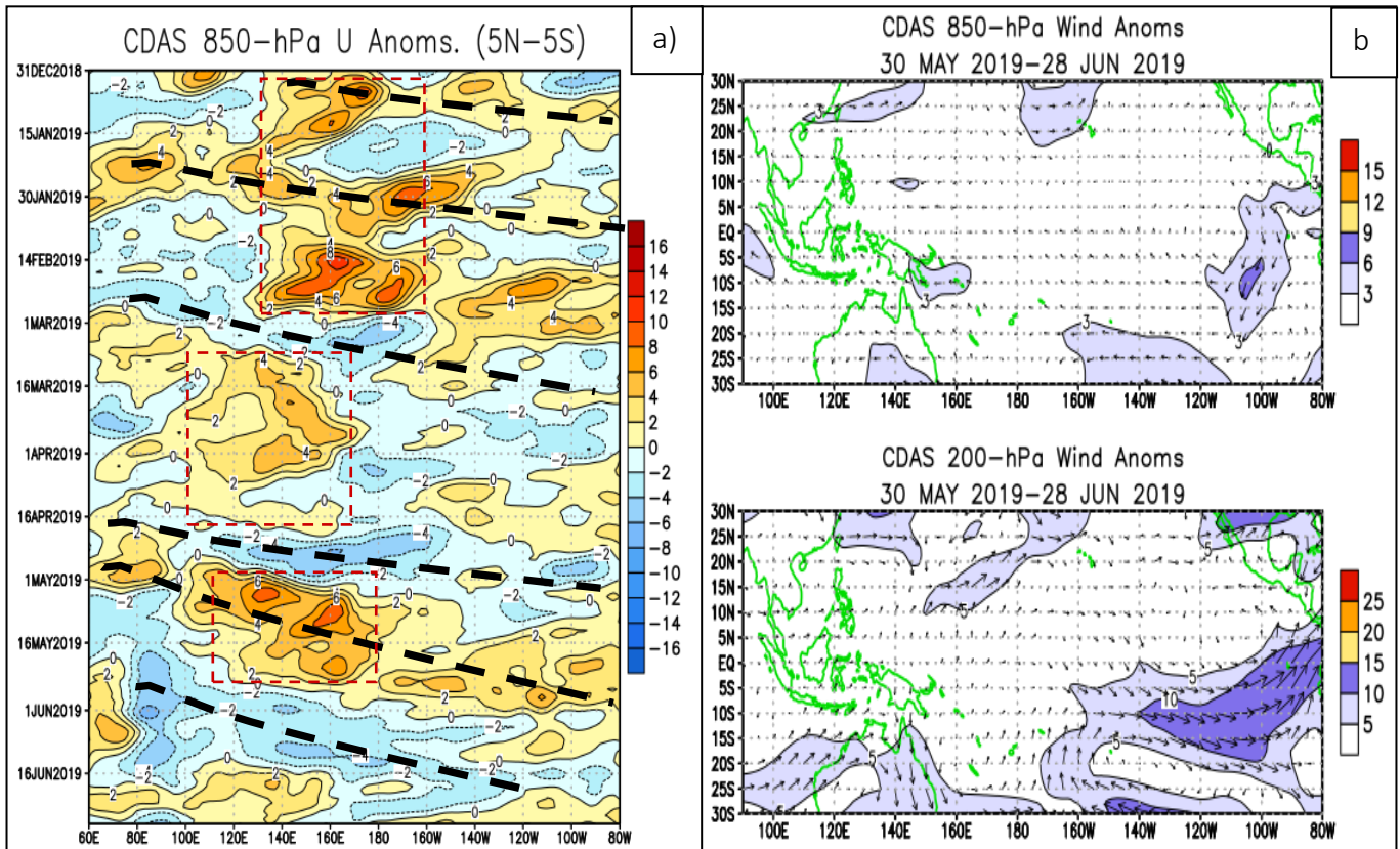
Figura 7. Anomalías campos de vientos sobre el Océano Pacífico Ecuatorial (OPE) para el periodo comprendido entre el 30 de mayo al 28 de junio del 2019. Fuente: Climate Prediction Center-NOAA.
