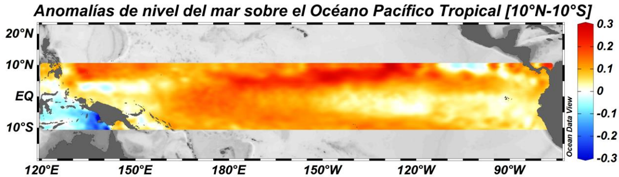
Figura 5. Anomalías de nivel del mar en el Océano Pacífico Tropical (OPT) para el mes de agosto del 2019. La escala de colores representa la magnitud de la variable medida en metros (m) (Fuente: Copernicus Marine Service (CMEMS), Procesamiento: CCCP).
