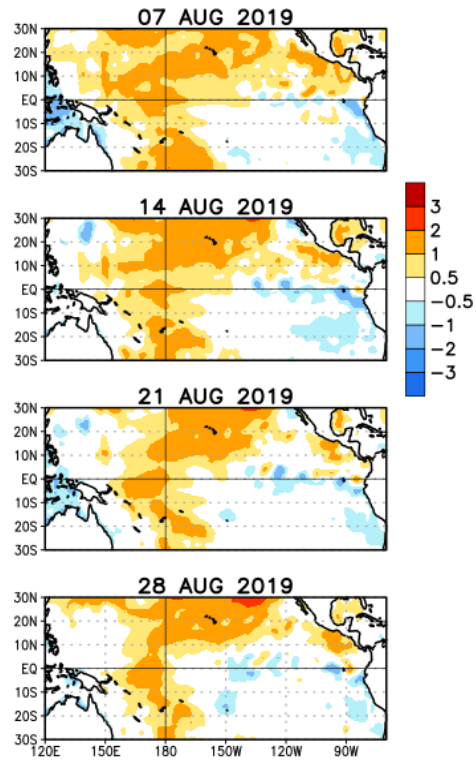
Figura 3. Anomalías semanales de TSM en el Océano Pacífico Tropical para el periodo comprendido del 07 al 28 de agosto del 2019. Fuente: Climate Prediction Center-NOAA.
