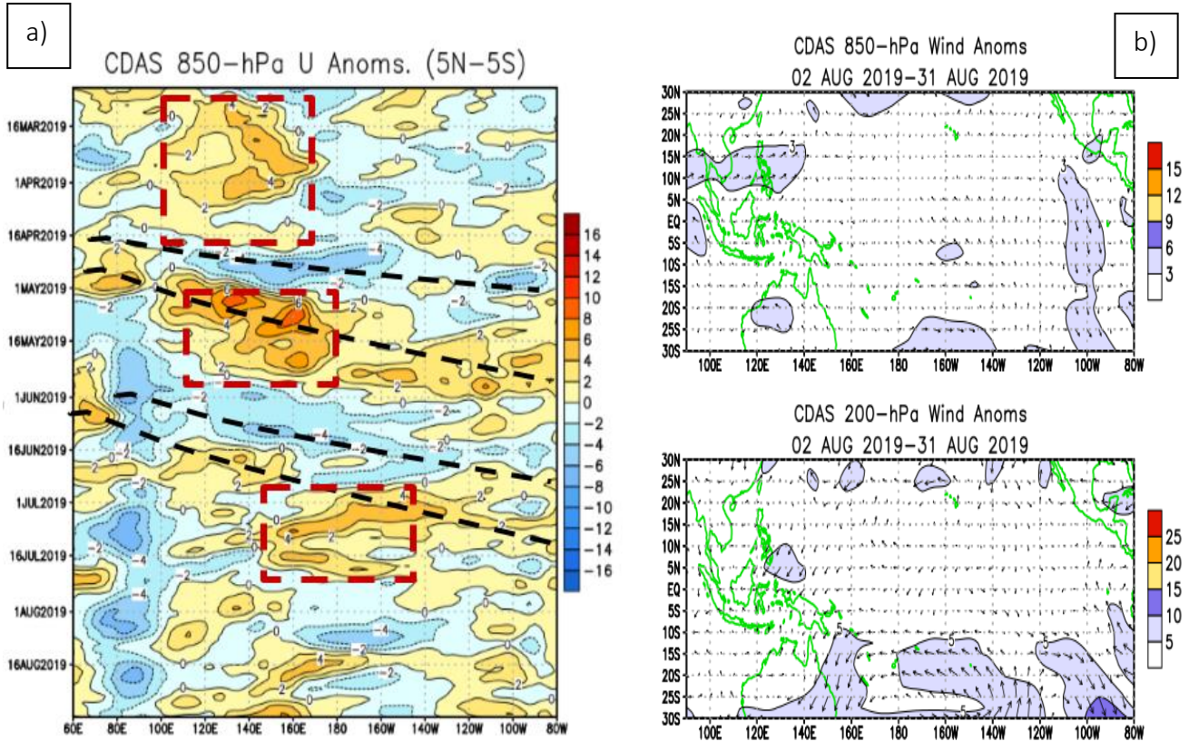
Figura 7. Anomalías campos de vientos sobre el Océano Pacífico Ecuatorial (OPE) para el periodo comprendido entre el 02 al 31 de agosto del 2019. Fuente: Climate Prediction Center-NOAA.
