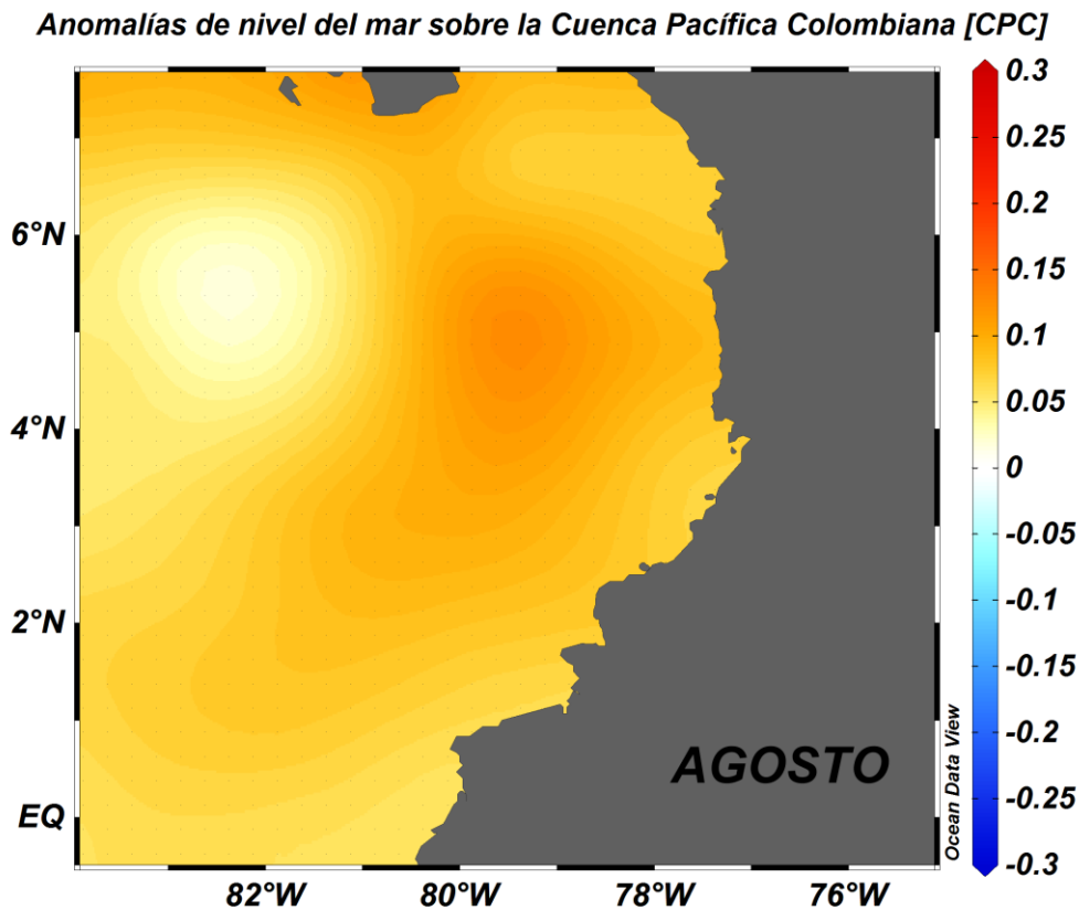
Figura 6. Anomalías de nivel del mar en la Cuenca Pacífica Colombiana (CPC) para el mes de agosto del 2019 (Fuente: Copernicus Marine Service (CMEMS), Procesamiento: CCCP).
