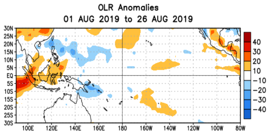
Figura 8. Anomalías Radiación de Onda Larga (OLR, por sus siglas en inglés) Para el periodo comprendido entre el 01 al 26 de agosto del 2019. La escala de colores representa en W/m^2 . Fuente: Climate Prediction Center-NOAA.
