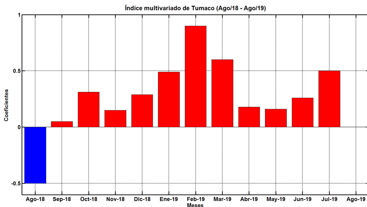
Figura 13. Comportamiento del Índice Multivariado de Tumaco (IMT) para el periodo comprendido entre agosto del 2018 y agosto del 2019. Fuente: CCCP.
