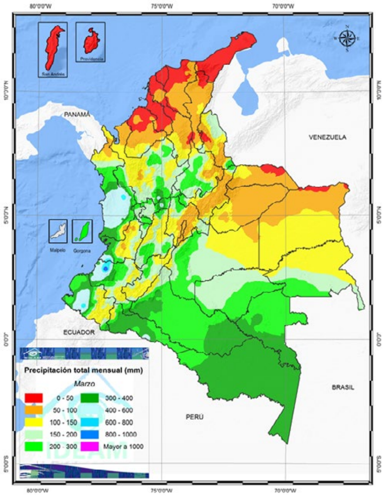
Figura 8. Mapa de precipitación acumulada climatológica promedio del mes de marzo, para el período 1981-2010. Fuente: IDEAM
