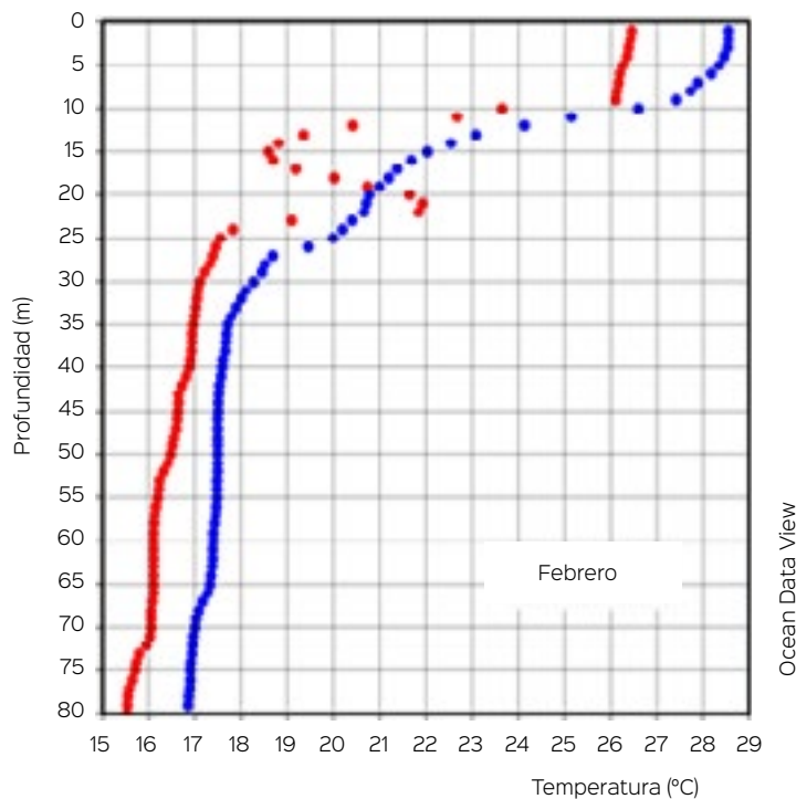
Figura 1. Muestreo realizado el 14 de febrero en línea roja y en azul muestreo realizado el día 04 de marzo. Fuente: CCCP
