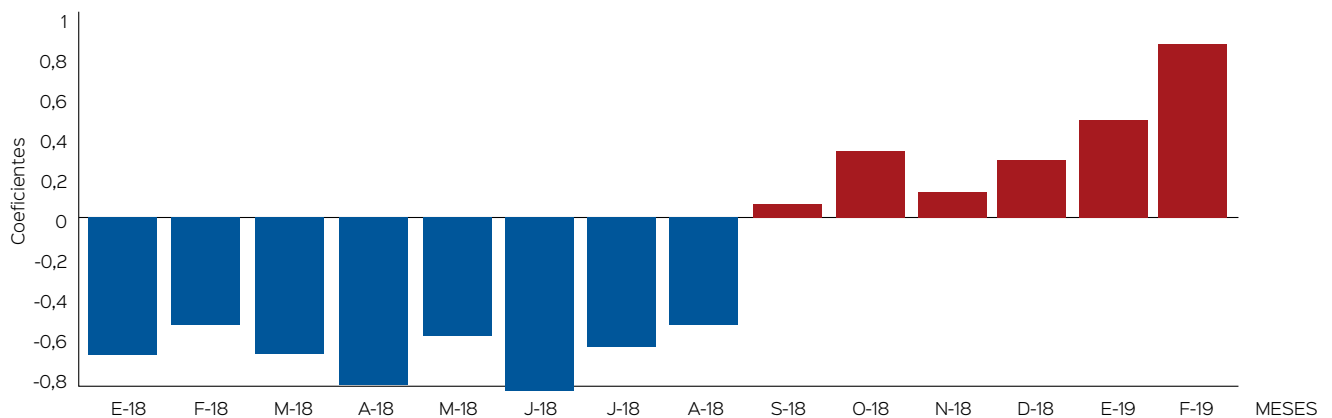
Figura 3. Comportamiento del Índice Multivariado de Tumaco (IMT) para el periodo comprendido entre enero del 2018 y febrero del 2019. Fuente: CCCP
