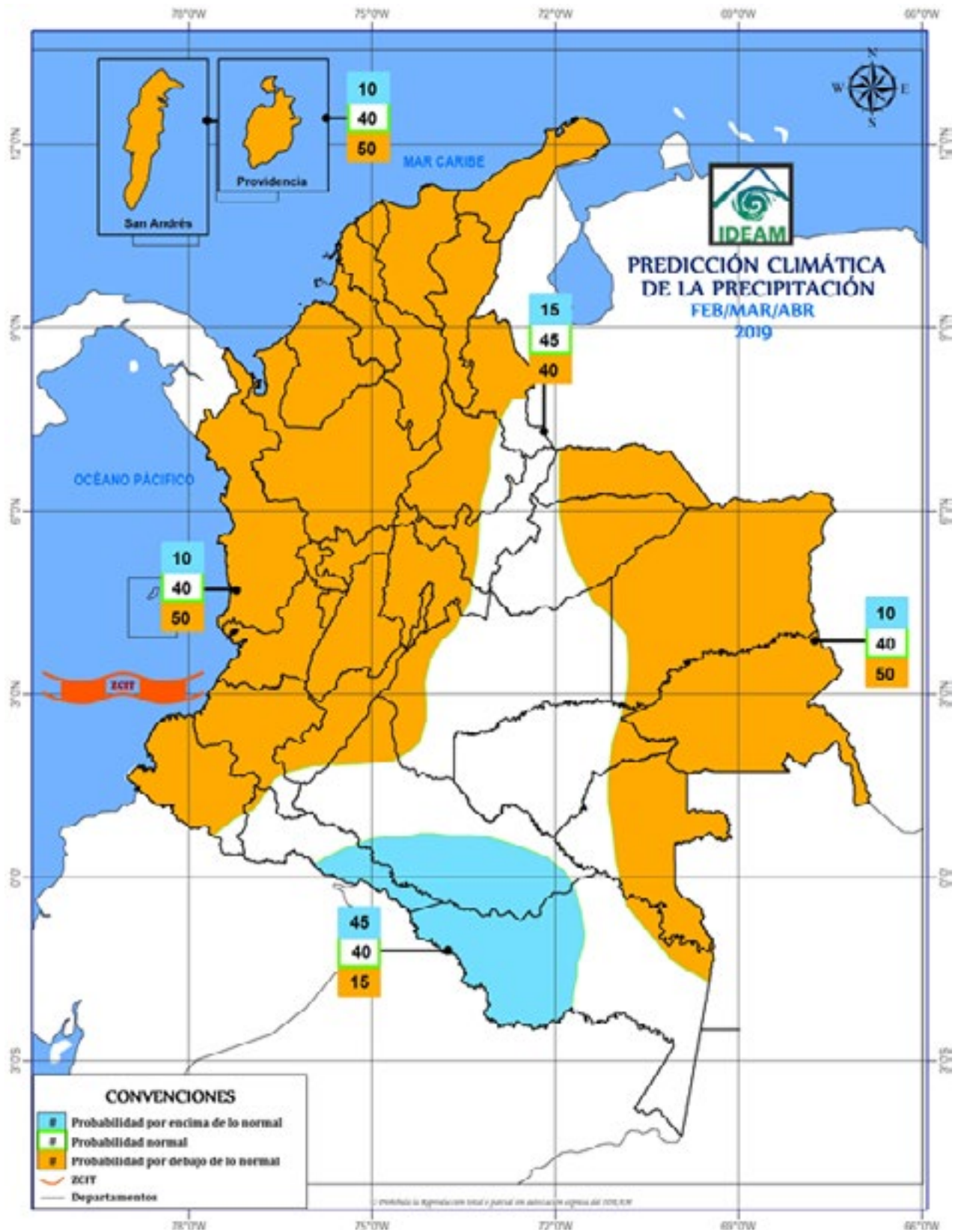
Figura 9. Mapa de predicción de la precipitación acumulada trimestre MAM de 2019, por consenso. Fuente: IDEAM
