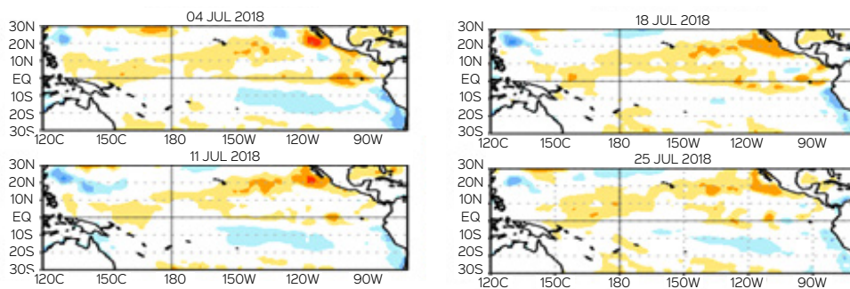
Figura 5. Anomalías semanales de TSM en el Océano Pacífico Tropical para el periodo comprendido entre el 04 y el 25 de julio del 2018. Fuente: Climate Prediction Center-NOAA.
