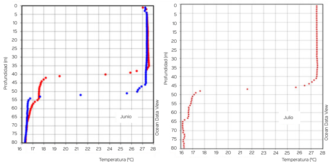
Figura 1. Izq. Muestreo realizado el 15 de junio (línea roja) y el 25 de junio del 2018 (línea azul). Der. Muestreo realizado el 13 de julio (línea roja).
