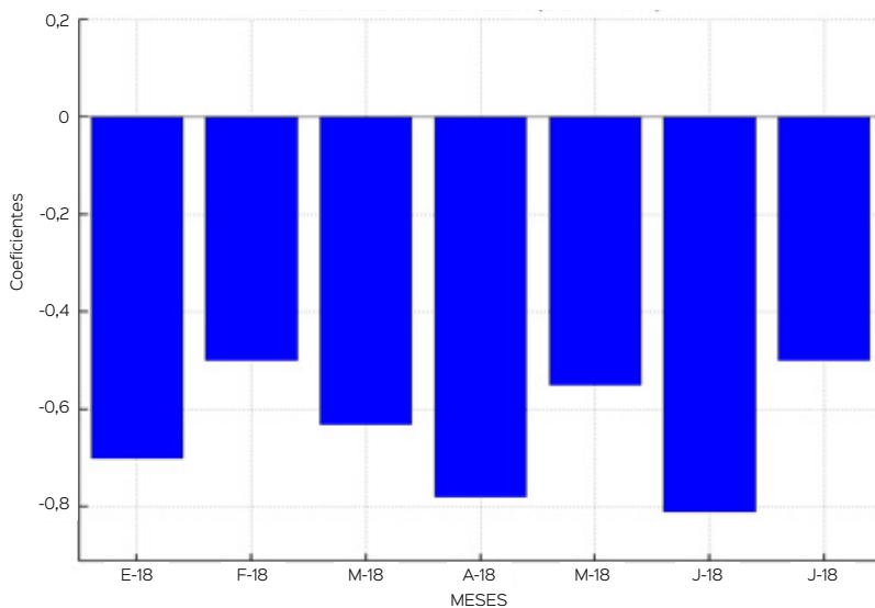
Figura 3. Comportamiento del Índice Multivariado de Tumaco (IMT) para el periodo comprendido entre enero del 2018 y julio del 2018. Fuente: CCCP.
