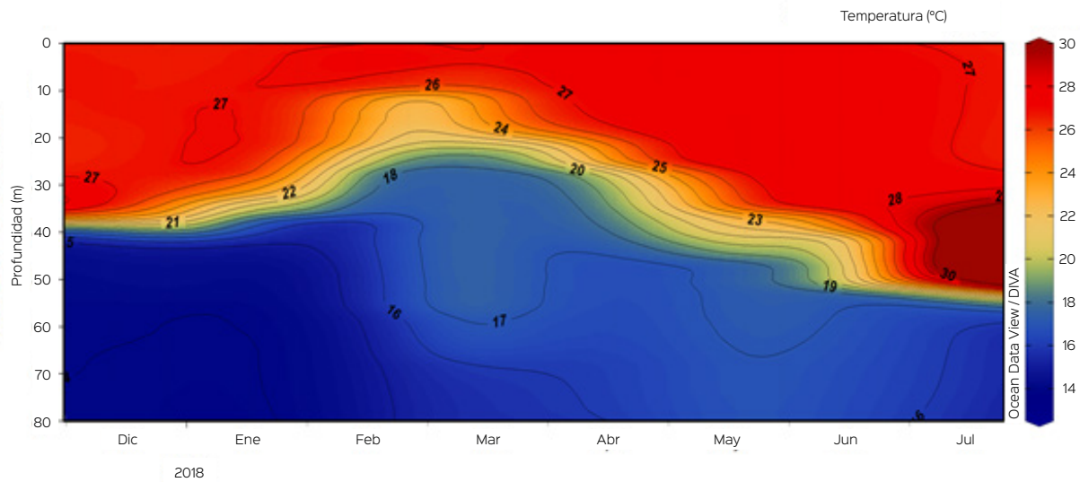
Figura 2. Serie temporal de temperatura del agua en la estación costera fija de Tumaco entre 0 a 80 metros de profundidad, para el periodo de comprendido entre diciembre del 2017 y julio del 2018. La escala de colores representa la magnitud de la temperatura medida en °C. Fuente: CCCP.
