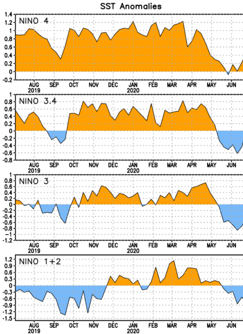
Figura 4. Evolución de las anomalías en la TSM monitoreadas en las regiones Niño 4, 3.4, 3 y 1+2 de la NOAA. Los valores ubicados en el eje Y, representan las magnitudes de las anomalías en °C. Fuente: Climate Prediction Center-NOAA.
