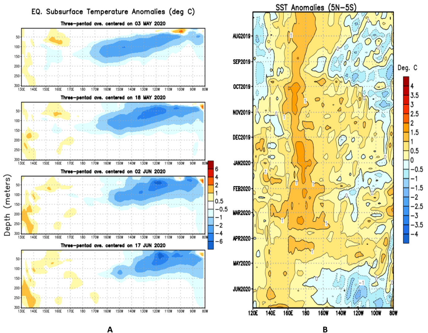
Figura 1. Evolución de las anomalías de temperatura subsuperficial (A) en el (OPE) y superficiales (B) entre latitudes 5^{\circ}\text{S} y 5^{\circ}\text{N} para el periodo comprendido entre el 03 de mayo al 17 de junio del 2020. La escala de colores representa la magnitud de las anomalías en ^{\circ}\text{C} . Fuente: Climate Prediction Center-NOAA.
