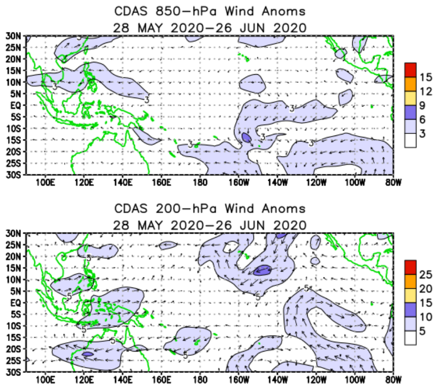
Figura 7. Anomalías campos de vientos sobre el Océano Pacífico Ecuatorial (OPE) para el periodo comprendido del 28 de mayo al 26 de junio de 2020. Fuente: Climate Prediction Center-NOAA.
