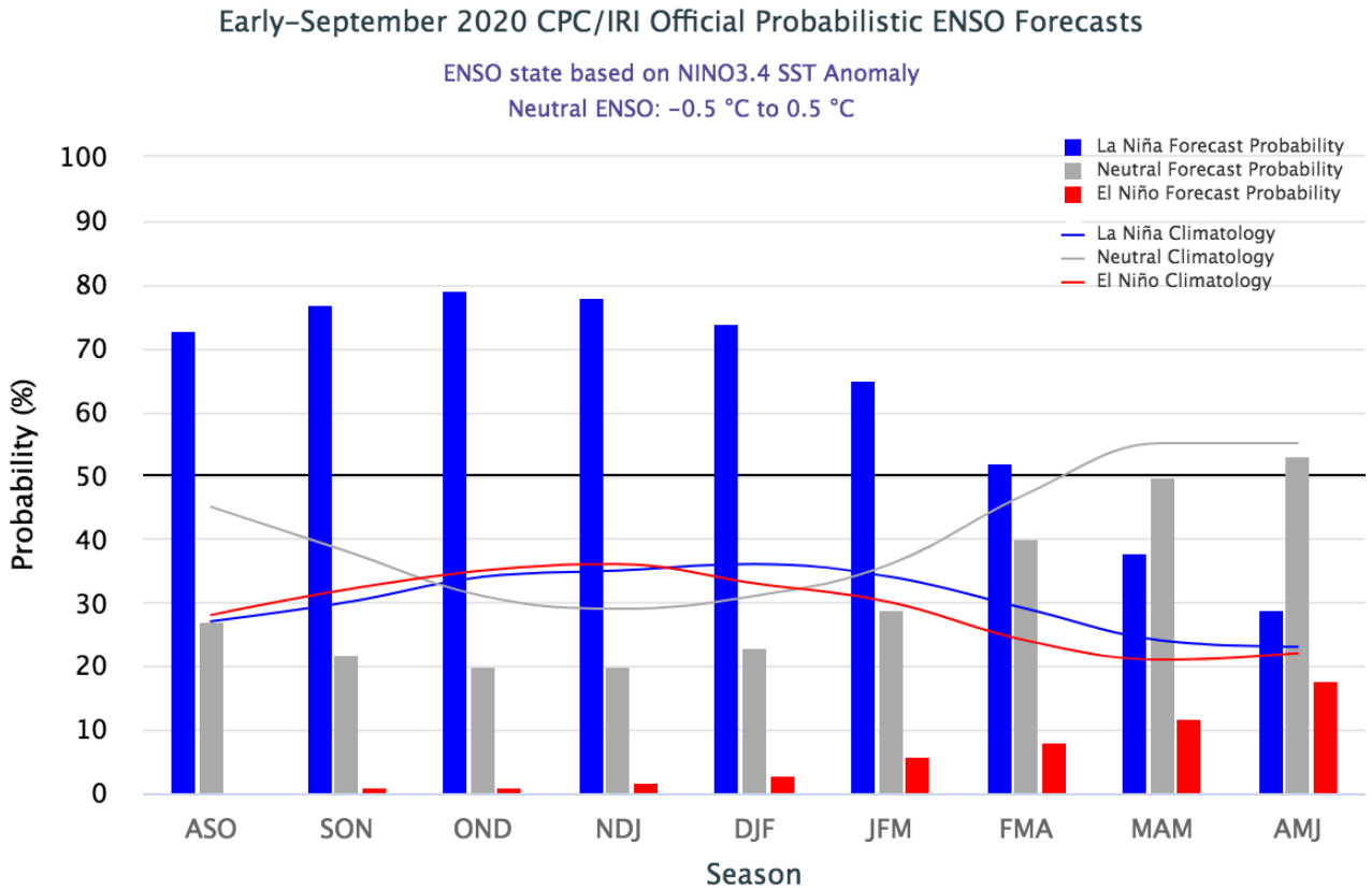
Figura 14. Predicción modelos estadísticos y dinámicos de condiciones IRI ENOS 10 de septiembre del 2020. (Fuente: IRI/CPC).
