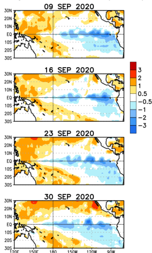
Figura 3. Anomalías semanales de TSM en el Océano Pacífico Tropical para el periodo comprendido del 09 al 30 de septiembre del 2020. Fuente: Climate Prediction Center-NOAA.
