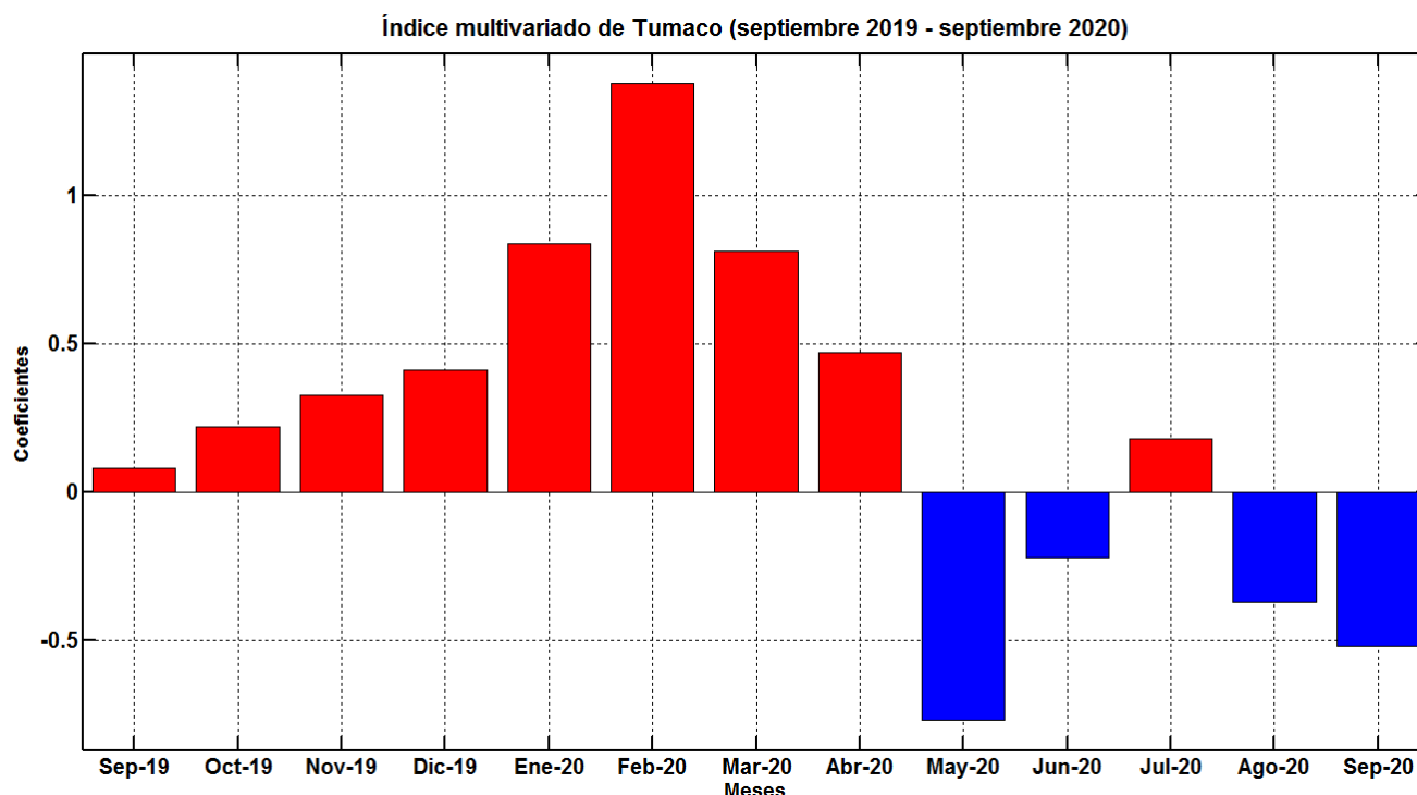
Figura 13. Comportamiento del Índice Multivariado de Tumaco (IMT) para el periodo comprendido entre septiembre del 2019 y septiembre del 2020. Fuente: CCCP.
