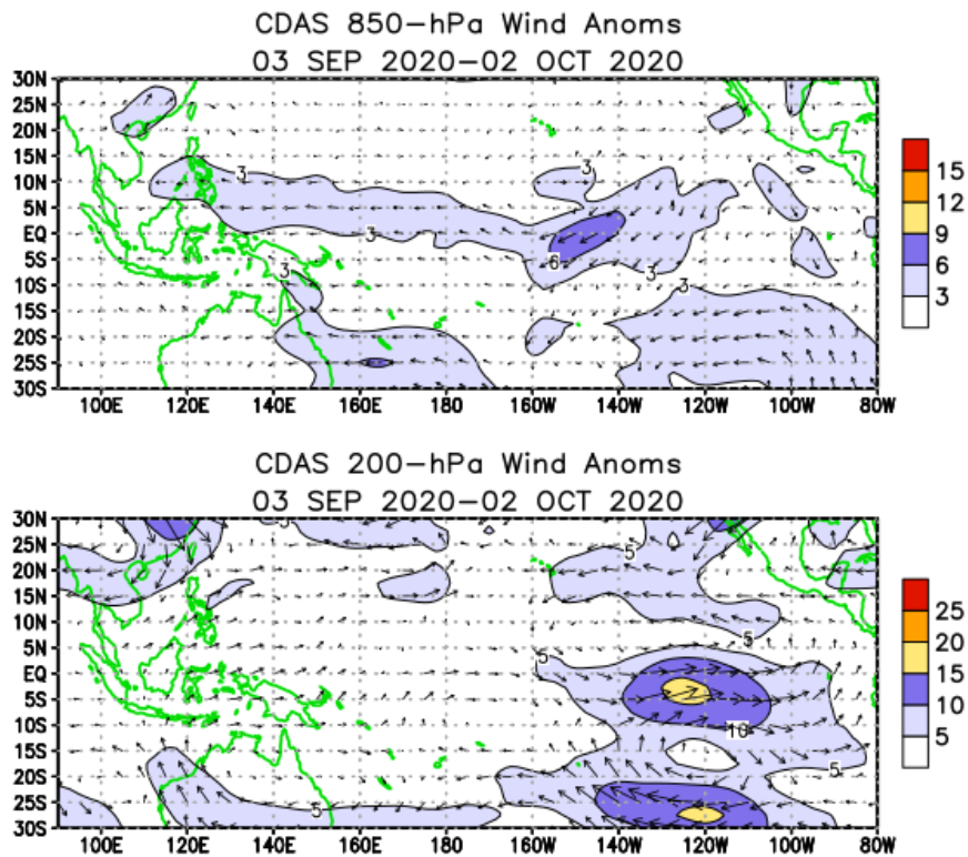
Figura 7. Anomalías campos de vientos sobre el Océano Pacífico Ecuatorial (OPE) para el periodo comprendido del 03 de septiembre al 02 de octubre de 2020. Fuente: Climate Prediction Center-NOAA.
