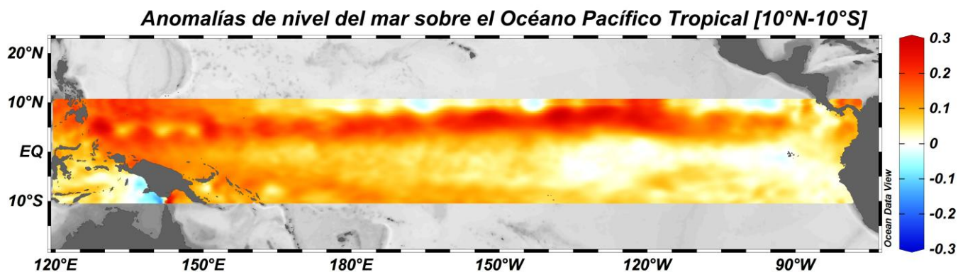
Figura 5. Anomalías de nivel del mar en el Océano Pacífico Tropical (OPT) para el mes de septiembre del 2020. La escala de colores representa la magnitud de la variable medida en metros (m) (Fuente: Copernicus Marine Service (CMEMS), Procesamiento: CCCP).
