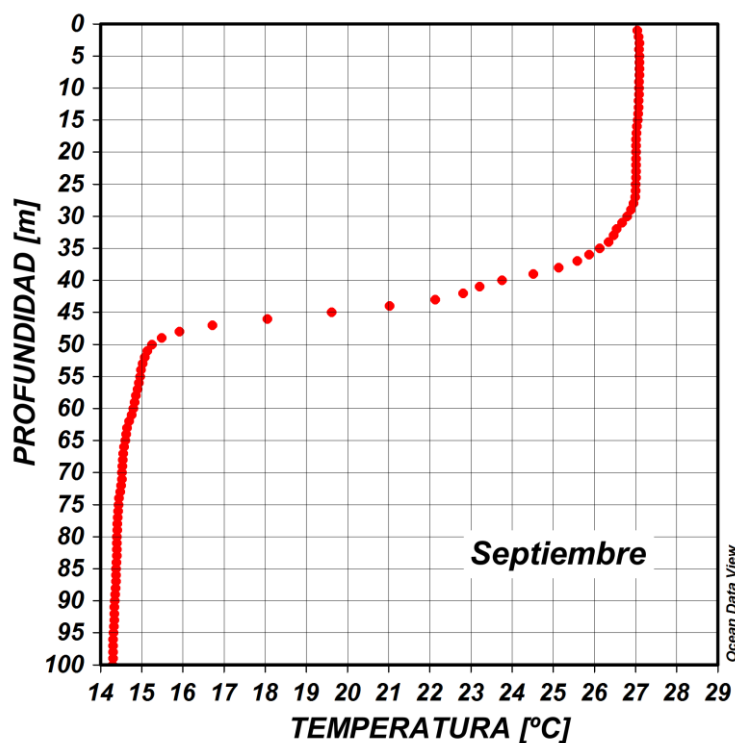
Figura 12. Perfil de temperatura para el mes de septiembre del 2020 registrado en la estación costera fija de Tumaco. Fuente: CCCP.
