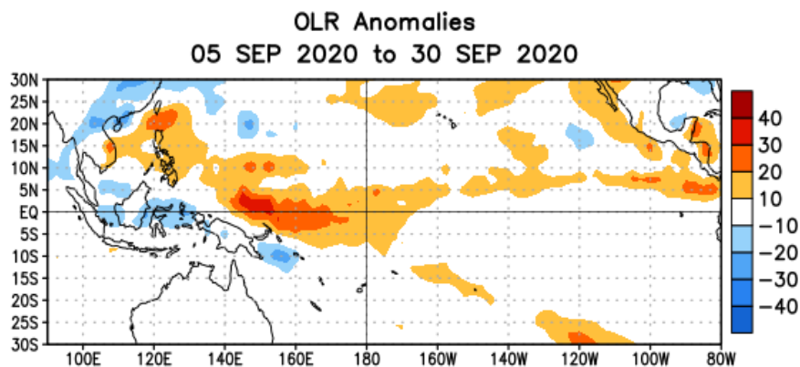
Figura 8. Anomalías Radiación de Onda Larga (OLR, por sus siglas en inglés) Para el periodo comprendido del 05 al 30 de septiembre del 2020. La escala de colores representa en W/m^2 . Fuente: Climate Prediction Center-NOAA.
