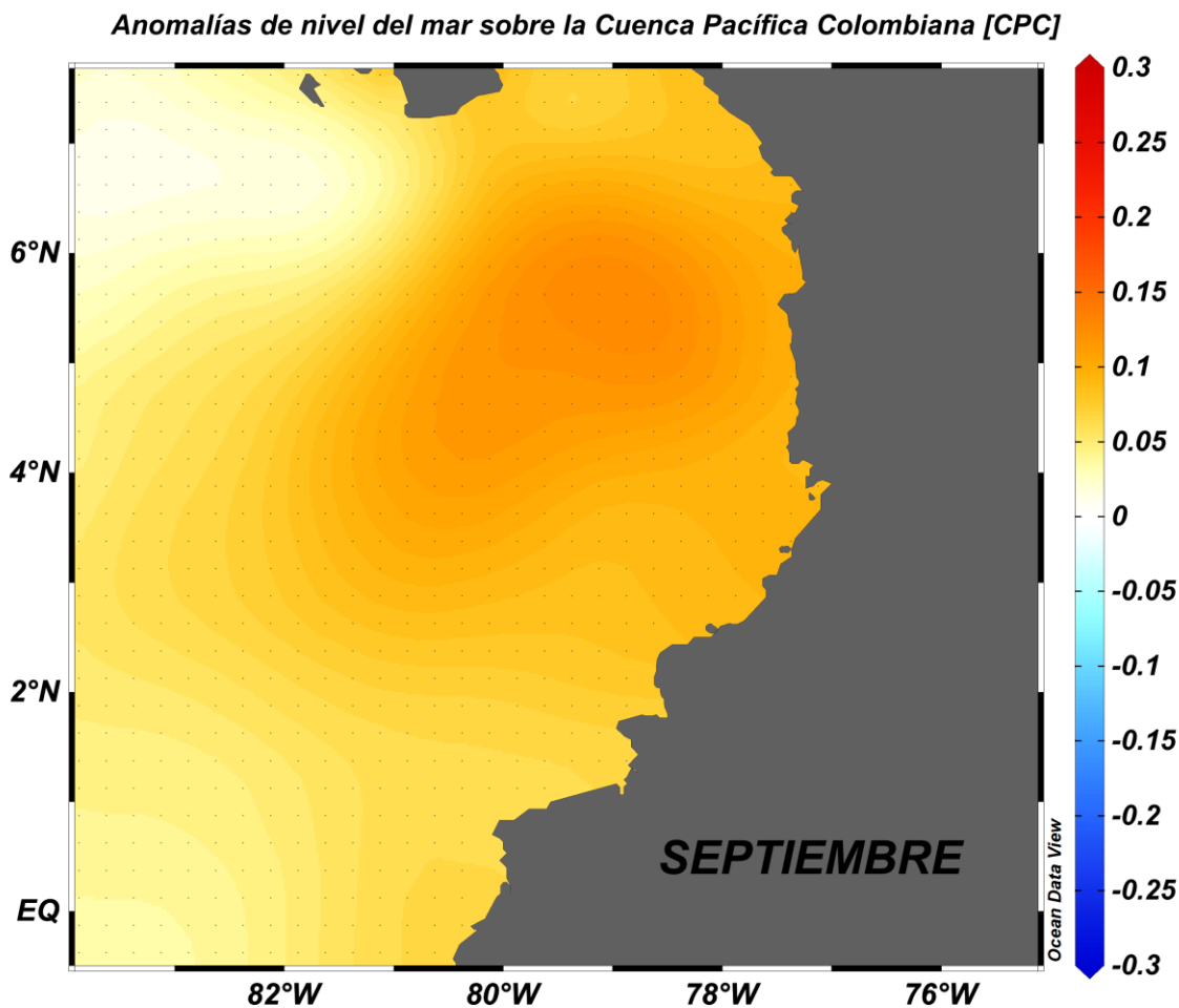
Figura 6. Anomalías de nivel del mar en la Cuenca Pacífica Colombiana (CPC) para el mes de septiembre de 2020 (Fuente: Copernicus Marine Service (CMEMS), Procesamiento: CCCP).
