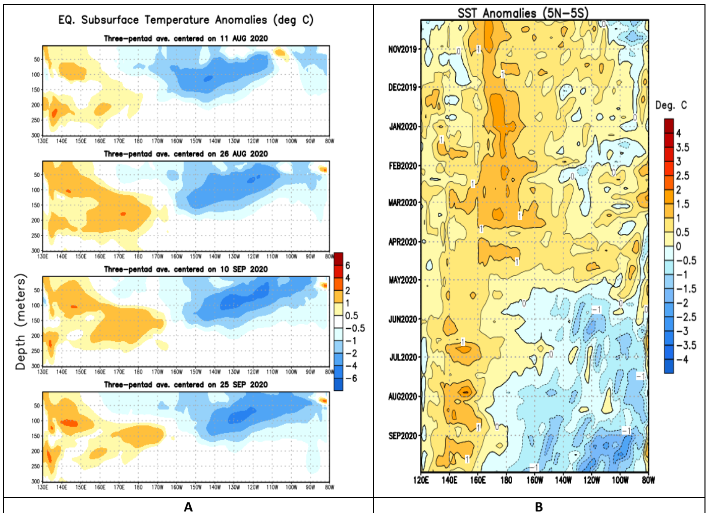
Figura 1. Evolución de las anomalías de temperatura subsuperficial (A) en el (OPE) y superficiales (B) entre latitudes 5^{\circ}\text{S} y 5^{\circ}\text{N} para el periodo comprendido entre el 11 de agosto al 25 de septiembre del 2020. La escala de colores representa la magnitud de las anomalías en ^{\circ}\text{C} . Fuente: Climate Prediction Center-NOAA.
