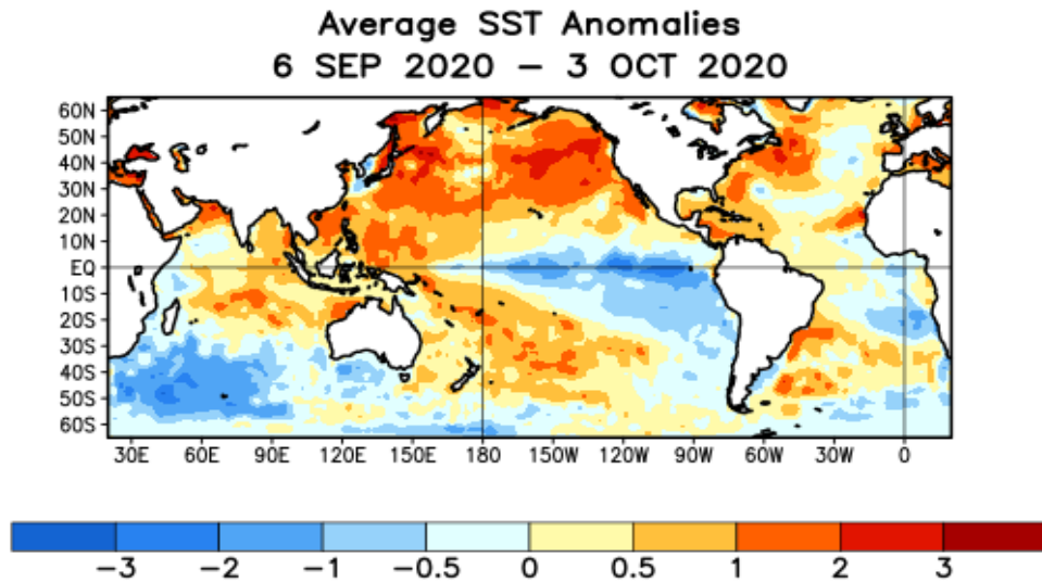
Figura 2. Anomalías de TSM en el Océano Pacífico Tropical para el periodo comprendido del 06 de septiembre al 03 de octubre de 2020. La escala de colores representa la magnitud en ^{\circ}\text{C} . Fuente: Climate Prediction Center – NOAA.
