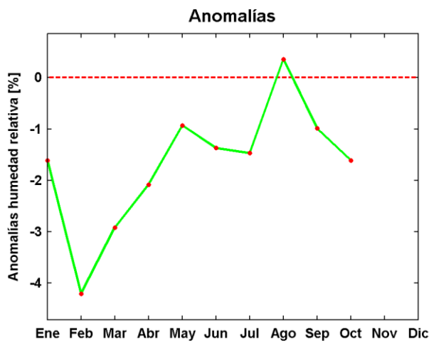
Figura 9. Serie de tiempo, histograma de frecuencia, anomalía y resumen estadístico mensual de la humedad relativa en Buenaventura.
