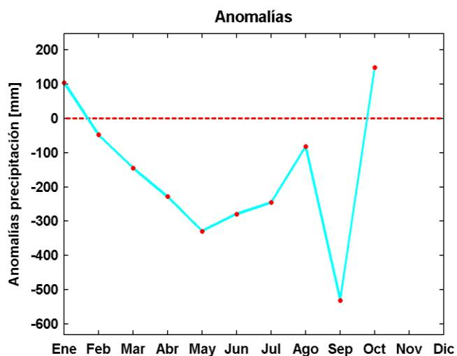
Figura 5. Serie de tiempo, histograma de frecuencia, anomalía y resumen estadístico mensual de la precipitación en Bahía Solano.
