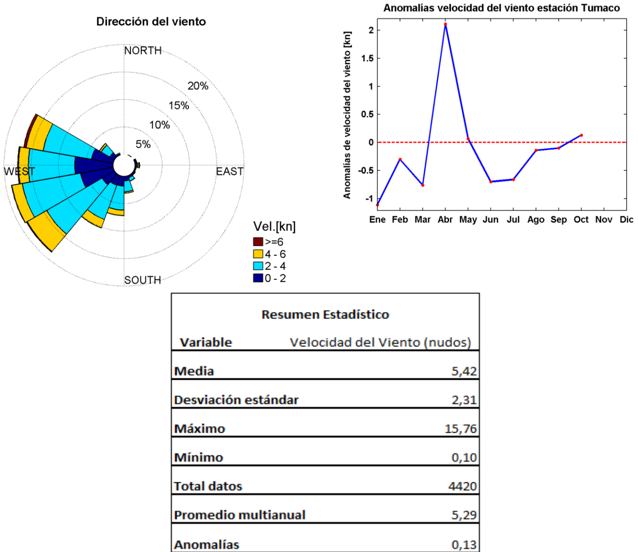
Figura 18. Distribución de frecuencia de la dirección, velocidad, anomalía velocidad y resumen estadístico del viento en Tumaco.
