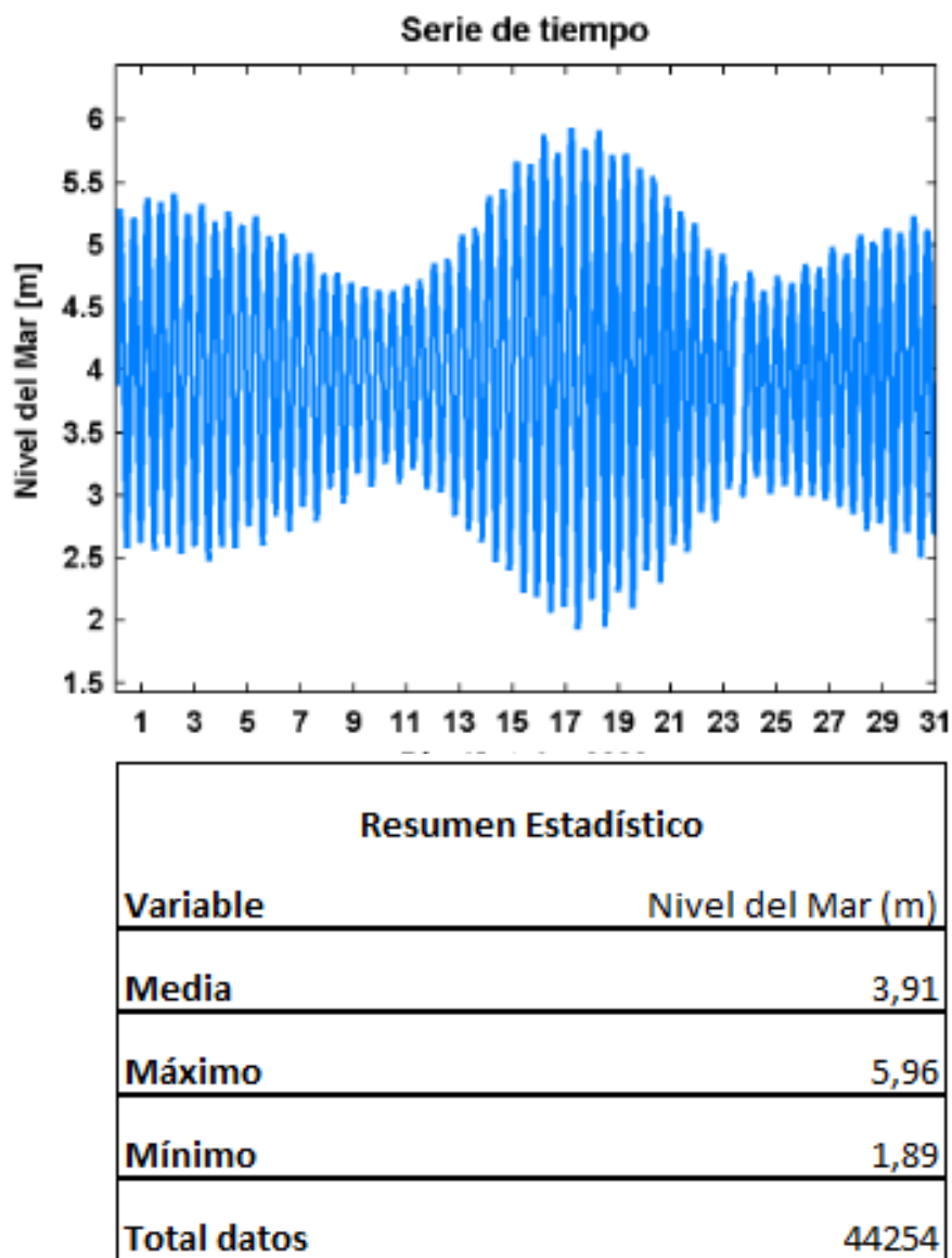
Figura 19. Serie de tiempo y resumen estadístico mensual del nivel del mar en Tumaco.
