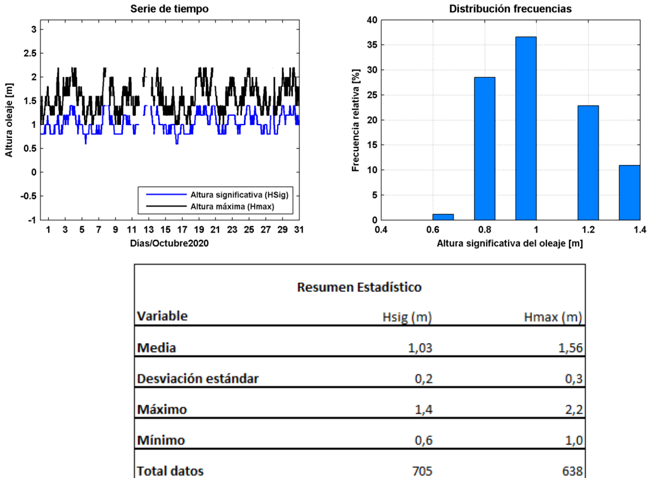
Figura 21. Serie de tiempo, histograma de frecuencia y resumen estadístico mensual de la altura significativa y máxima del oleaje, Tumaco.
