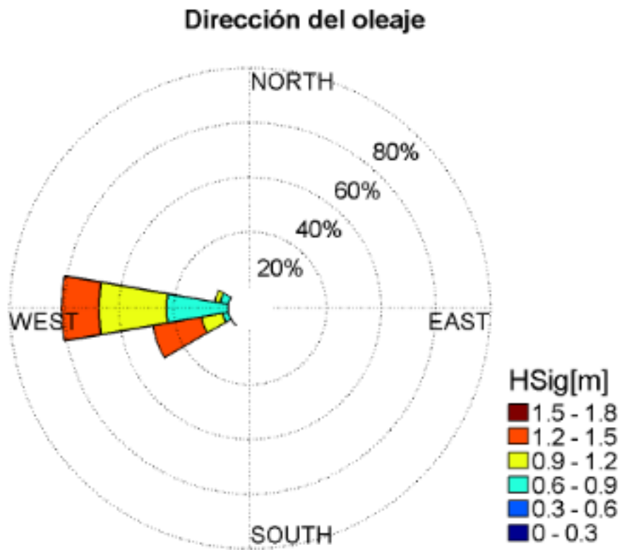
Figura 20. Distribución de frecuencia de la dirección del oleaje, Tumaco.
