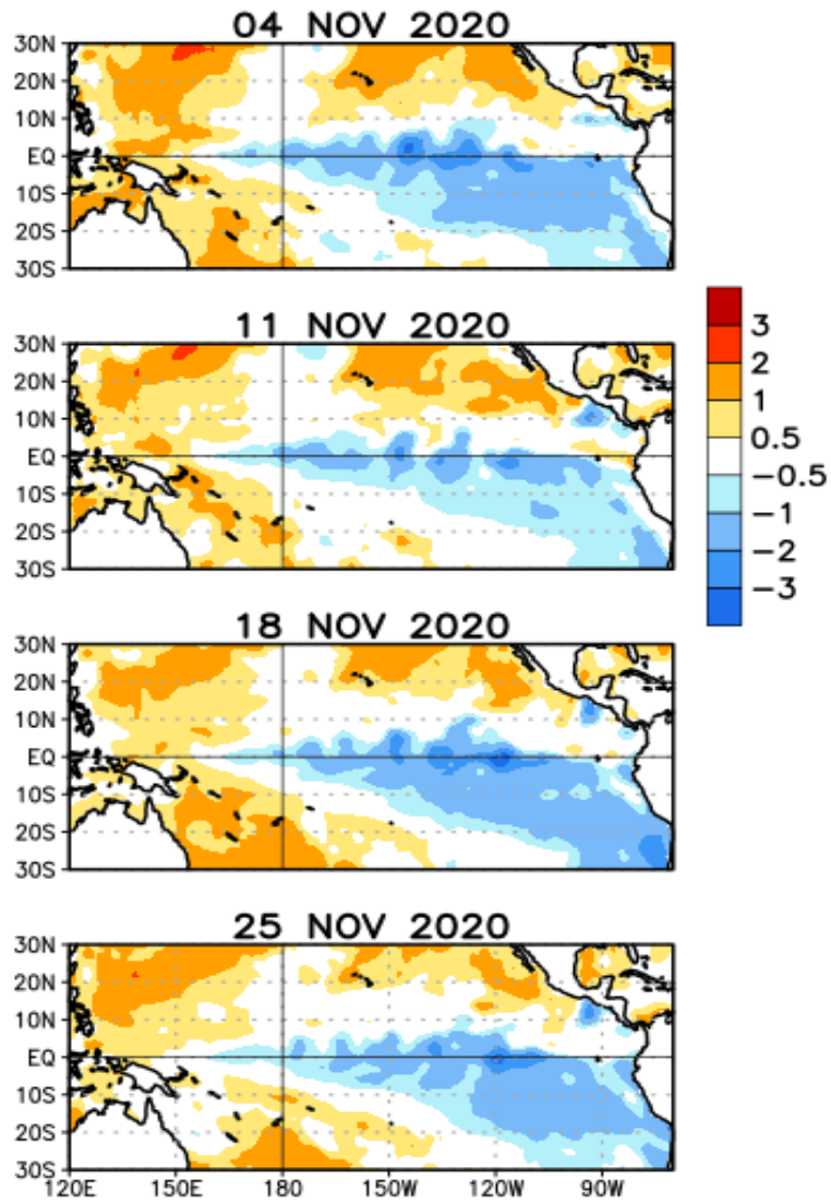
Figura 3. Anomalías semanales de TSM en el Océano Pacífico Tropical para el periodo comprendido del 04 al 25 de noviembre del 2020. Fuente: Climate Prediction Center-NOAA.
