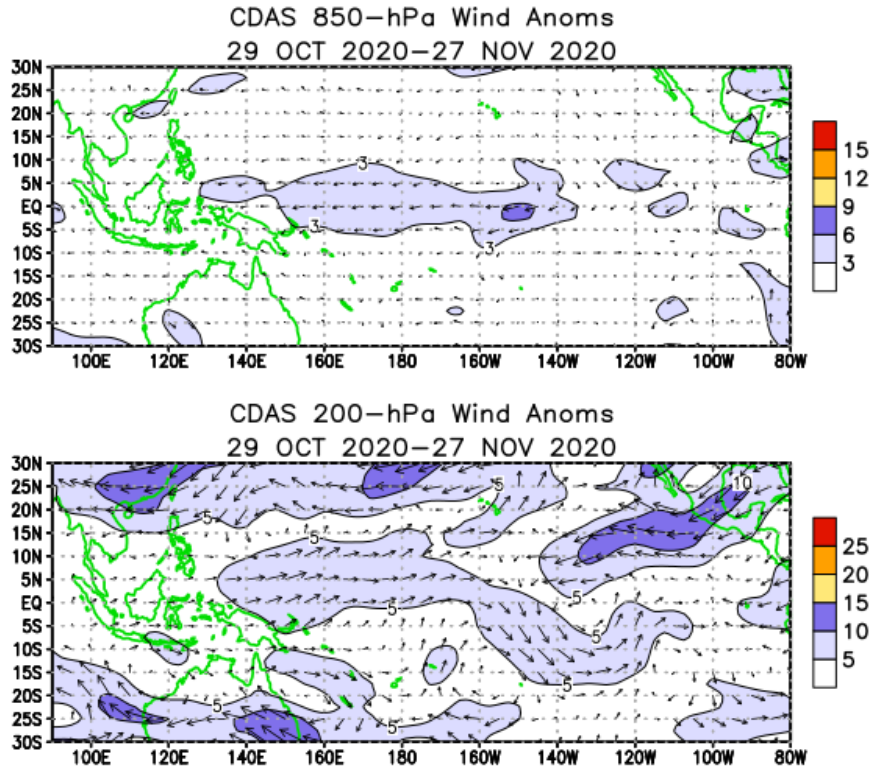
Figura 5. Anomalías campos de vientos sobre el Océano Pacífico Ecuatorial (OPE) para el periodo comprendido del 29 de octubre al 27 de noviembre de 2020. Fuente: Climate Prediction Center-NOAA.
