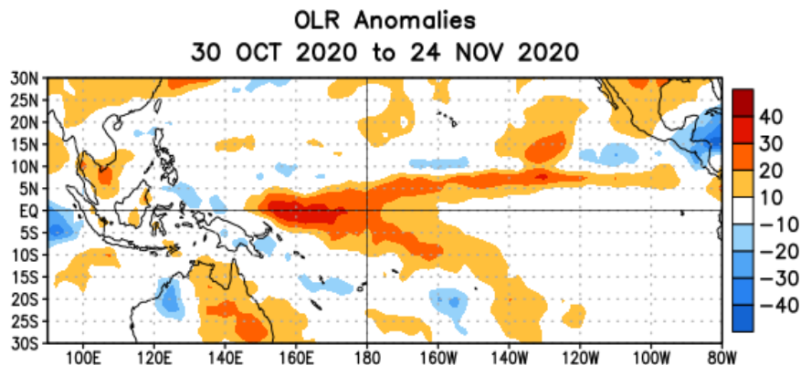
Figura 6. Anomalías Radiación de Onda Larga (OLR, por sus siglas en inglés) Para el periodo comprendido del 30 de octubre al 24 de noviembre del 2020. La escala de colores representa en W/m 2 . Fuente: Climate Prediction Center-NOAA.
