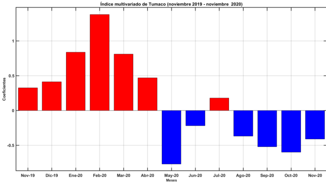
Figura 11. Comportamiento del Índice Multivariado de Tumaco (IMT) para el periodo comprendido entre noviembre del 2019 y noviembre del 2020. Fuente: CCCP.
