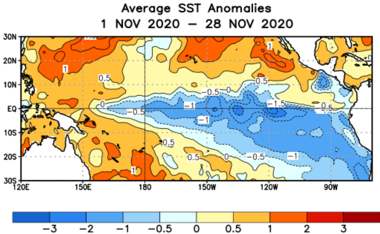
Figura 2. Anomalías de TSM en el Océano Pacífico Tropical para el periodo comprendido del 01 al 28 de noviembre de 2020. La escala de colores representa la magnitud en ^{\circ}\text{C} . Fuente: Climate Prediction Center – NOAA.
