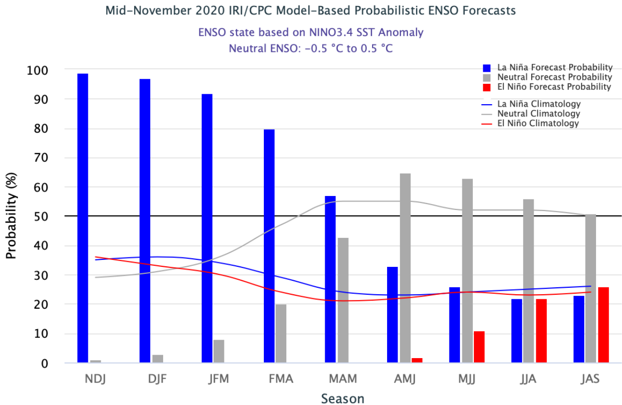
Figura 12. Predicción modelos estadísticos y dinámicos de condiciones IRI ENOS 19 de noviembre del 2020. (Fuente: IRI/CPC).
