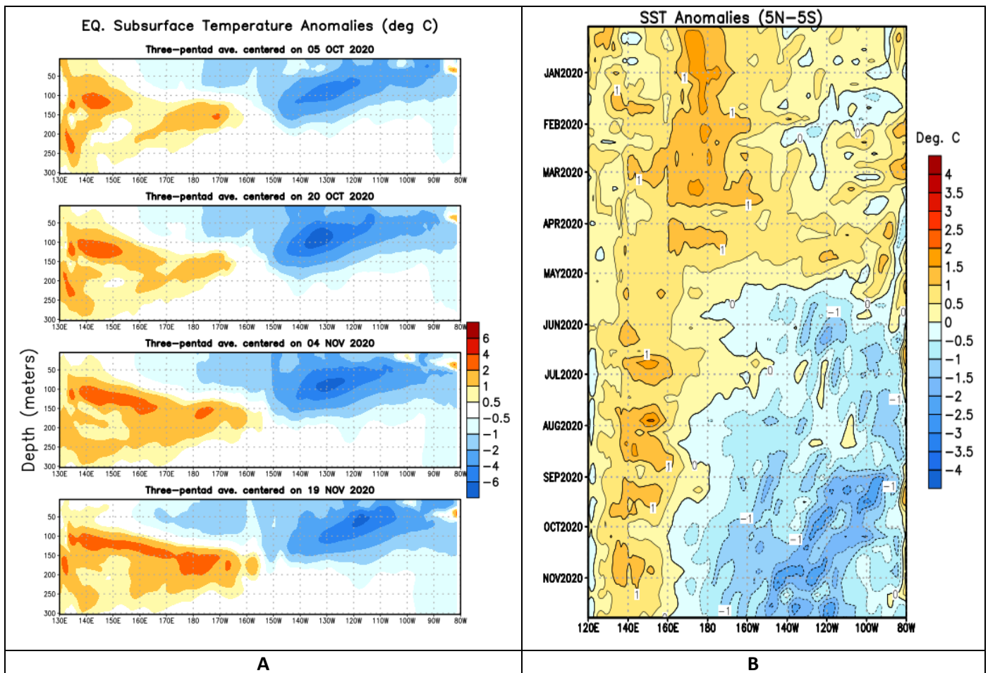
Figura 1. Evolución de las anomalías de temperatura subsuperficial (A) en el (OPE) y superficiales (B) entre latitudes 5^{\circ}\text{S} y 5^{\circ}\text{N} para el periodo comprendido entre el 05 de octubre al 19 de noviembre del 2020. La escala de colores representa la magnitud de las anomalías en ^{\circ}\text{C} . Fuente: Climate Prediction Center-NOAA.
