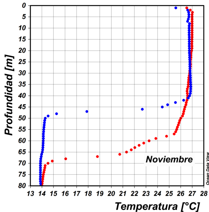
Figura 10. Perfil de temperatura para el mes de noviembre del 2020 registrado en la estación costera fija de Tumaco.
