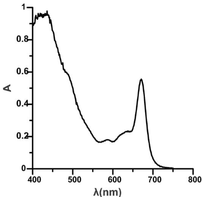
FIGURA 5. Espectro de absorción normalizado (A, adimensional) de Gymnodinium sp. de las muestras tomadas en El Laguito.
