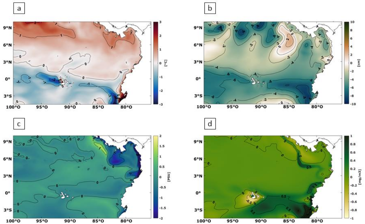
Figura 11. Distribuciones espaciales esperadas en el periodo comprendido entre el 1-14 de octubre para: a) TSM en °C, b) Nivel del mar en cm, c) Salinidad en PSU y d) Clorofila-a en mg/m3. Fuente: COPERNICUS Marine Service. Elaboración: CCCP.
