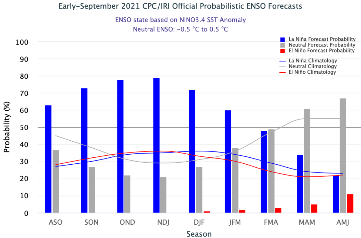
Figura 12. Pronósticos probabilísticos de las condiciones ENOS actualizados el 09 de septiembre del 2021. Fuente: Research Institute for Climate and Society (IRI) .
