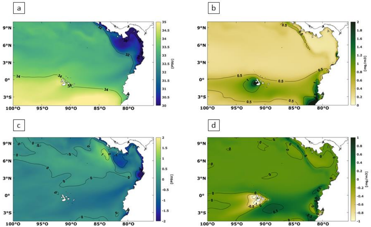
Figura 7. Distribuciones espaciales mensuales de a) Salinidad y b) Clorofila-a en mg/m 3 . Distribuciones espaciales mensuales de las anomalías de c) Salinidad y d) Clorofila-a en mg/m 3 . Fuente: COPERNICUS Marine Service. Elaboración: CCCP.
