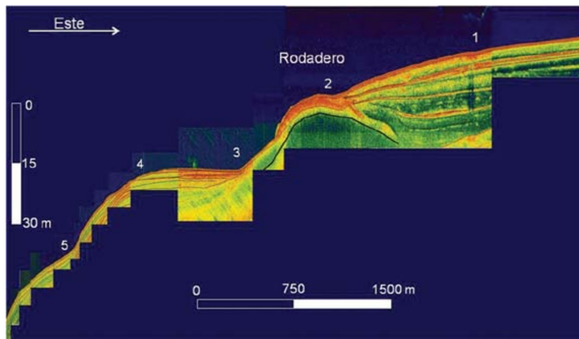
Figura 10. Perfil F en la ensenada de Gaira, frente a El Rodadero. Secuencia sedimentaria finamente estratificada (1 y 3), interrumpida hacia la mitad del perfil por un afloramiento rocoso (2). En el recuadro puede observarse el acuñamiento de los estratos contra la roca. A 75 m de profundidad (4) empieza a hacerse más fuerte la pendiente y se extiende así hasta el final del perfil, con un ligero quiebre a 120 m (5).
