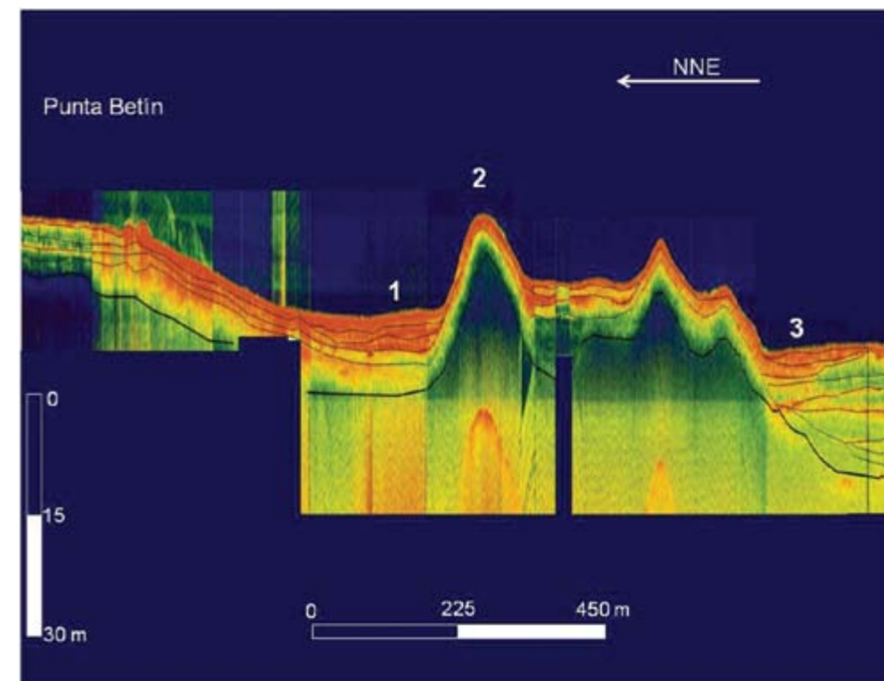
Figura 8. Perfil meridional (NNE-SSW) hecho entre la Bahía de Santa Marta, sedimentos estratificados (1) sistema rocoso (2), contacto con sedimentos blandos (3) la línea café y blanca muestra la máxima penetración.
