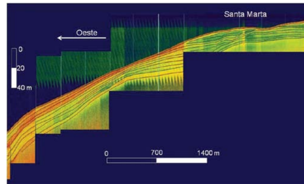
Figura 9. Perfil E frente a Santa Marta, desde el centro de la bahía hacia el oeste. Relieve muy regular con estratificación uniforme que alcanza hasta 35 m en el extremo W. Algunas ondulaciones y acuñamientos y un aparente cambio de material del fondo registrado a partir de los 90 m de profundidad (la imagen tiene exageración vertical).
