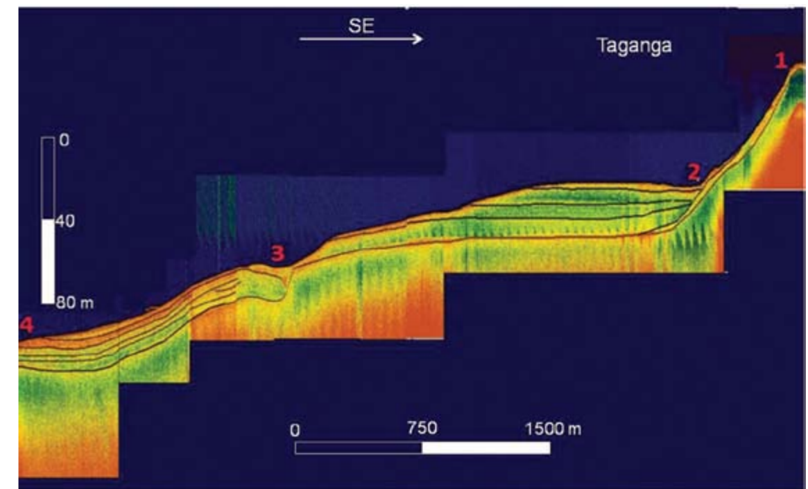
Figura 6. Perfil B frente a Taganga. A 113 m de profundidad la estratificación uniforme se acuña, sobre lo que parece ser una estructura asociada al sistema rocoso de La Sierra. (1), vertiente cubierta por sedimentos blandos (2), acuñamiento de la estratificación sobre la vertiente; (3) posible estructura geológica, (4) estratificación que sigue el relieve inicial del fondo, sobre rocas de la SNSM (La imagen está exagerada en la vertical).
