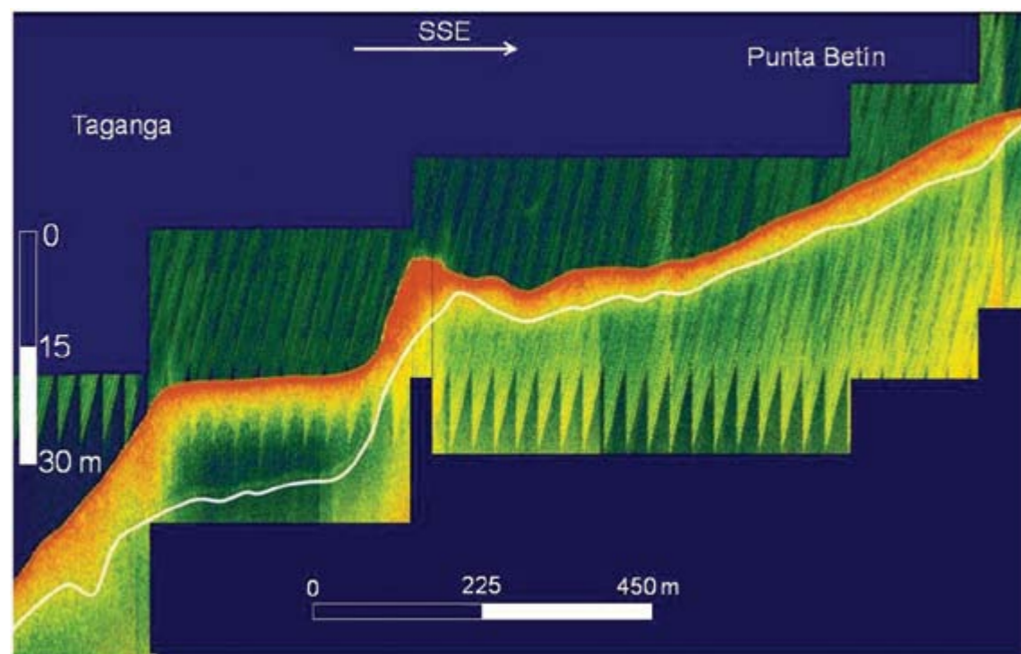
Figura 7. Perfil meridional entre Taganga y Punta Betín (C), con un fondo duro que permitió poca penetración. A 85 m se registra un escalón o quiebre en la pendiente que podría estar asociado con una estructura geológica.
