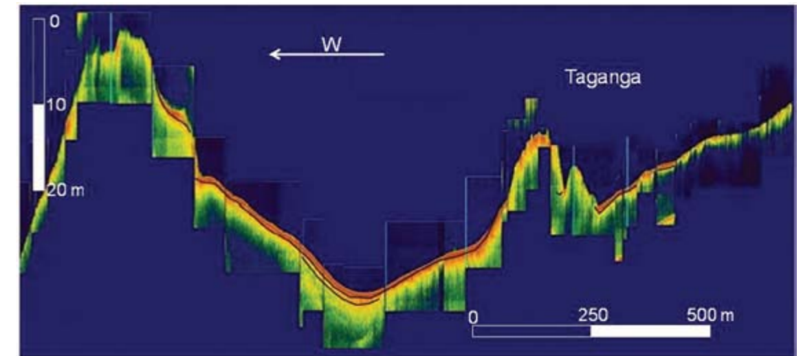
Figura 5. El fondo dentro de la Bahía de Taganga (perfil A), formaciones montañosas de estratos muy duros, la línea café muestra la máxima penetración.
