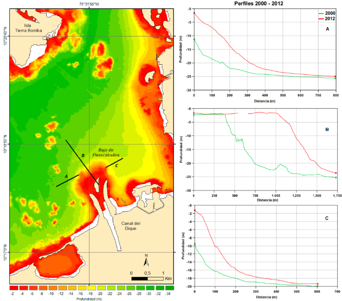
Figura 4. Perfiles de profundidad en las batimetrías de los años 2000 y 2012.
