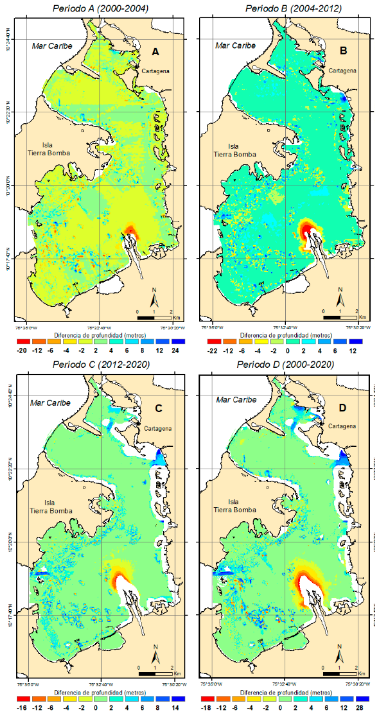
Figura 3. Vista 2D de la diferencia entre las batimetrías de la bahía de Cartagena en cuatro periodos de los últimos 20 años.
