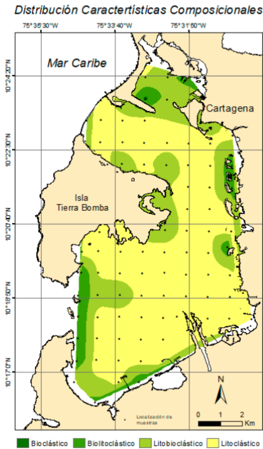
Figura 6. Visualización de la distribución de las características composicionales de los sedimentos superficiales de la bahía de Cartagena.
