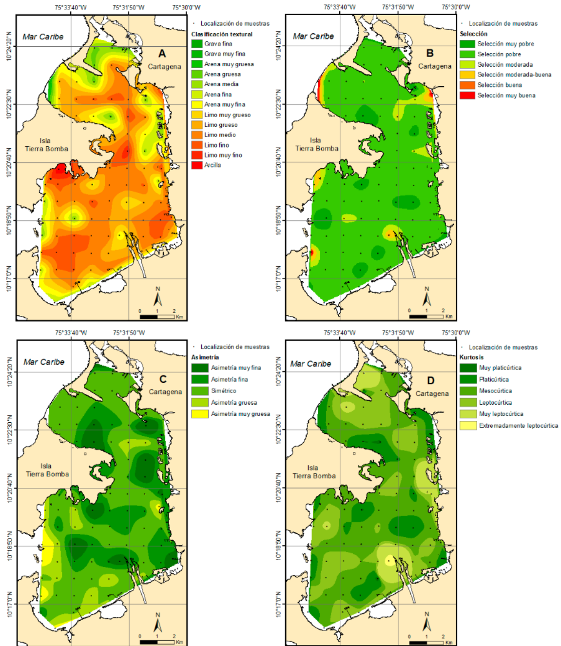
Figura 5. Visualización de la distribución de las características texturales de los sedimentos superficiales de la bahía de Cartagena.
