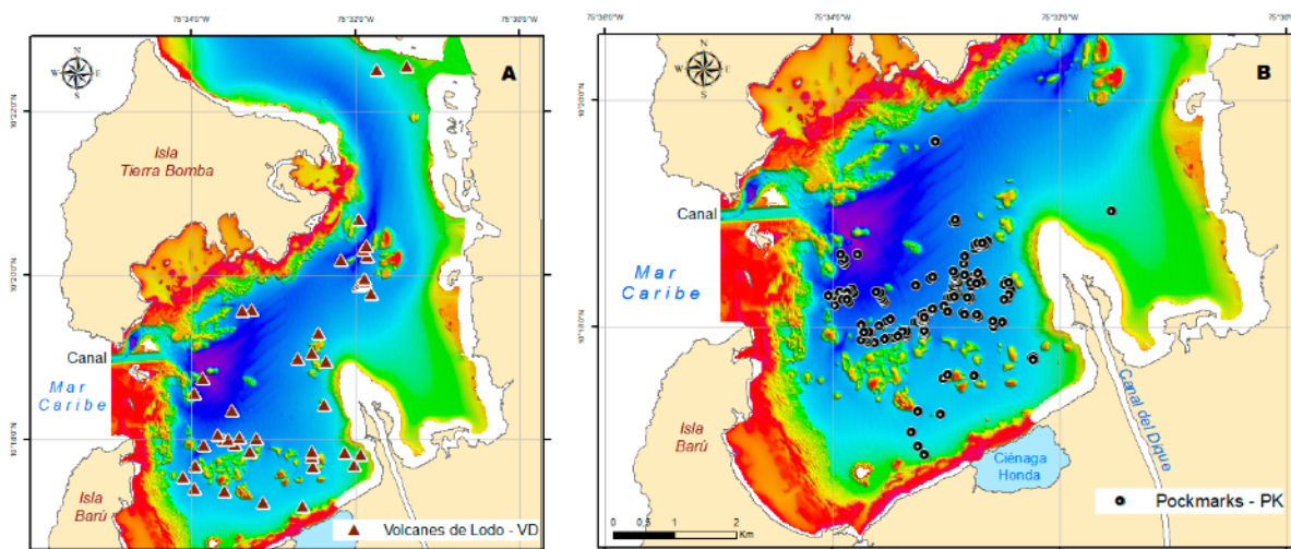
Figura 7. Localización de volcanes de lodo (VD) y pockmarks (PK) en la bahía de Cartagena.
