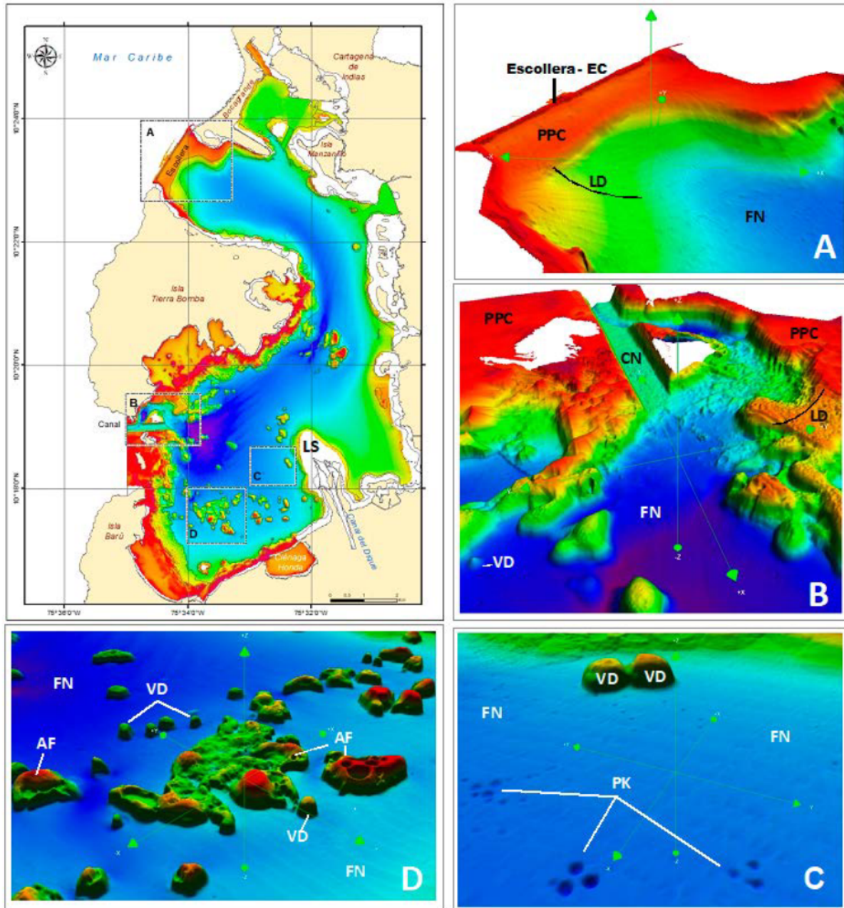
Figura 2. Unidades geomorfológicas: plano continental (PPC), ladera (LD), fondo (FN), arrecife (AF), volcán de lodo (VD), pockmarks (PK), canal (CN), lóbulo de sedimento (LS), escollera (EC).
