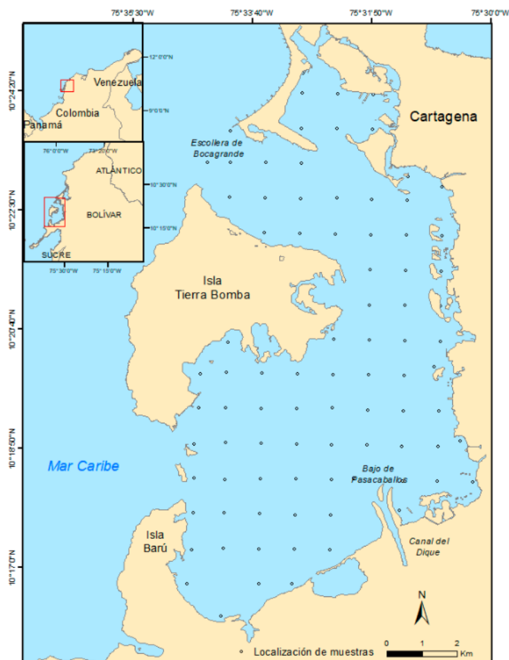
Figura 1. Ubicación del área de estudio y los puntos de muestreo (puntos negros).
