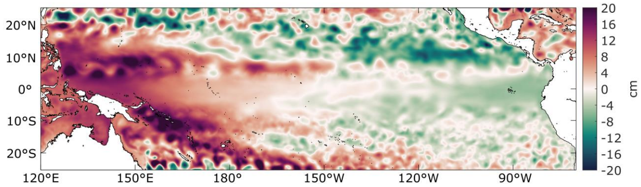
Anomalía Temperatura Superficial del Mar (ATSM)
