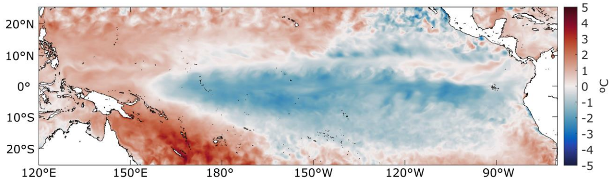
Figura 1. Distribución espacial mensual de variables océano-atmosféricas en el Océano Pacífico Tropical.
