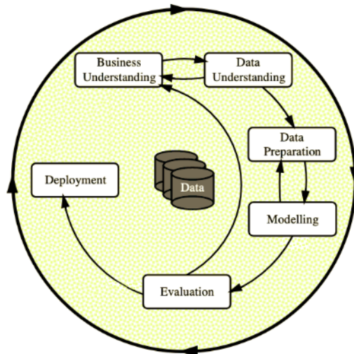
Figura 2. Fases del Modelo del Proceso CRISP-DM (Wirth y Hipp, 2000).
