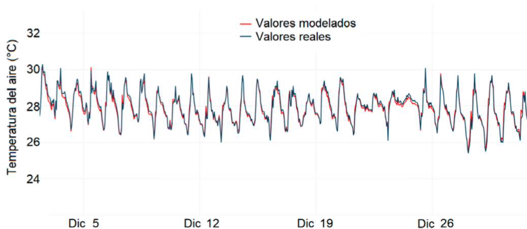
Figura 15. Modelado de datos en el último mes de 2021 con el modelo de RNN para la serie de temperatura del aire.
