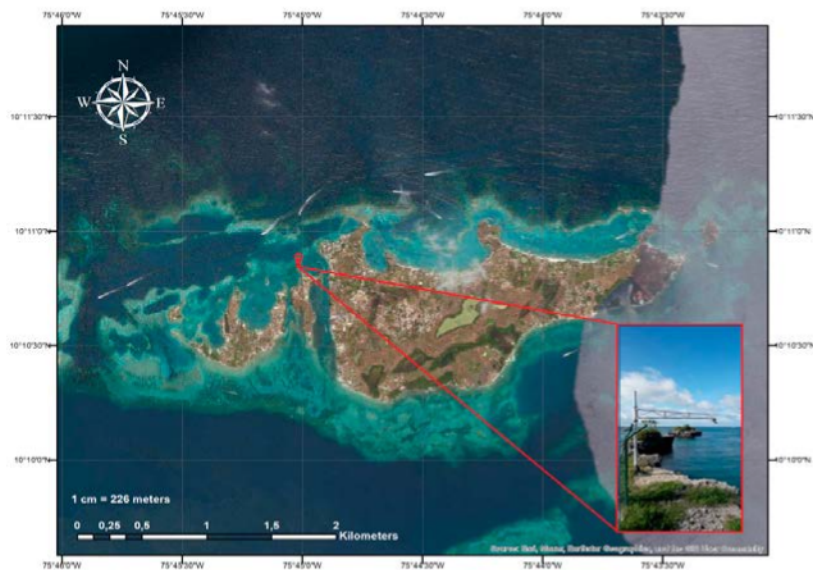
Figura 4. Ubicación de la estación meteorológica automática en Isla Naval (Islas del Rosario, Caribe colombiano) perteneciente a RedMpomm.
