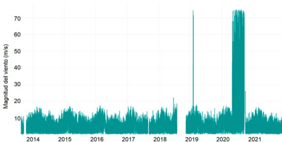
Figura 6. Serie de tiempo original para la magnitud del viento.
