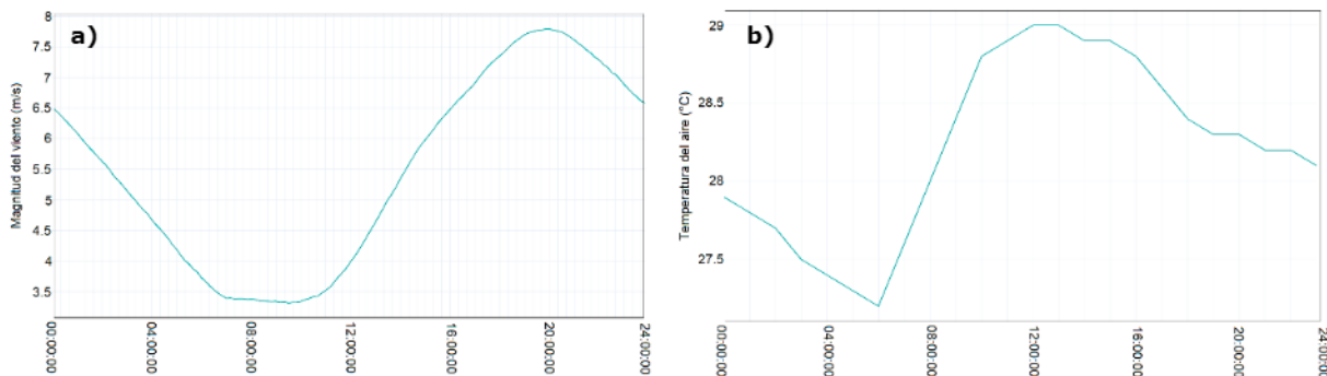
Figura 10. Promedio diario de la magnitud del viento (a) y la temperatura del aire (b).
