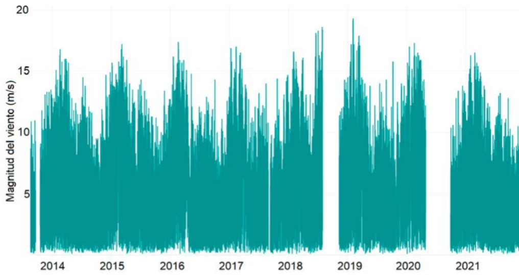
Figura 7. Serie de tiempo de la magnitud del viento (m/s) después del proceso de limpieza.
