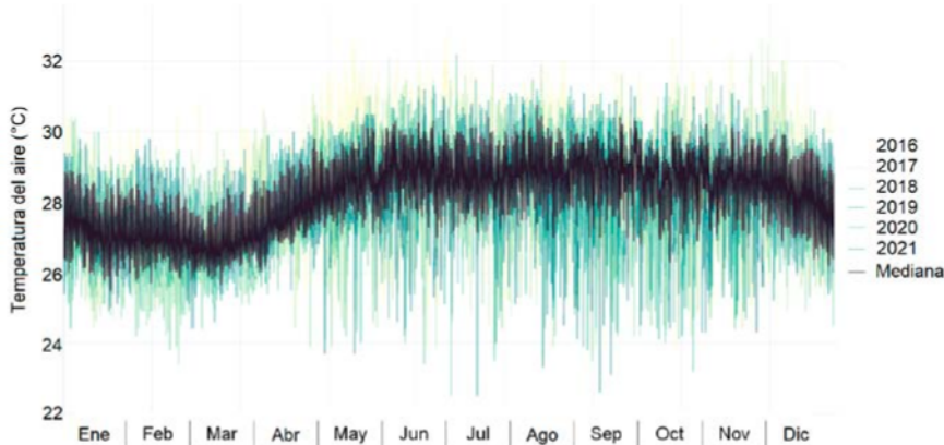
Figura 11. Serie superpuesta de la temperatura del aire (°C), de 2016 a 2021. Incluye la mediana de todos los años.
