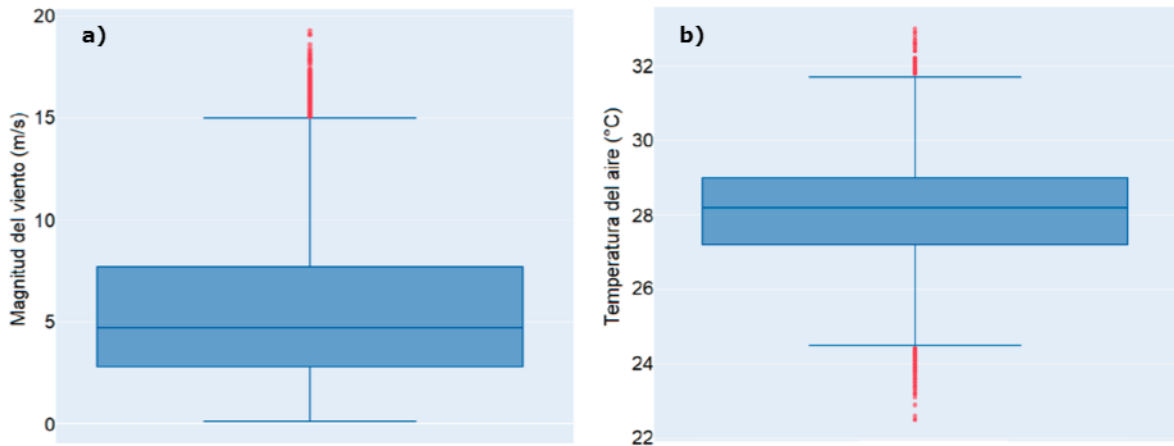
Figura 9. Diagrama de caja y bigotes para la magnitud del viento (a) y la temperatura del aire (b).
