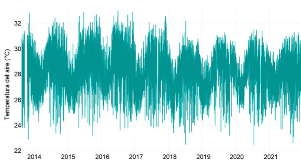
Figura 8. Serie de tiempo de la temperatura del aire (°C) después del proceso de limpieza.
