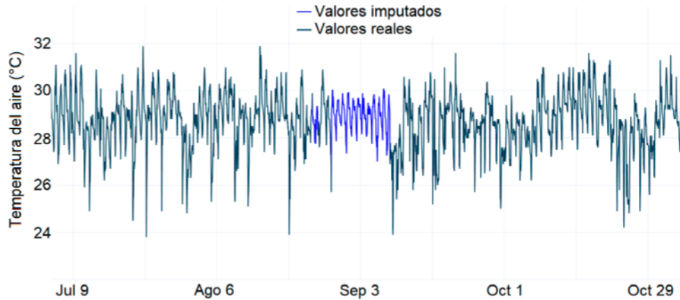
Figura 13. Serie reconstruida de temperatura del aire, desde agosto a septiembre de 2017.
