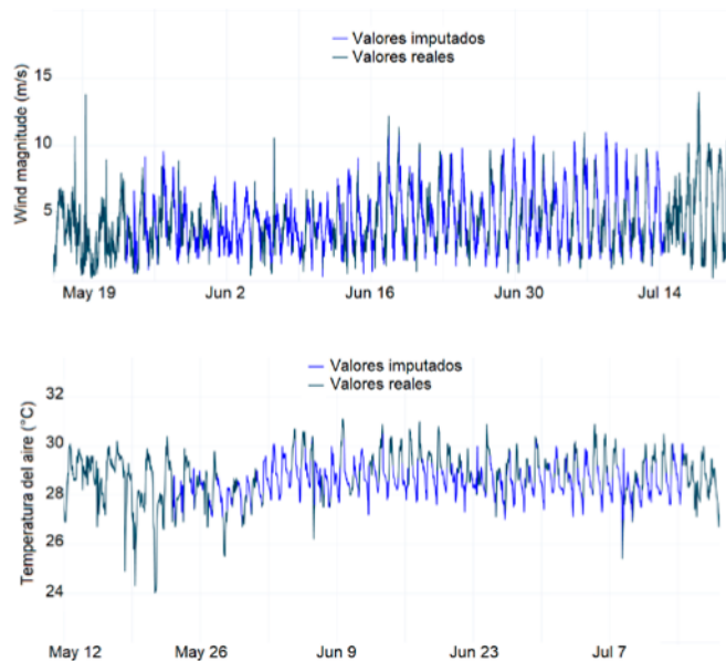
Figura 12. Valores imputados y reales en 2019 para la magnitud del viento (a) y la temperatura del aire (b).
