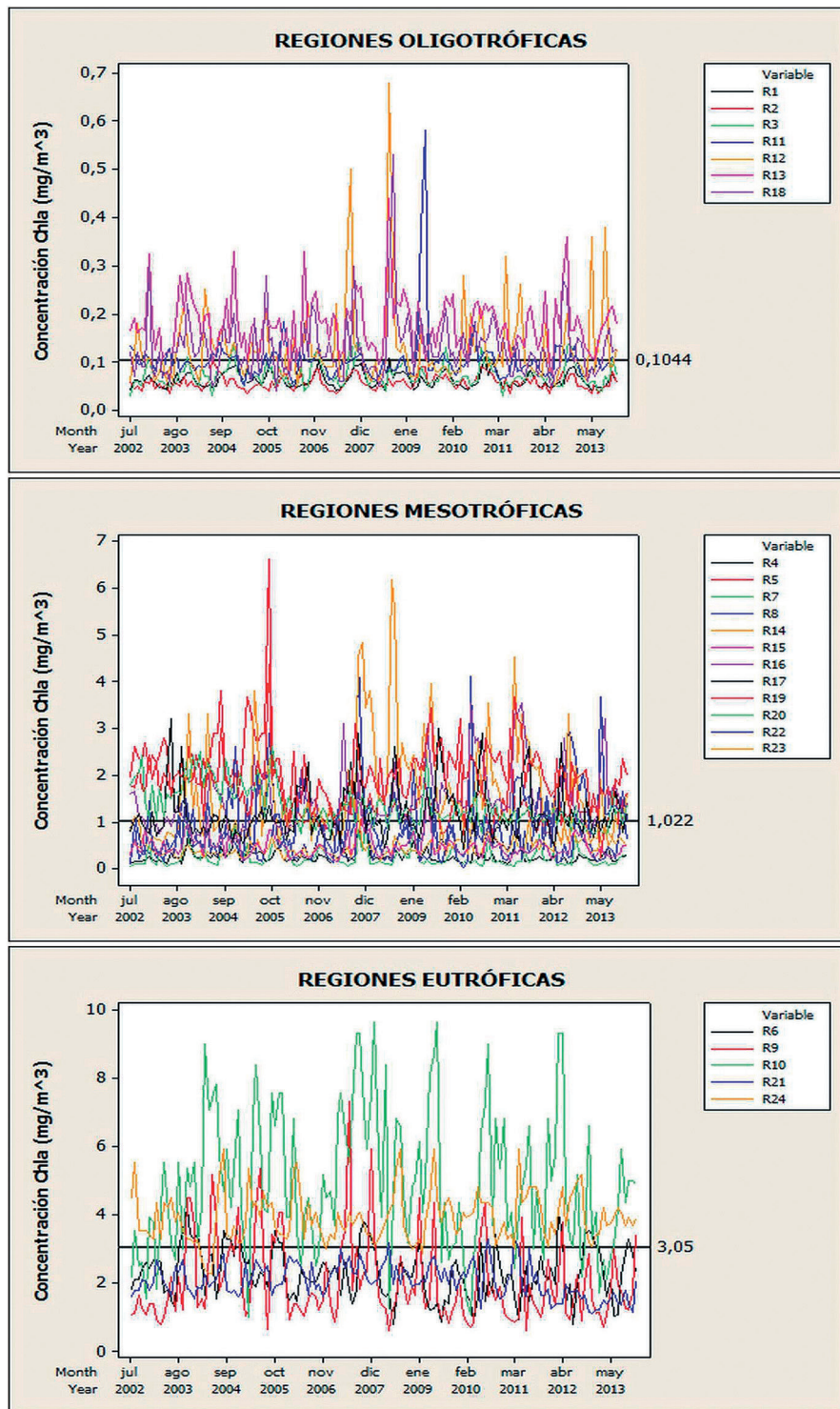
Figura 4. Series de tiempo para las regiones oligotróficas, mesotróficas y eutróficas en la isla de Santo Domingo. Serie de tiempo mensual junio 2002-noviembre 2013 de las 30 estaciones. La línea continua negra indica el valor promedio.
