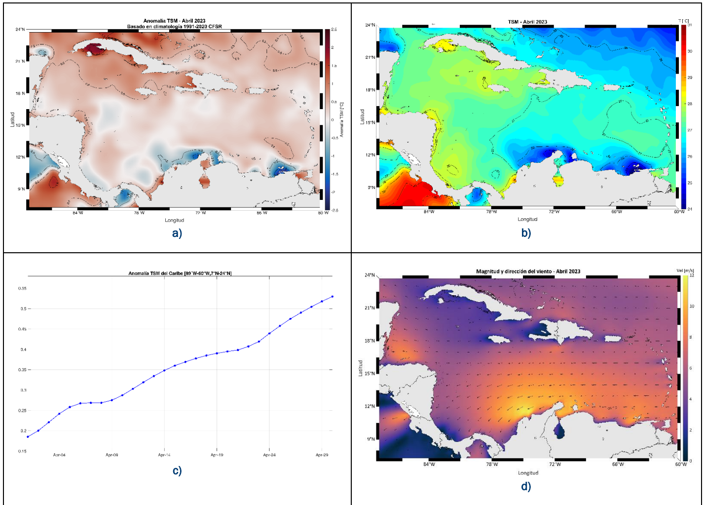
Figura 3 Valores promedio (a), anomalía (b), evolución diaria de la TSM (c), vientos superficiales (d), observados durante el mes de abril de 2023 en el mar Caribe. Fuente: STAR Satellite Rainfall Estimates - Hydro-Estimator- NOAA (Scofield & Kuligowski, 2003) y Modelo CFSR – NCEP (Saha et al., 2014).
