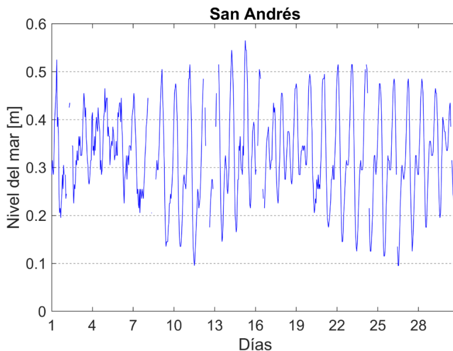
Figura 27 Comportamiento mensual del nivel del mar en la zona Insular de la Cuenca Caribe colombiana.
