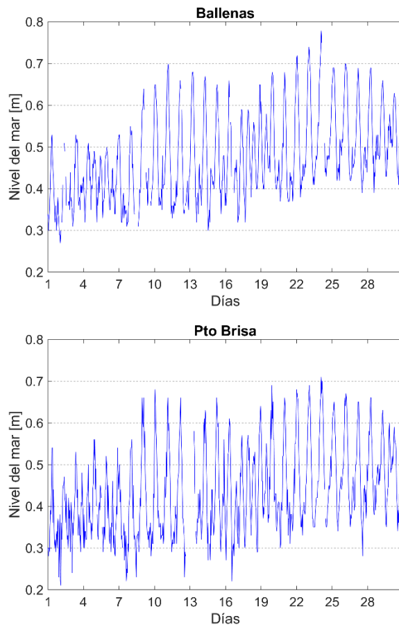
Figura 9 Comportamiento mensual del nivel del mar en la zona norte de la Cuenca Caribe colombiana.
