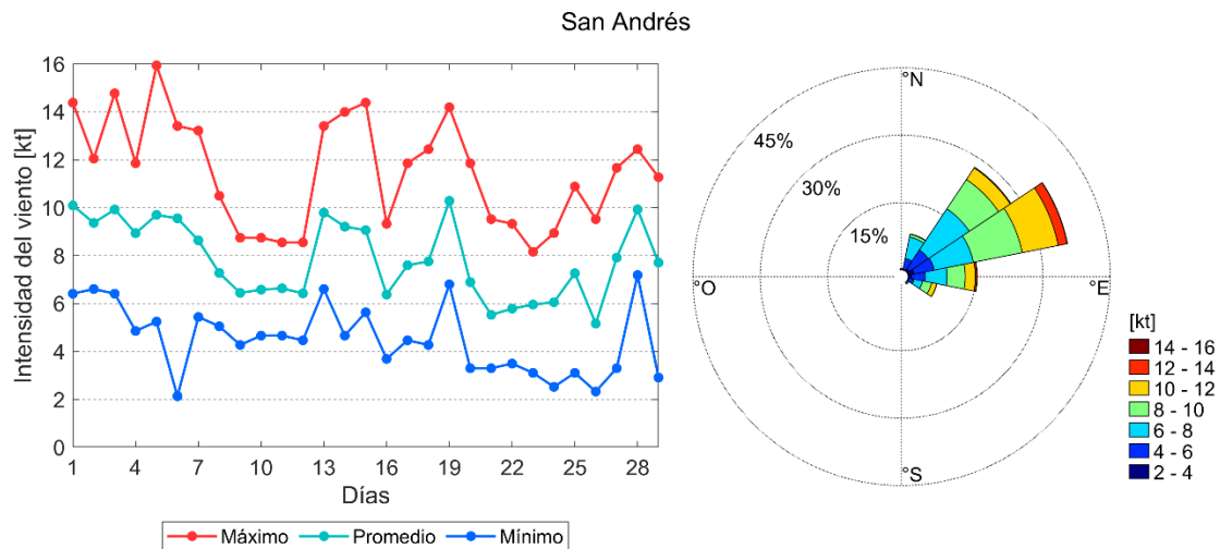
Figura 25 Comportamiento mensual de los vientos superficiales en la zona Insular de la Cuenca Caribe colombiana.
