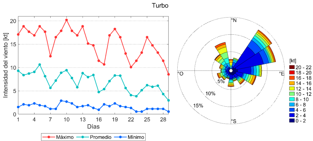
Figura 19 Comportamiento mensual de los vientos superficiales en la zona sur de la Cuenca Caribe colombiana.
