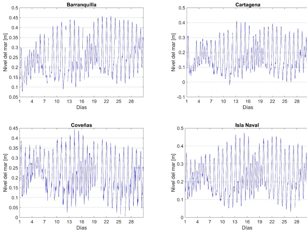
Figura 15 Comportamiento mensual del nivel del mar en la zona centro de la Cuenca Caribe colombiana.
