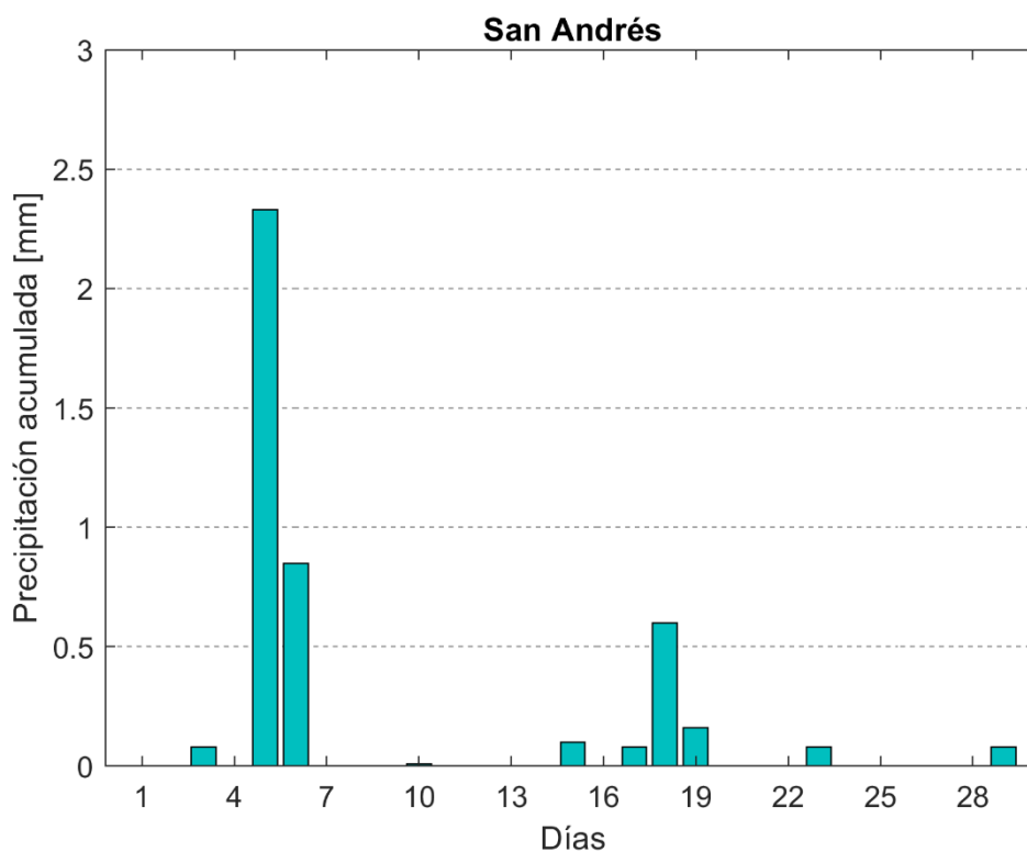
Figura 26 Comportamiento mensual de precipitación en la zona Insular de la Cuenca Caribe colombiana.
