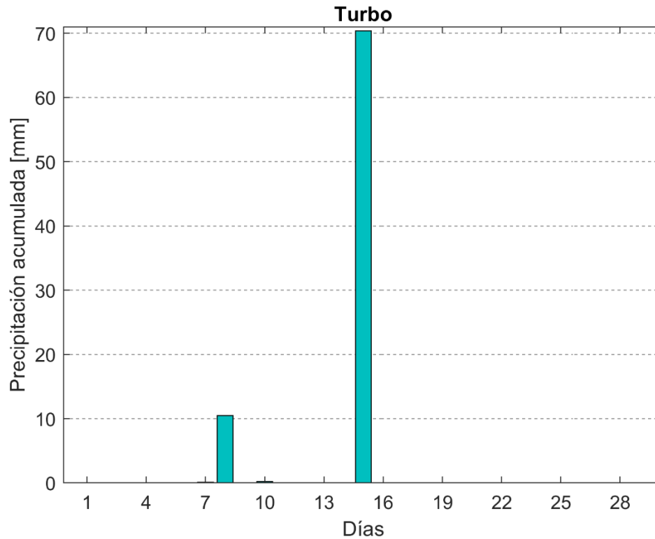
Figura 20 Comportamiento mensual de precipitación en la zona sur de la Cuenca Caribe colombiana.
