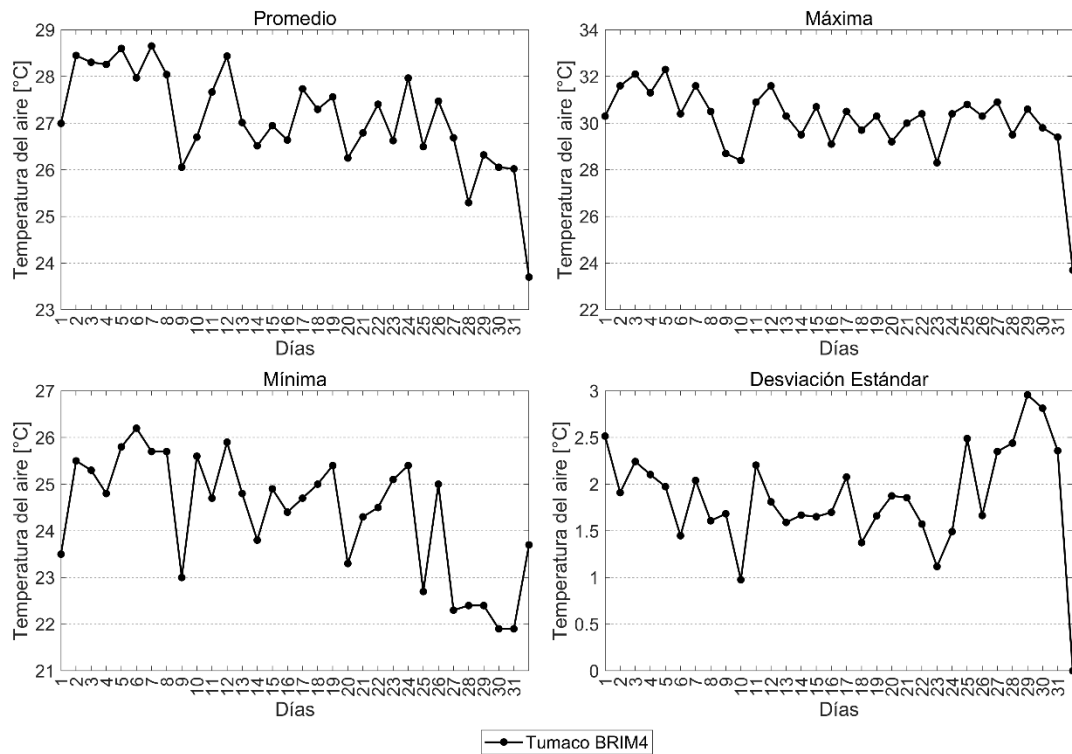
Figura 12. Comportamiento mensual de la temperatura del aire en la zona sur de la CPC.
