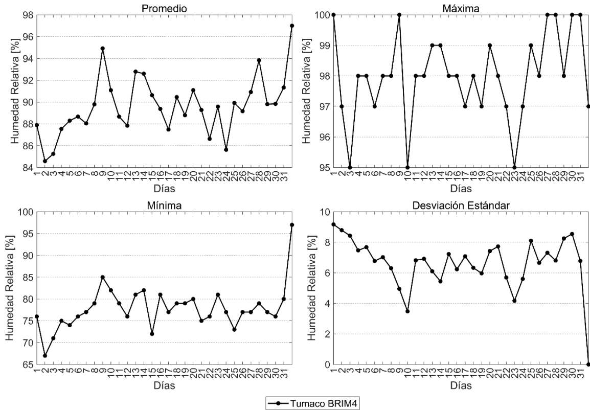
Figura 15. Comportamiento mensual de la humedad relativa en la zona sur de la CPC.
