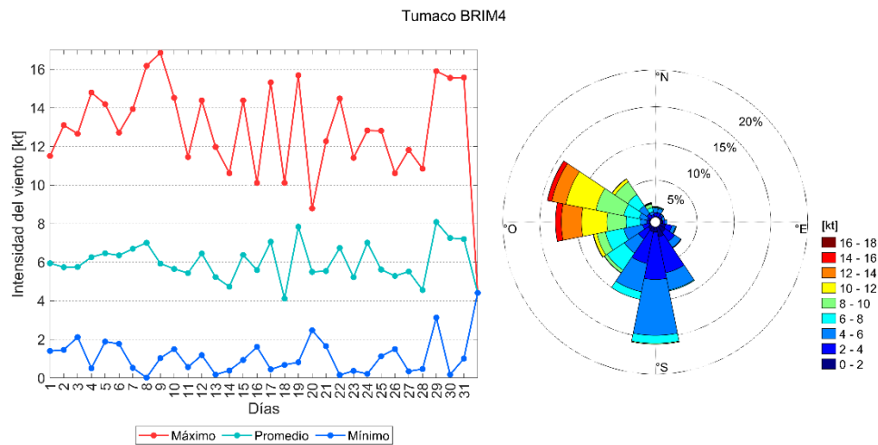
Figura 14. Comportamiento mensual del régimen de vientos superficiales en la zona sur de la CPC.
