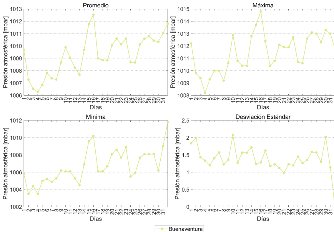
Figura 7. Comportamiento mensual de la presión atmosférica en la zona centro de la CPC.
