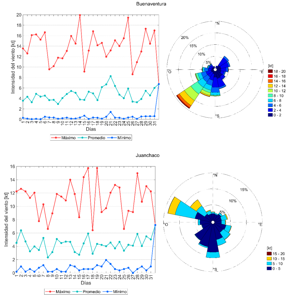
Figura 8. Comportamiento mensual del régimen de vientos superficiales en la zona centro de la CPC.
