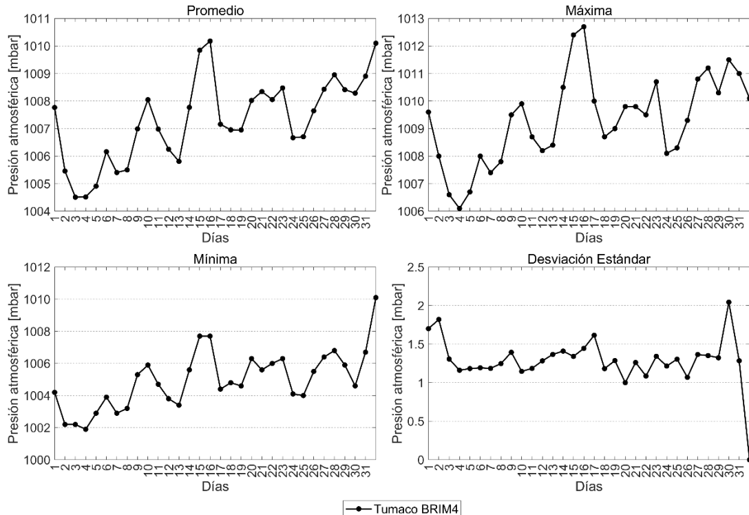
Figura 13. Comportamiento mensual de la presión atmosférica en la zona sur de la CPC
