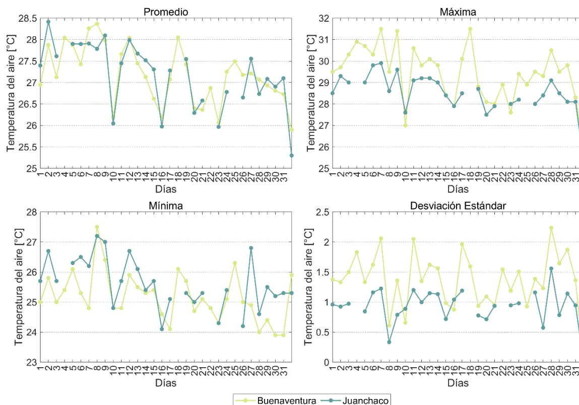
Figura 6. Comportamiento mensual de la temperatura del aire en la zona centro de la CPC.
