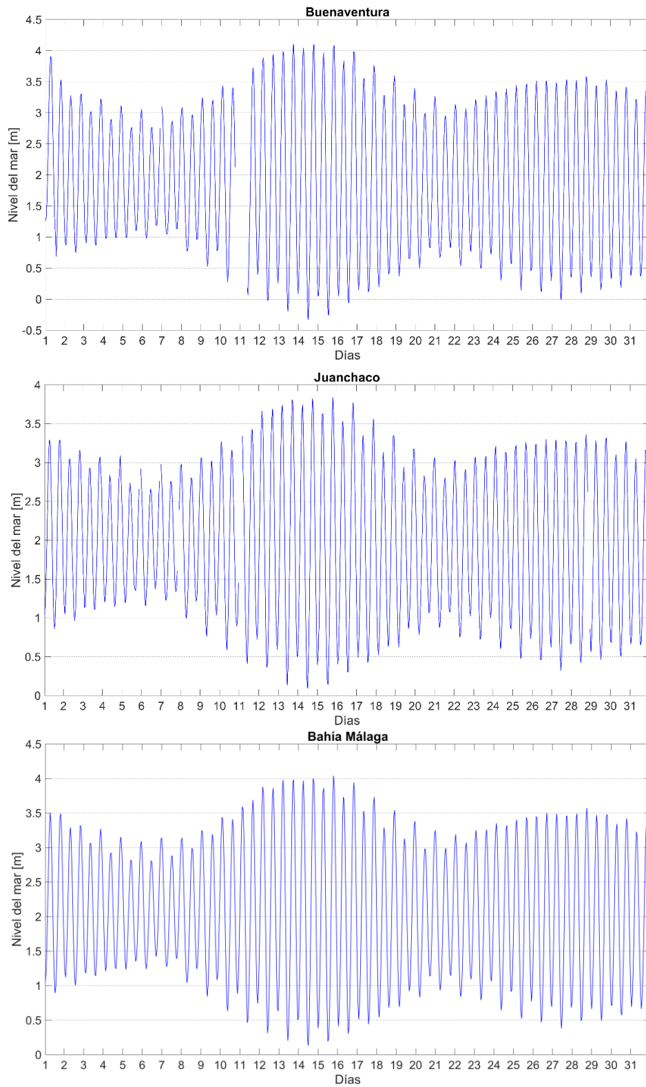
Figura 10. Comportamiento mensual del nivel del mar en la zona centro de la CPC.
