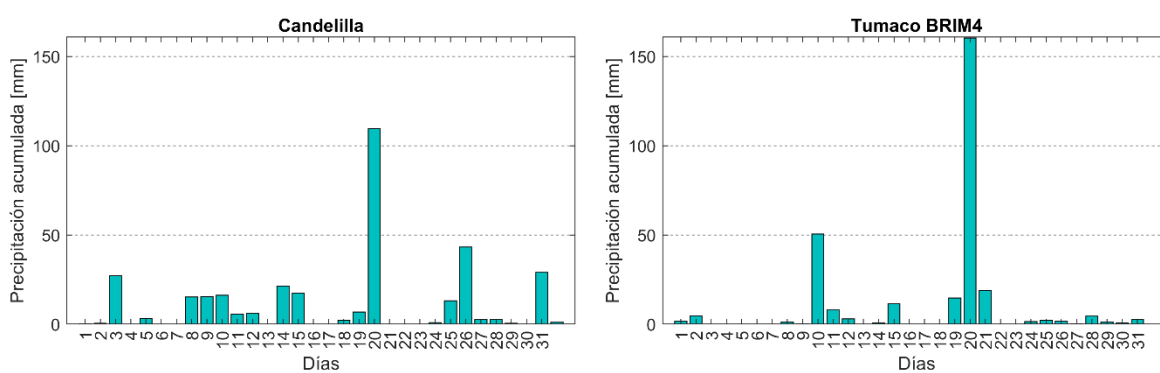
Figura 15. Comportamiento mensual de la precipitación acumulada en la zona sur de la CPC.
