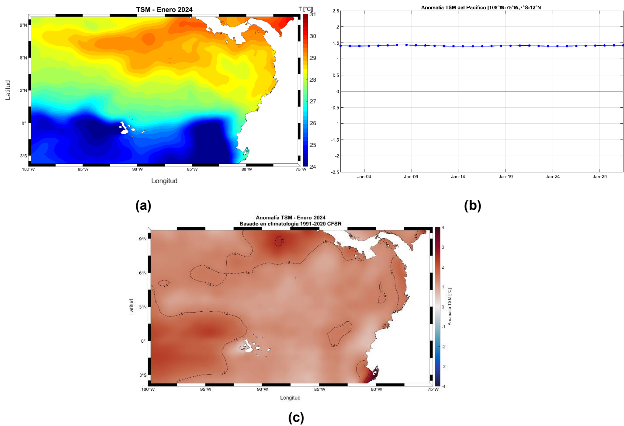
Figura 5. Temperatura superficial del mar en el Pacifico colombiano. (a) Promedio mensual de TSM; (b) anomalías de TSM (c) evolución diaria de TSM para enero de 2024. (Tomado de Climate Forecast System Reanalysis (CFSR)).
