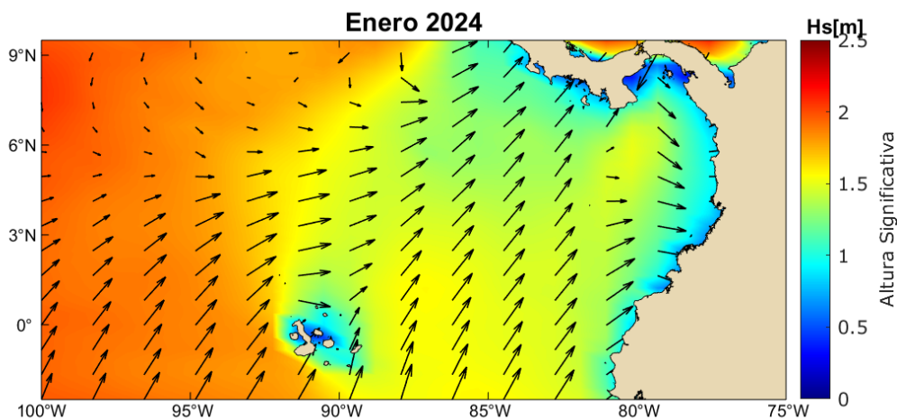
Figura 3. Distribución espacial de oleaje en el Pacífico colombiano durante enero 2024. (Tomado de Copernicus Marine Service, 2023).
