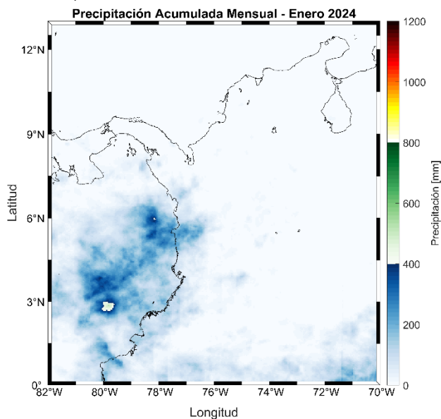
Figura 4. Distribución espacial de la precipitación acumulada mensual en el Pacífico colombiano durante enero 2024. (Procesado con datos de NESDIS. NOAA, 2023).
