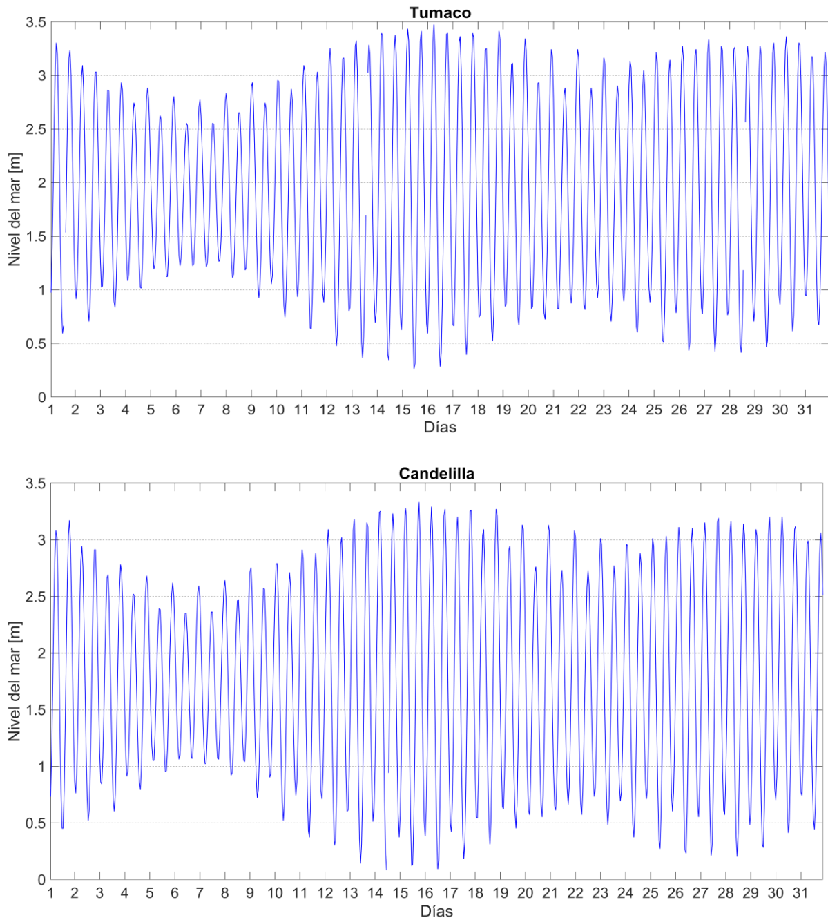
Figura 20. Comportamiento mensual del nivel del mar en la zona sur de la CPC.
