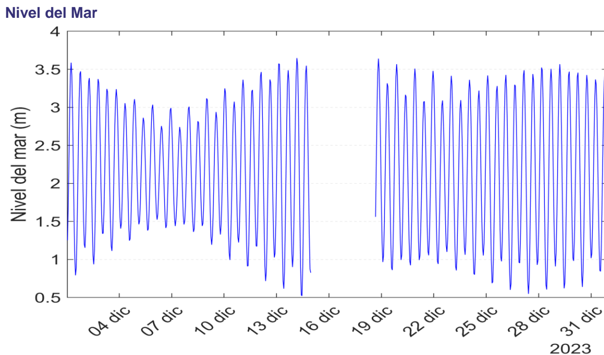
Figura 9. Comportamiento mensual del nivel del mar en la zona norte de la CP
