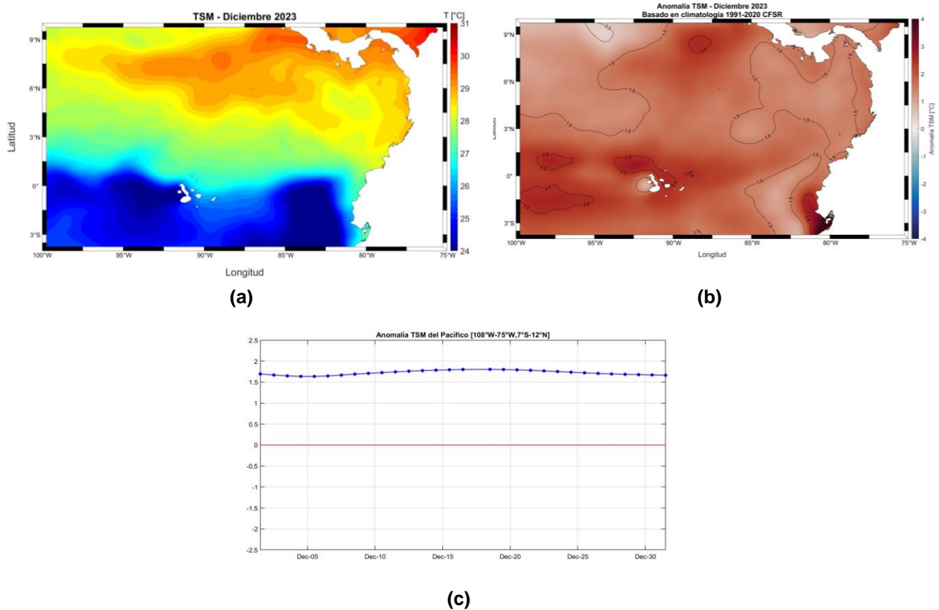
Figura 5. Temperatura superficial del mar en el Pacífico colombiano. (a) Promedio mensual de TSM; (b) anomalías de TSM (c) evolución diaria de TSM para diciembre de 2023. (Tomado de Climate Forecast System Reanalysis (CFSR)).
