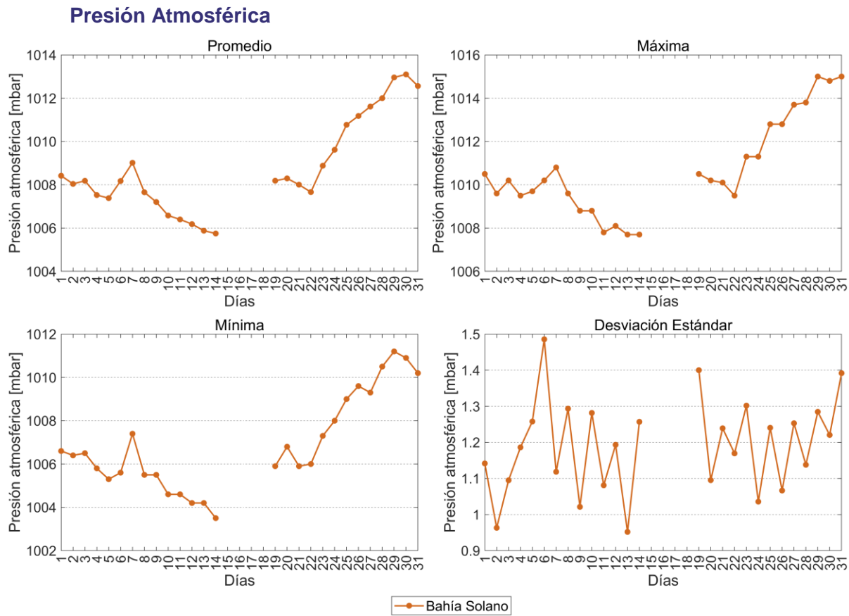
Figura 6. Comportamiento mensual de la presión atmosférica en la zona norte de la CPC.
