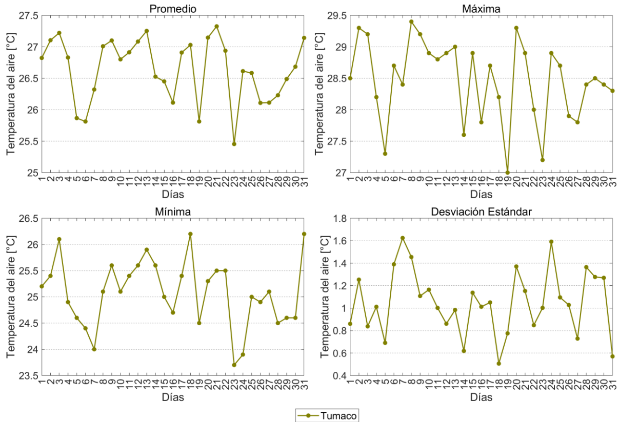
Figura 15. Comportamiento mensual de la temperatura del aire en la zona sur de la CPC.
