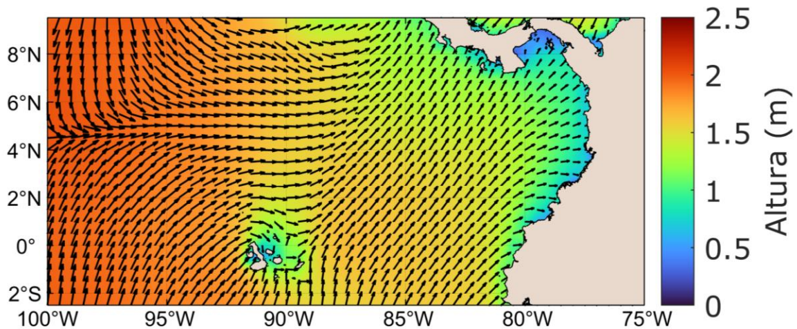
Figura 3. Distribución espacial de oleaje en el Pacífico colombiano durante diciembre 2023. (Tomado de Copernicus Marine Service, 2023).
