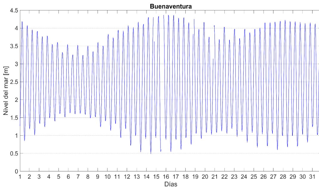
Figura 14. Comportamiento mensual del nivel del mar en la zona centro de la CPC.
