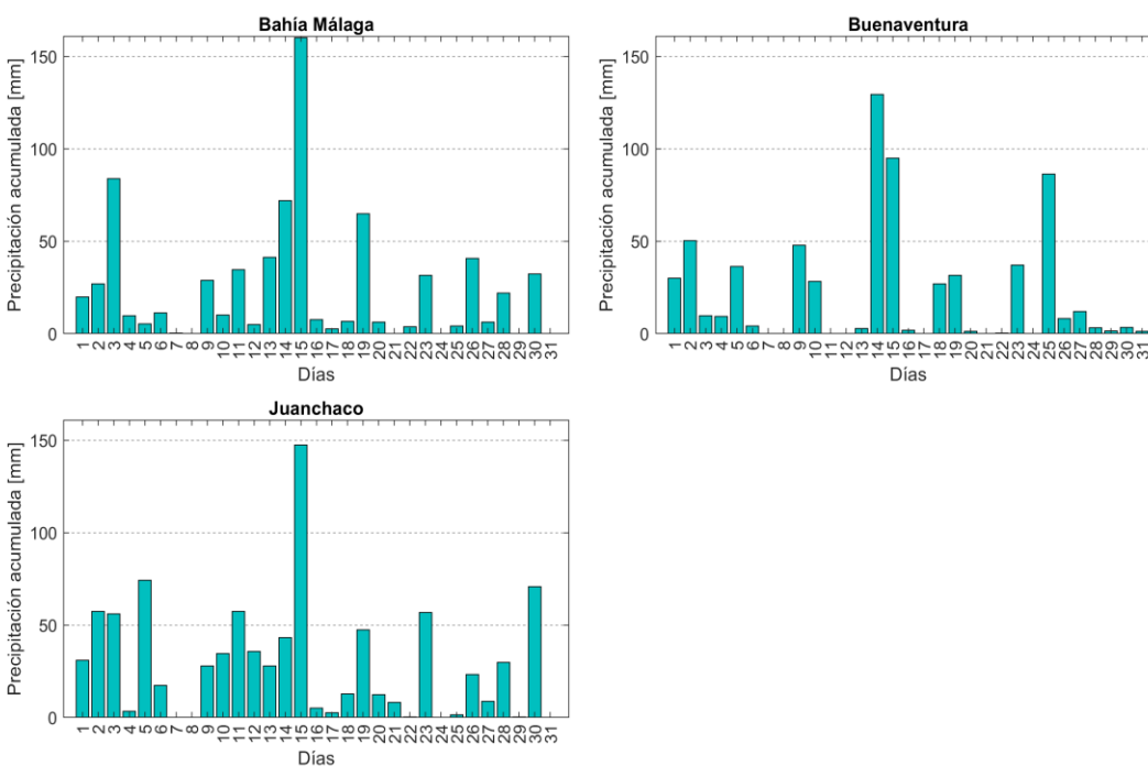
Figura 13. Comportamiento mensual de la precipitación acumulada en la zona centro de la CPC.
