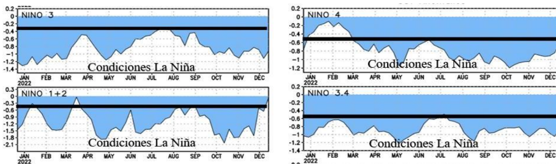
Figura 1. Evolución de las anomalías de la TSM en el Pacífico ecuatorial hasta enero de 2023.
