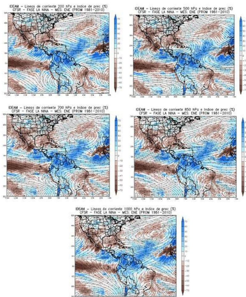
Figura 4. Líneas de corriente en 200, 500, 700, 850 y 1000 hPa y promedio de precipitaciones para el mes de enero bajo condiciones La Niña (1981-2010) extraídas del CFSR
