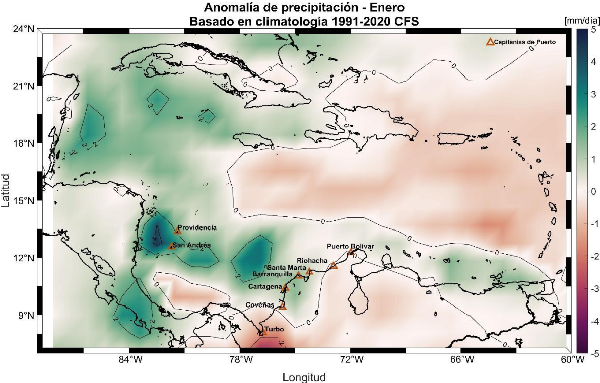
Figura 6. Pronóstico de la anomalía diaria de precipitación para el mes de enero de 2023.
