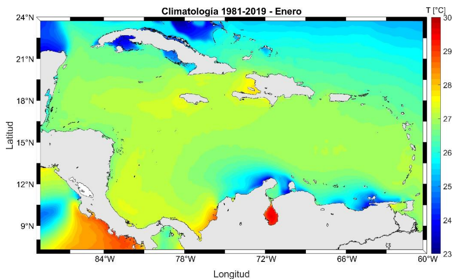
Figura 11. Valores climatológicos de la TSM para el mes enero (1981-2019). Fuente: Good et al., 2020.
