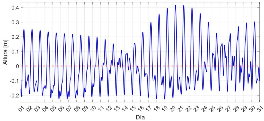
Figura 13. Pronóstico de marea de enero de 2023 para los principales puertos marítimos del Caribe colombiano.
