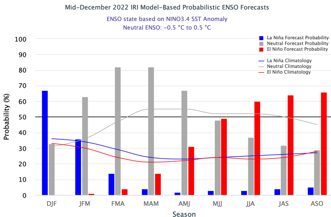
Figura 2. Pronóstico probabilístico de las condiciones ENSO hasta el trimestre ASO de 2023.
