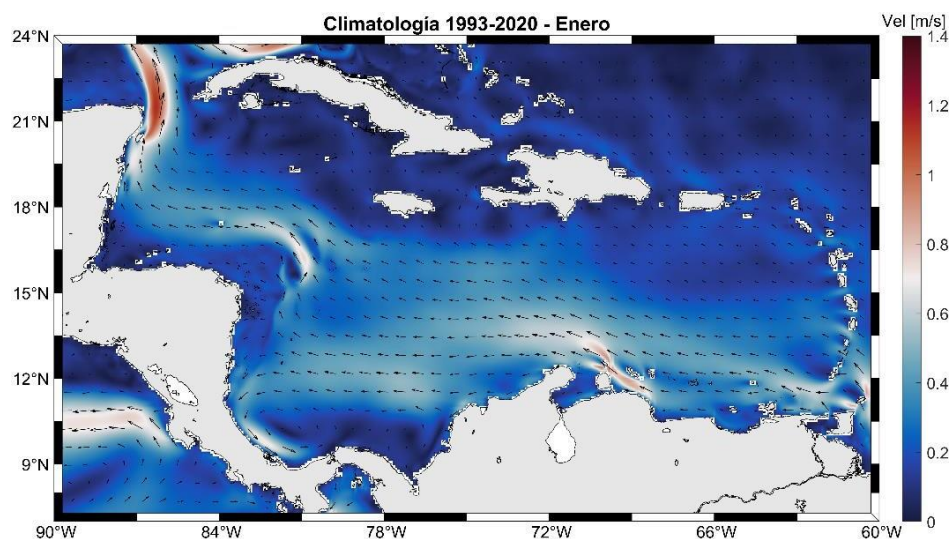
Figura 10. Valores climatológicos de la velocidad y dirección de la corriente superficial predominante para enero (1993-2020).
