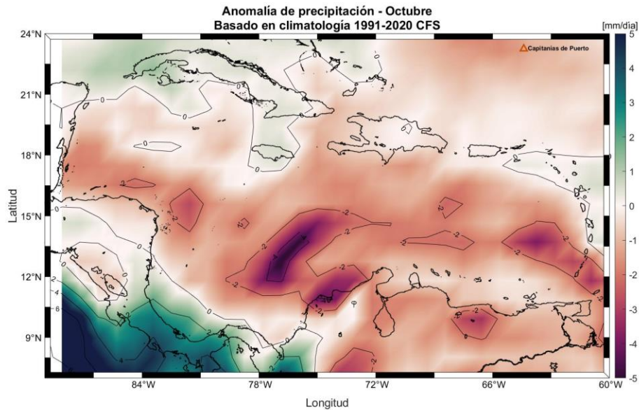
Figura 7. Pronóstico de la anomalía diaria de precipitación para el mes de noviembre de 2023. Fuente: ModeloCFSv2 (NOAA -NCEP, 2023).
