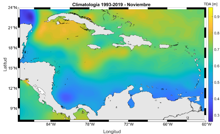
Figura 11. Valores climatológicos de altura dinámica absoluta del mar para el mes de noviembre (1993-2020). Fuente: Copernicus Marine Environment Monitoring Service (CMEMS, 2020).
