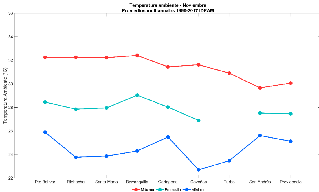
Figura 9. Valores climatológicos de temperatura media, mínima y máxima para el mes de noviembre (1990-2017) en los principales puertos del Caribe. Fuente: DIMAR - CIOH (2023)
