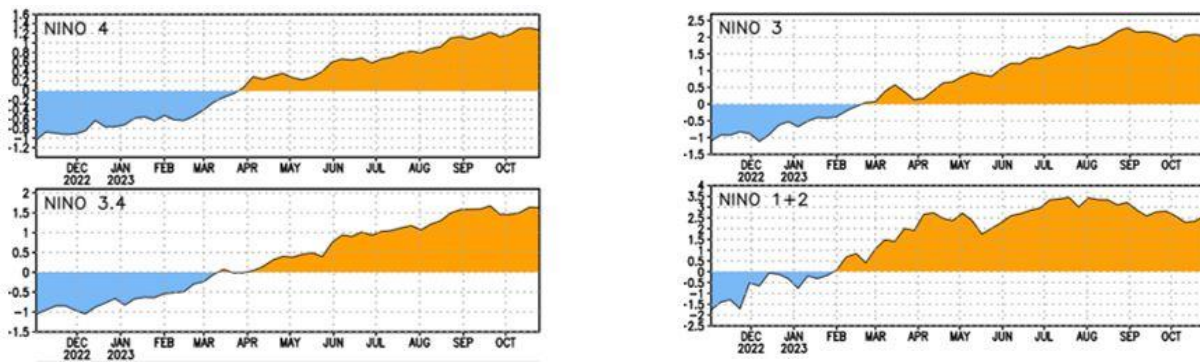
Figura 2. Evolución de las ATSM en el Pacífico ecuatorial hasta noviembre de 2023. Fuente: Modificado de CPC – NCEP, 2023.
