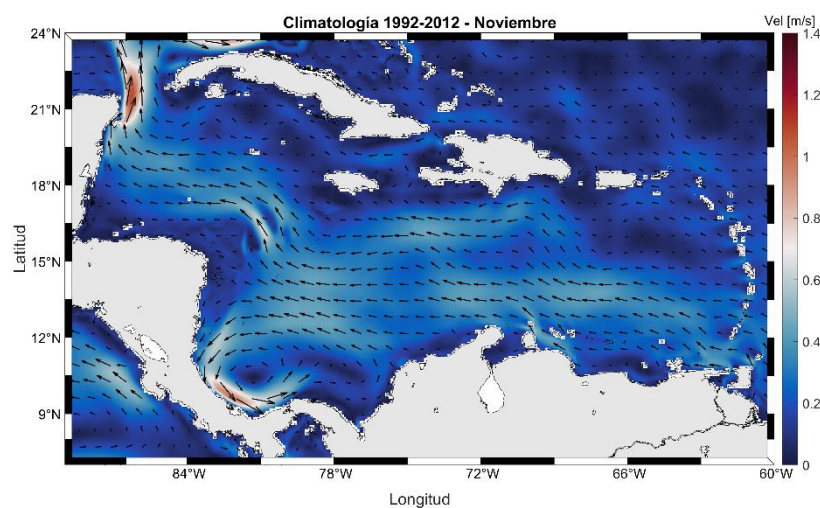
Figura 12. Valores climatológicos de la velocidad y dirección de la corriente superficial predominante para noviembre (1993-2020). Fuente: NRL, 2020
