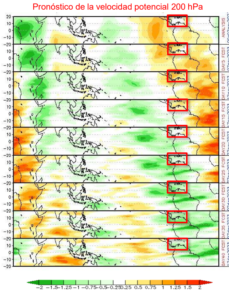
Figura 4. Predicción semanal de la velocidad potencial en 200 hPa, entre el 02 de noviembre hasta el 12 de diciembre de 2023. Fuente: CPC-NCEP, (2023)
