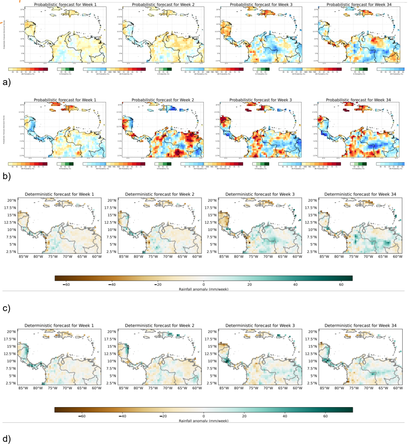
Figura 8. Pronósticos probabilísticos y determinísticos subestacionales de los modelos GEFS y CFS. a) ProbFcastCFSv2_SubX-CHIRPS-PCR; b) ProbFcastGEFSv12-CHIRPS-PCR; c) Deterministic-CFSv2_SubX-CHIRPS-PCR y d) Deterministic-GEFSv12-CHIRPS-PCR. Fuente: CIOH, 2023.
