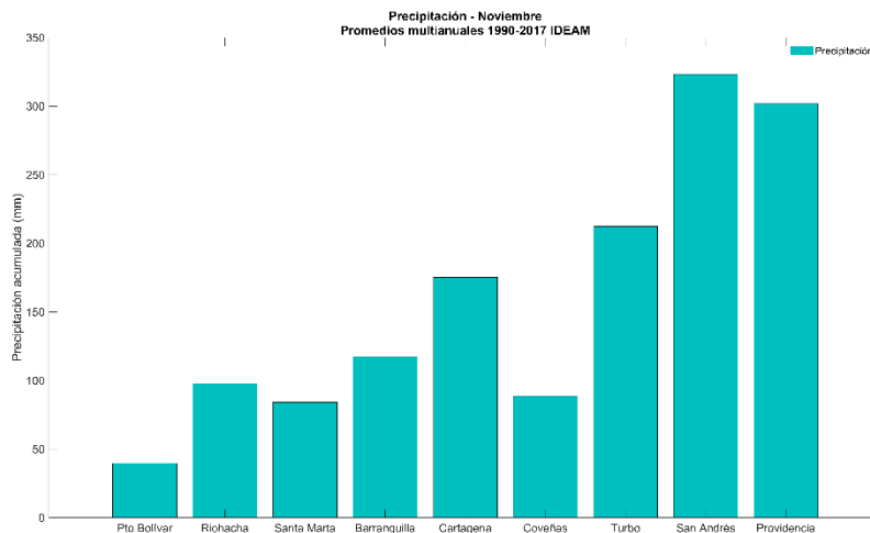
Figura 6. Valores climatológicos de precipitación para el mes de noviembre (1990-2017) en los principales puertos del Caribe. Fuente: DIMAR – CIOH (2023).
