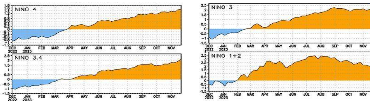
Figura 2. Evolución de las ATSM en el Pacífico ecuatorial hasta diciembre de 2023. Fuente: Modificado de CPC – NCEP, 2023.
