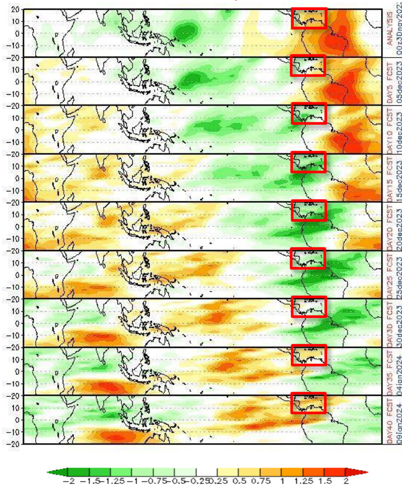
Figura 4. Predicción semanal de la velocidad potencial en 200 hPa, entre el 5 de diciembre de 2023 hasta el 09 de enero de 2024. Fuente: CPC-NCEP, (2023)
