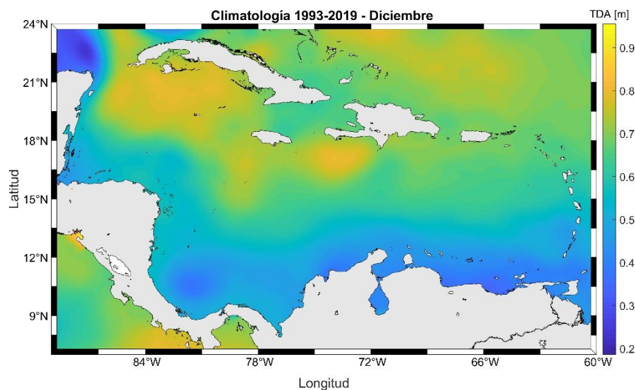
Figura 11. Valores climatológicos de altura dinámica absoluta del mar para el mes de diciembre (1993-2019). Fuente: Copernicus Marine Environment Monitoring Service (CMEMS, 2020).
