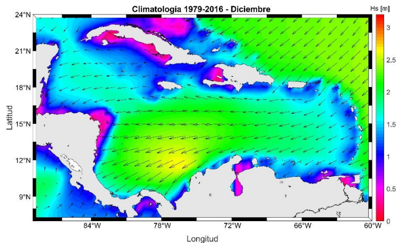
Figura 10. Valores climatológicos de dirección y altura de la ola en el mar Caribe para el mes de diciembre (1979-2016). Fuente: WW III (NWS - NOAA, 2009)
