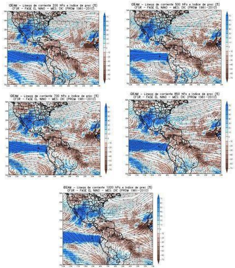
Figura 5. Líneas de corriente e índice de precipitación para el mes de diciembre (1981-2010) bajo condiciones El Niño en 200, 500, 700, 850 y 1000 hPa, extraídas del CFSR. Fuente: Ruíz & Melo, 2019.
