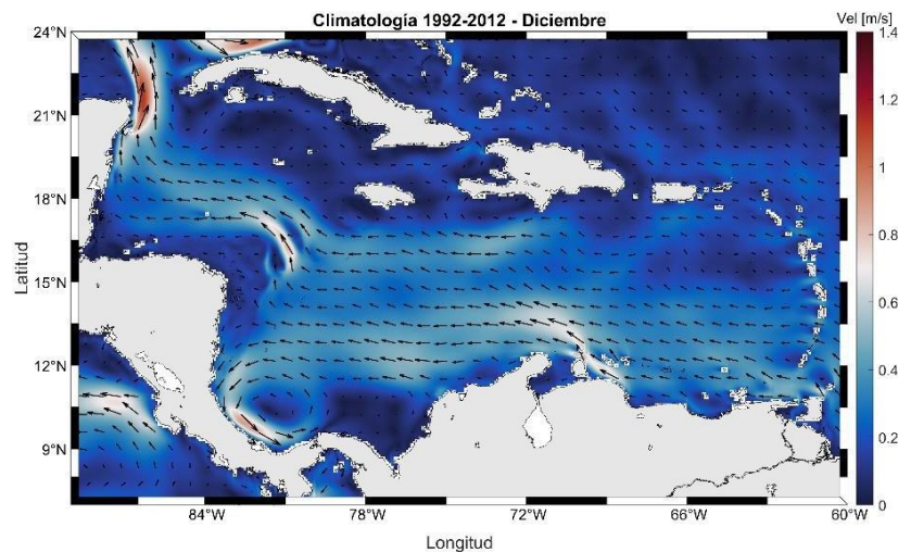
Figura 12. Valores climatológicos de la velocidad y dirección de la corriente superficial predominante para diciembre (1992-2012). Fuente: NRL, 2020
