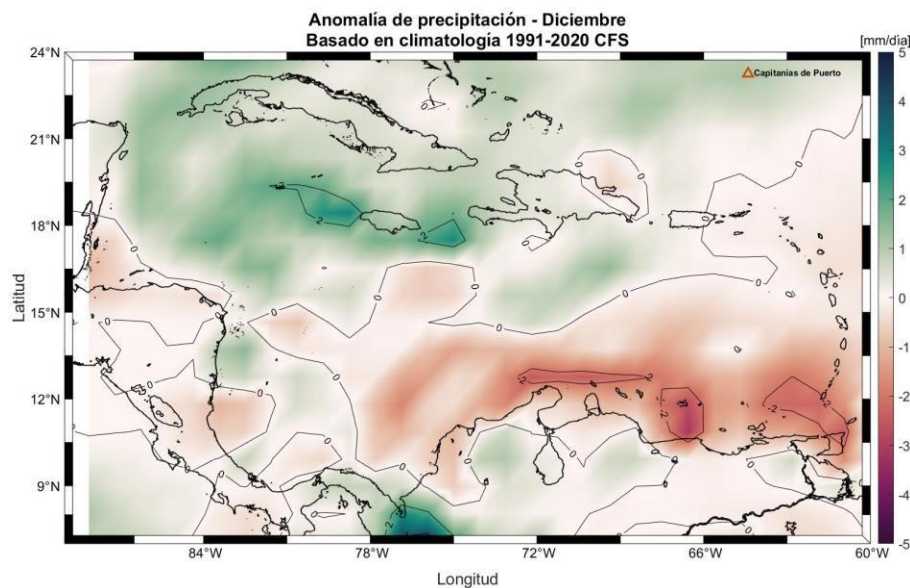
Figura 7. Pronóstico de la anomalía diaria de precipitación para el mes de diciembre de 2023. Fuente: ModeloCFSv2 (NOAA -NCEP, 2023).
