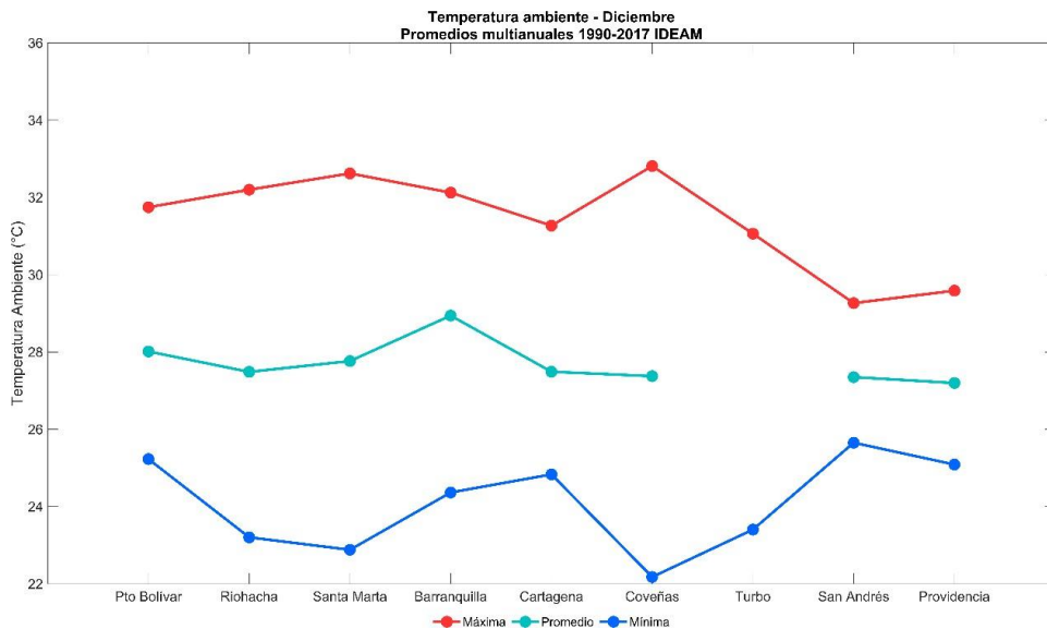
Figura 9. Valores climatológicos de temperaturas máxima, promedio y mínima para el mes de diciembre (1990-2017) en los principales puertos de la cuenca del Caribe colombiano. Fuente: DIMAR - CIOH (2023)
