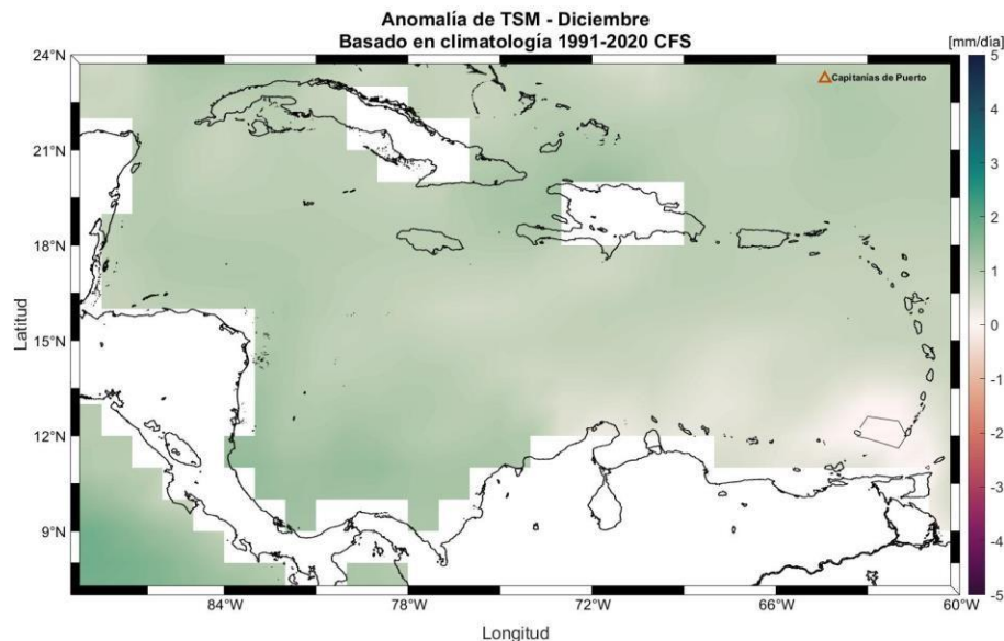
Figura 14. Pronóstico de las anomalías de TSM para el mes de diciembre de 2023. Fuente: NOAA-CPC, 2021
