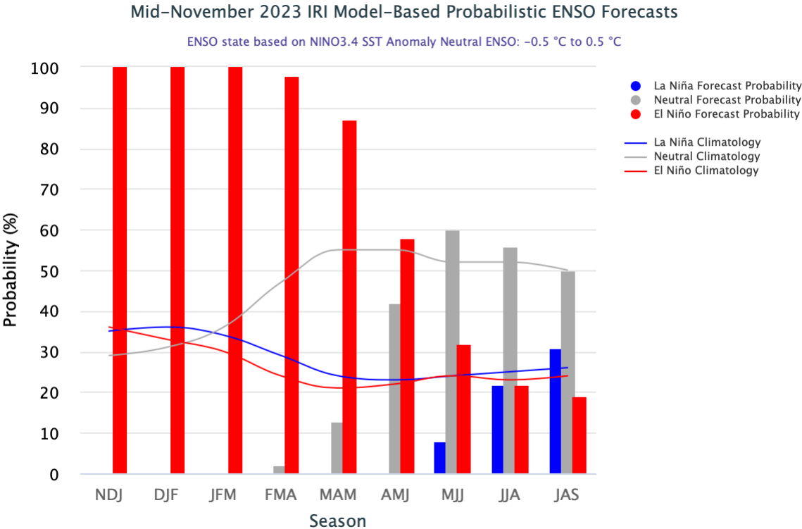
Figura 3. Pronóstico probabilístico de las condiciones ENSO hasta el trimestre JAS de 2024.
