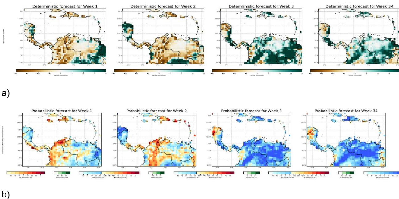
Figura 8. Pronósticos probabilísticos y determinísticos subestacionales de los modelos GEFS y CFS.
