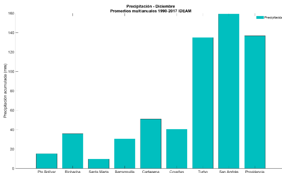
Figura 6. Valores climatológicos de precipitación para el mes de diciembre (1990-2017) en los principales puertos del Caribe. Fuente: DIMAR – CIOH (2023).
