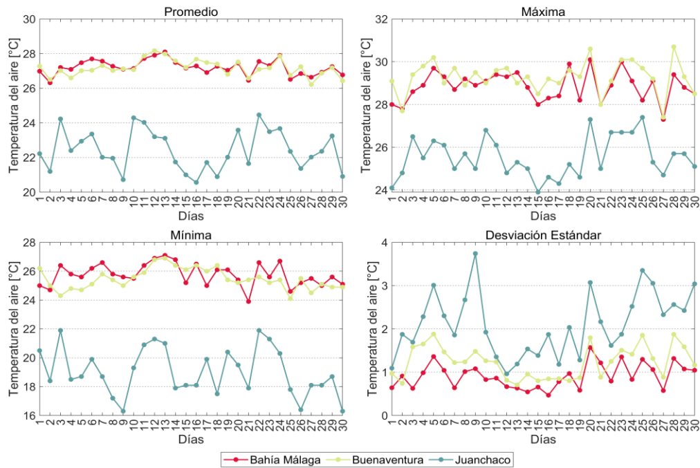
Figura 6. Comportamiento mensual de la Temperatura del aire en la zona centro de la CPC.
