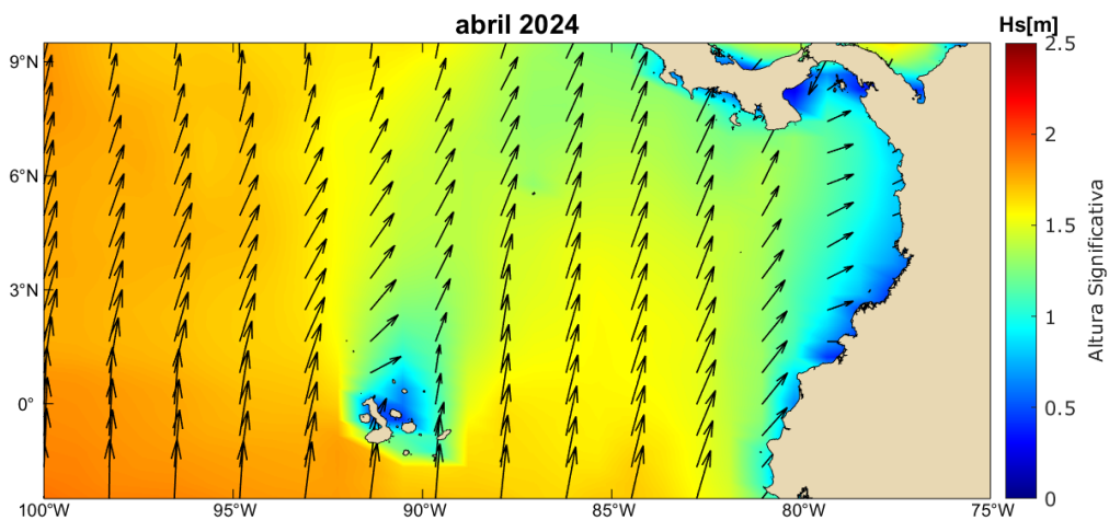
Figura 3. Distribución espacial de oleaje en el Pacífico colombiano durante abril 2024. (Tomado de Copernicus Marine Service, 2023).
