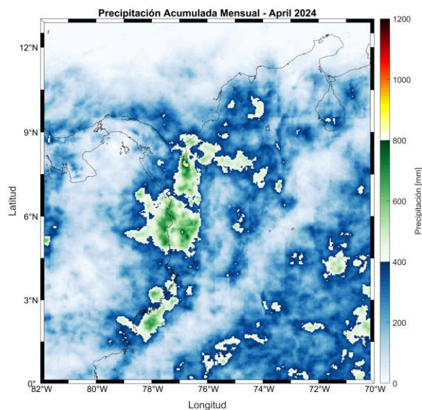
Figura 4. Distribución espacial de la precipitación acumulada mensual en el Pacífico colombiano durante abril 2024. (Procesado con datos de NESDIS. NOAA, 2023).
