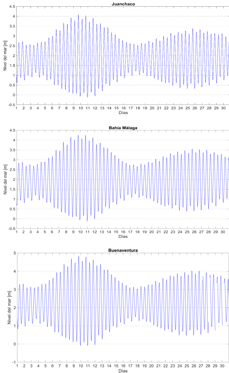
Figura 11. Comportamiento mensual del nivel del mar en la zona centro de la CPC.
