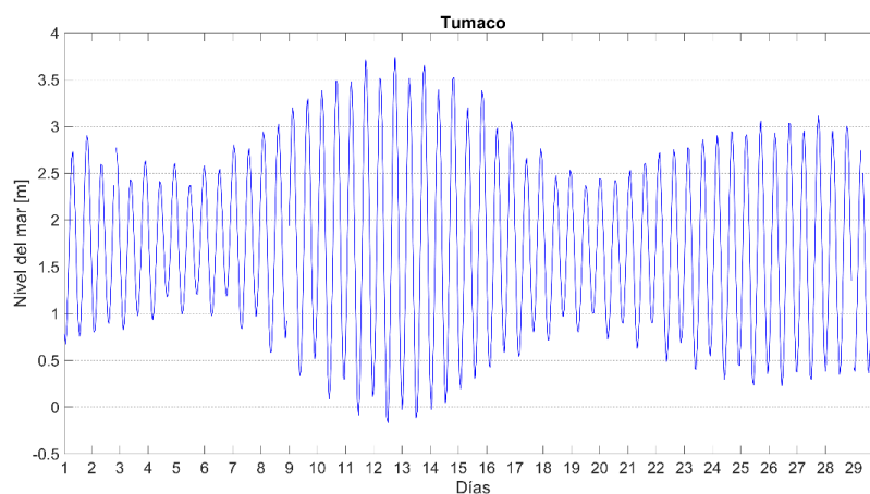
Figura 16. Comportamiento mensual del nivel del mar en la zona sur de la CPC.
