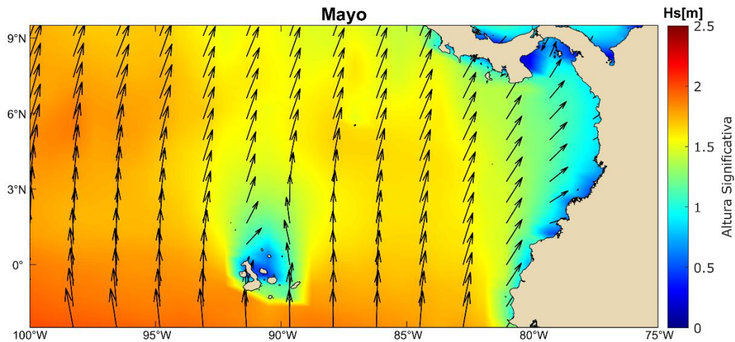
Figura 3. Distribución espacial de oleaje en el Pacífico colombiano durante mayo 2024. (Tomado de Copernicus Marine Service, 2023).
