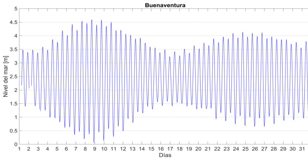
Figura 11. Comportamiento mensual del nivel del mar en la zona centro de la CPC.
