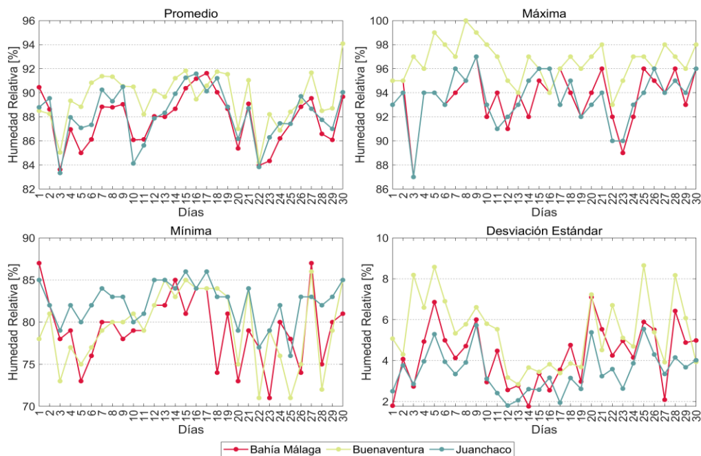
Figura 9. Comportamiento mensual de la humedad relativa en la zona centro de la CPC.
