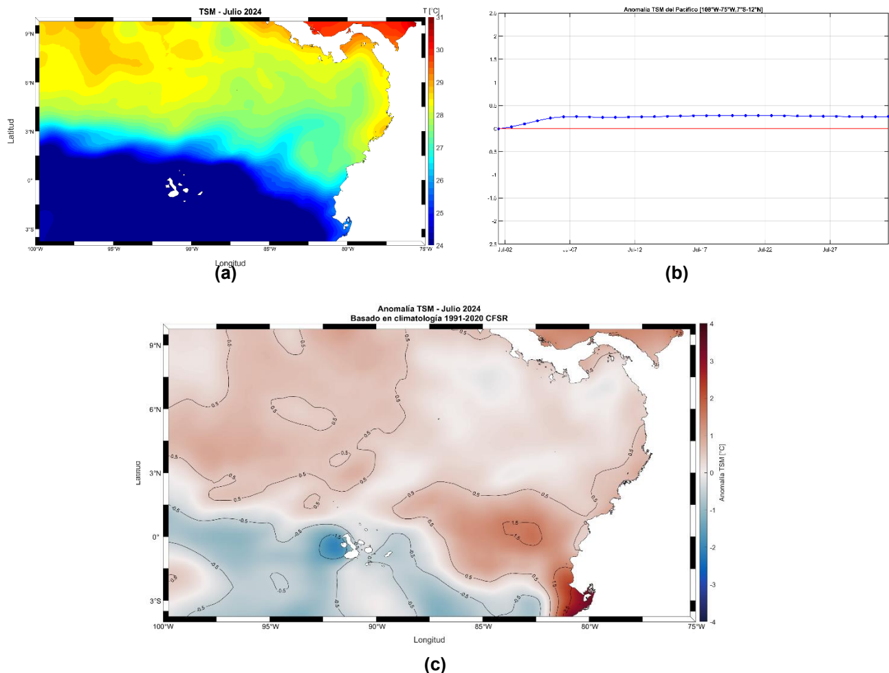
Figura 5. Temperatura superficial del mar en el Pacífico colombiano. (a) Promedio mensual de TSM; (b) anomalías de TSM (c) evolución diaria de TSM para julio de 2024. (Tomado de Climate Forecast System Reanalysis (CFSR)).
