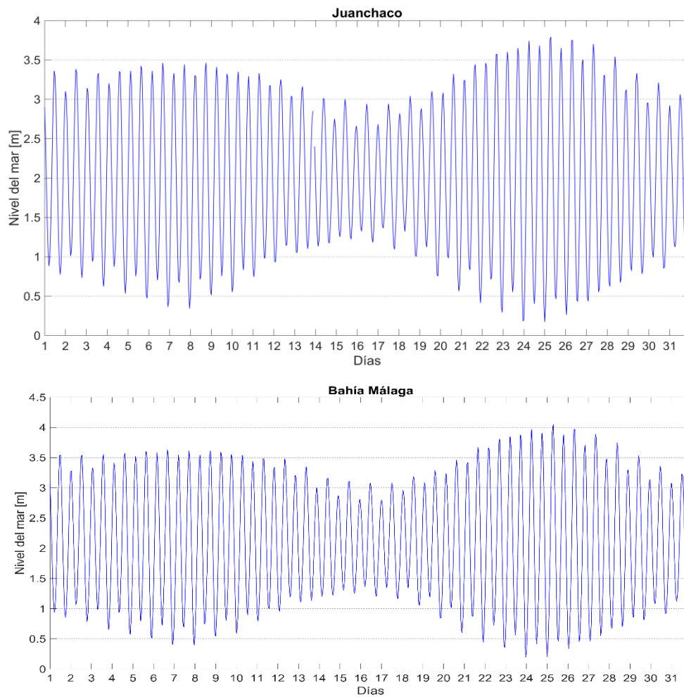
Figura 11. Comportamiento mensual del nivel del mar en la zona centro de la CPC.
