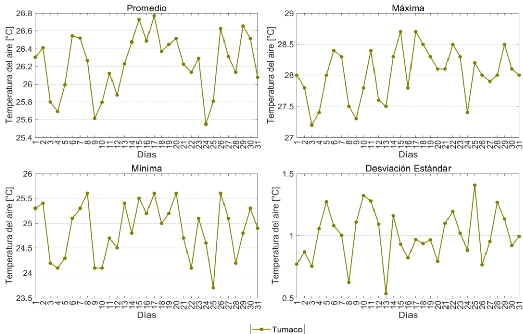
Figura 12. Comportamiento mensual de la temperatura del aire en la zona sur de la CPC.
