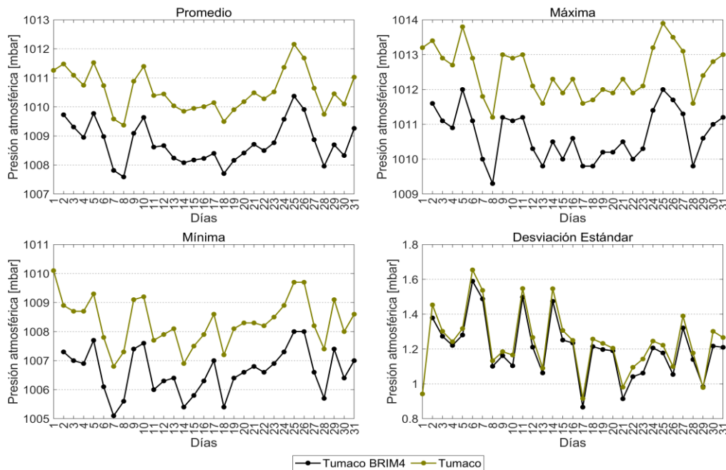
Figura 13. Comportamiento mensual de la presión atmosférica en la zona sur de la CPC
