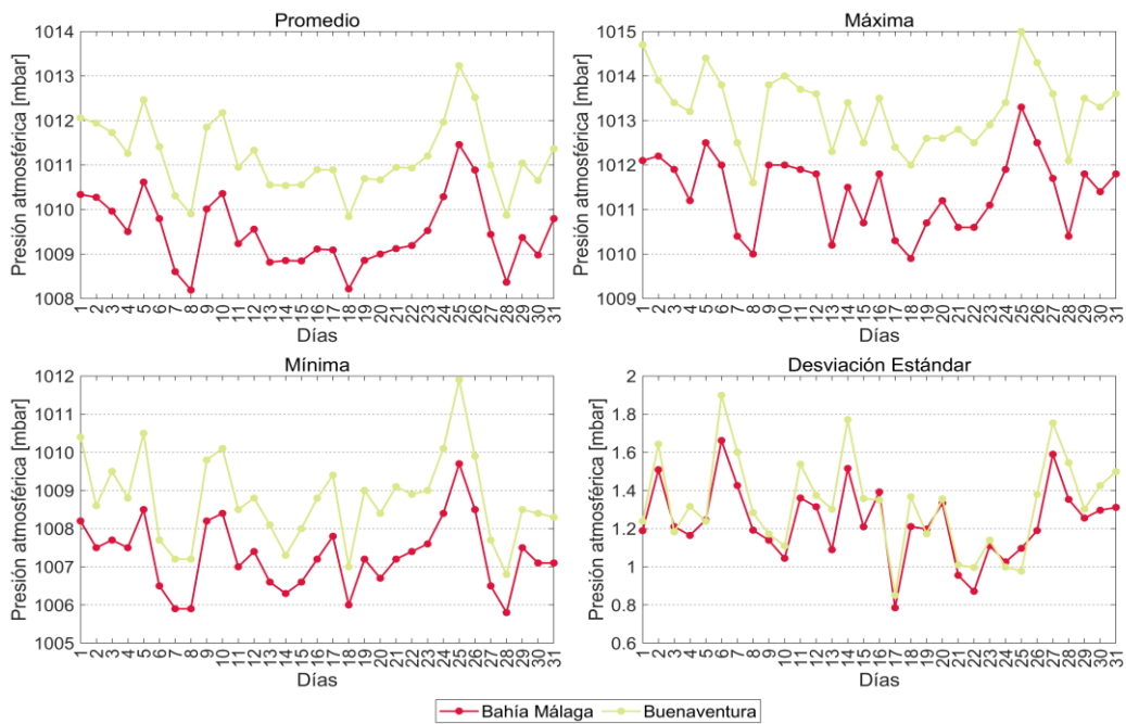
Figura 7. Comportamiento mensual de la presión atmosférica en la zona centro de la CPC.
