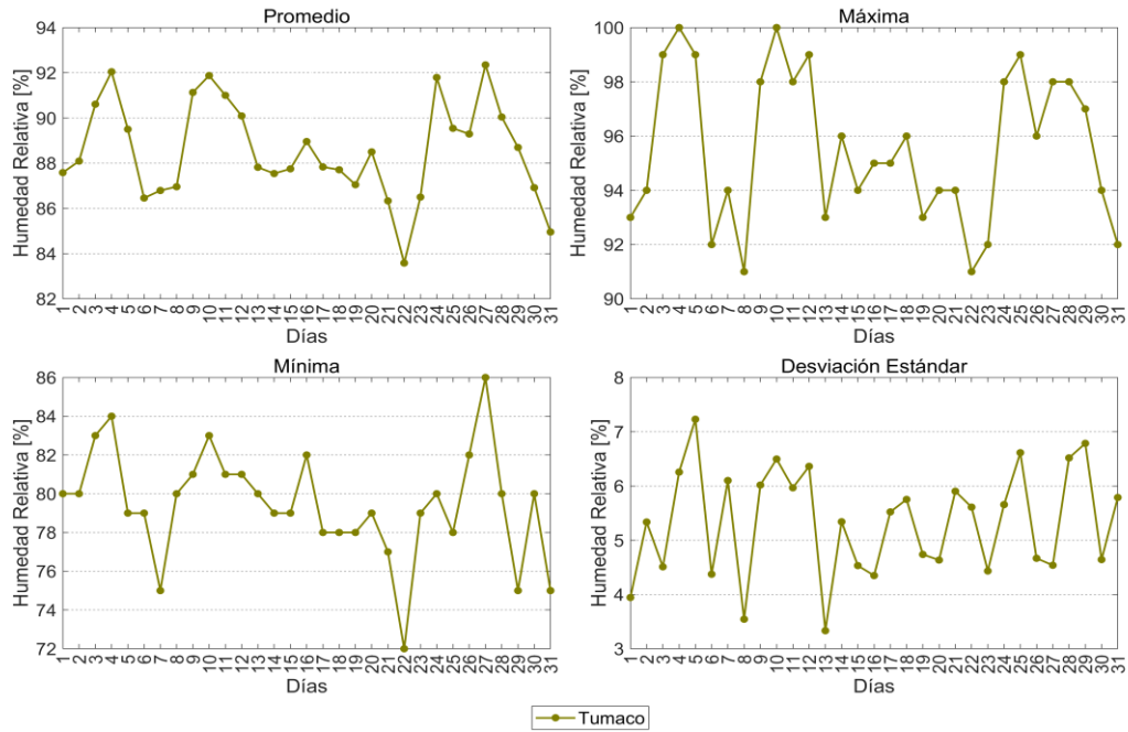
Figura 15. Comportamiento mensual de la humedad relativa en la zona sur de la CPC.
