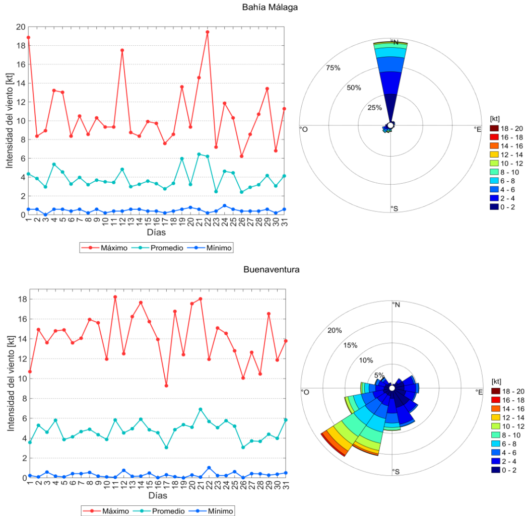
Figura 8. Comportamiento mensual del régimen de vientos superficiales en la zona centro de la CPC.
