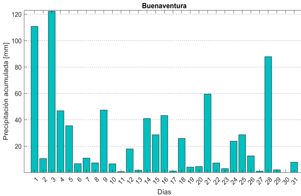
Figura 10. Comportamiento mensual de la precipitación acumulada en la zona centro de la CPC.
