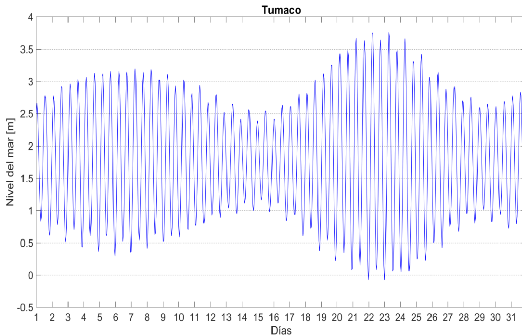
Figura 17. Comportamiento mensual del nivel del mar en la zona sur de la CPC.
