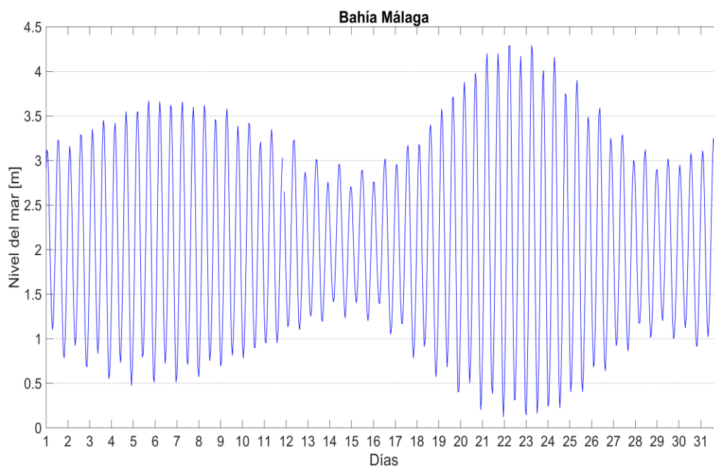
Figura 11. Comportamiento mensual del nivel del mar en la zona centro de la CPC.
