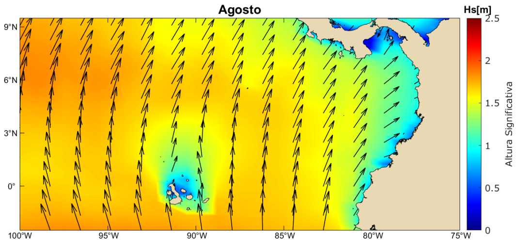
Figura 3. Distribución espacial de oleaje en el Pacífico colombiano durante agosto 2024. (Tomado de Copernicus Marine Service, 2023).
