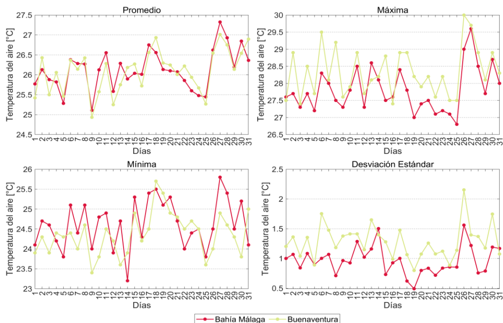
Figura 6. Comportamiento mensual de la Temperatura del aire en la zona centro de la CPC.
