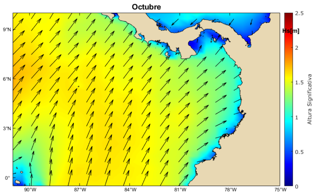
Distribución espacial de oleaje en el Pacífico colombiano durante octubre 2024. (Tomado de Copernicus Marine Service, 2023).
