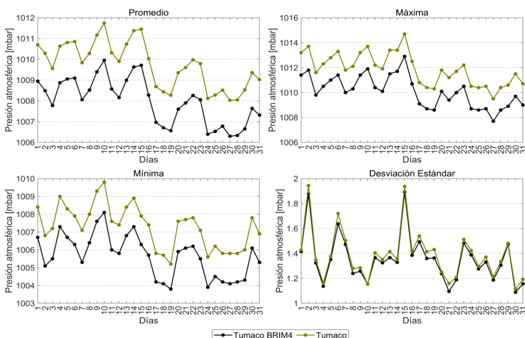
Figura 12. Comportamiento mensual de la presión atmosférica en la zona sur de la CPC
