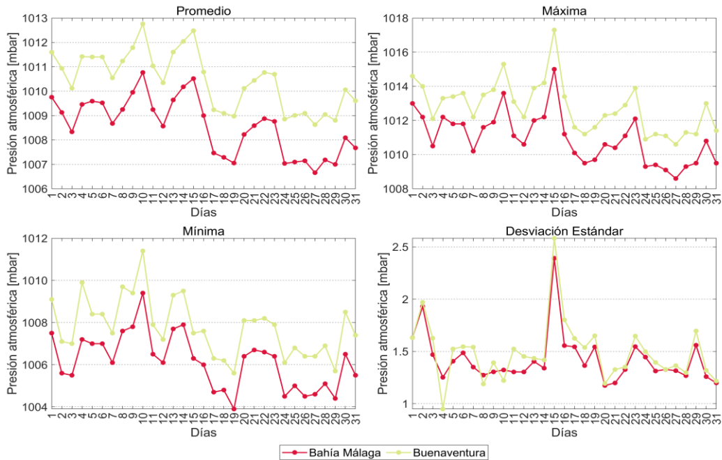
Figura 6. Comportamiento mensual de la presión atmosférica en la zona centro de la CPC.
