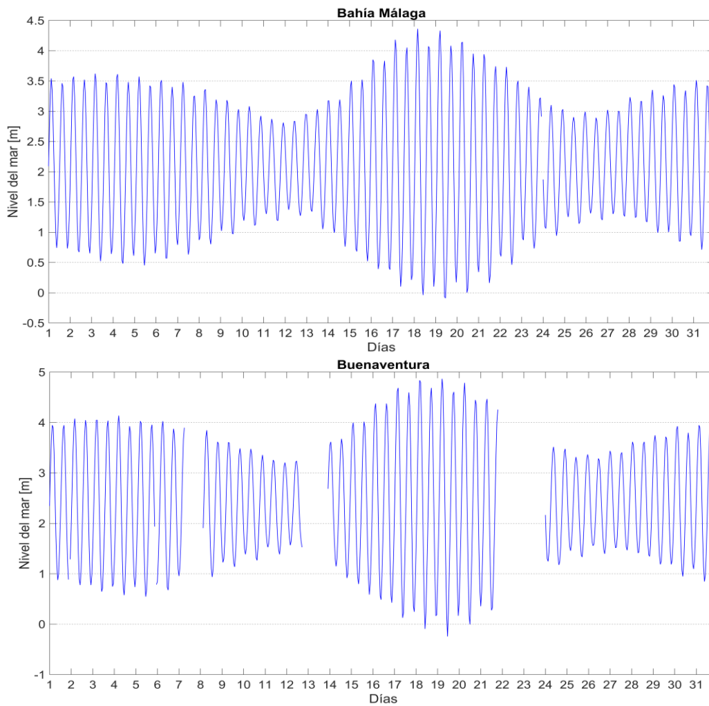
Figura 10. Comportamiento mensual del nivel del mar en la zona centro de la CPC.
