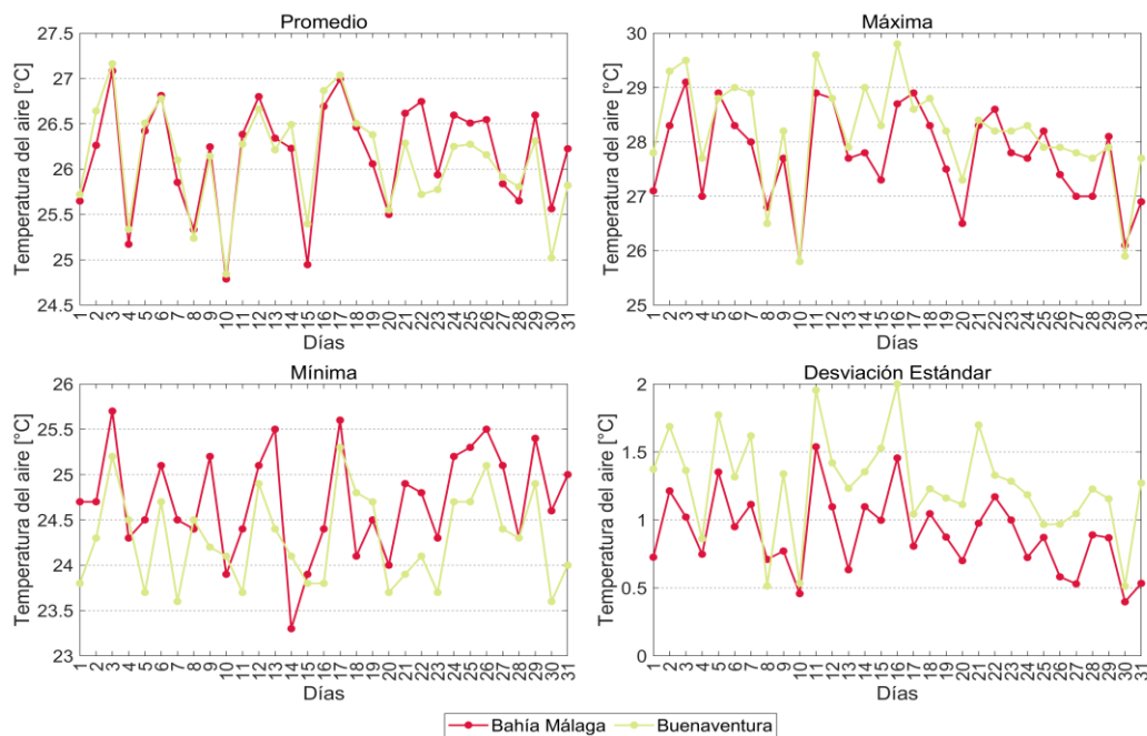
Figura 5. Comportamiento mensual de la Temperatura del aire en la zona centro de la CPC.
