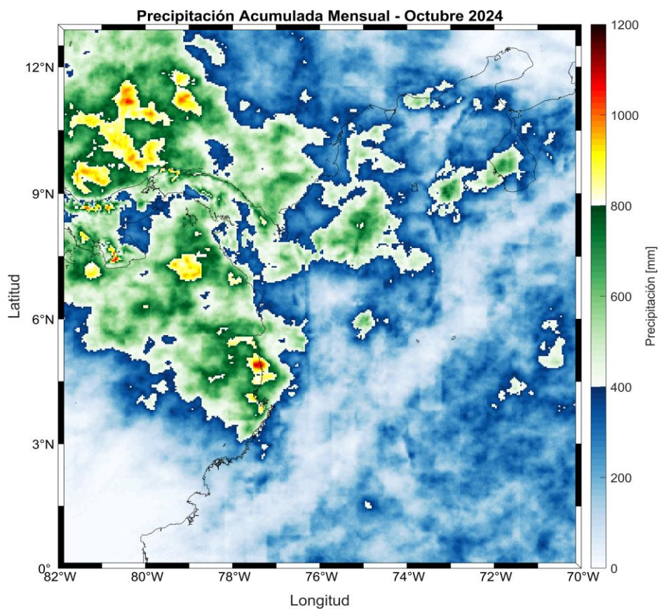
Figura 3. Distribución espacial de la precipitación acumulada mensual en el Pacífico colombiano durante octubre 2024. (Procesado con datos de NESDIS. NOAA, 2023).
