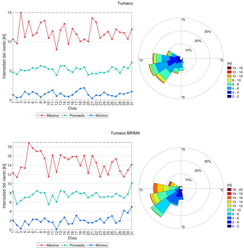
Figura 13. Comportamiento mensual del régimen de vientos superficiales en la zona sur de la CPC.
