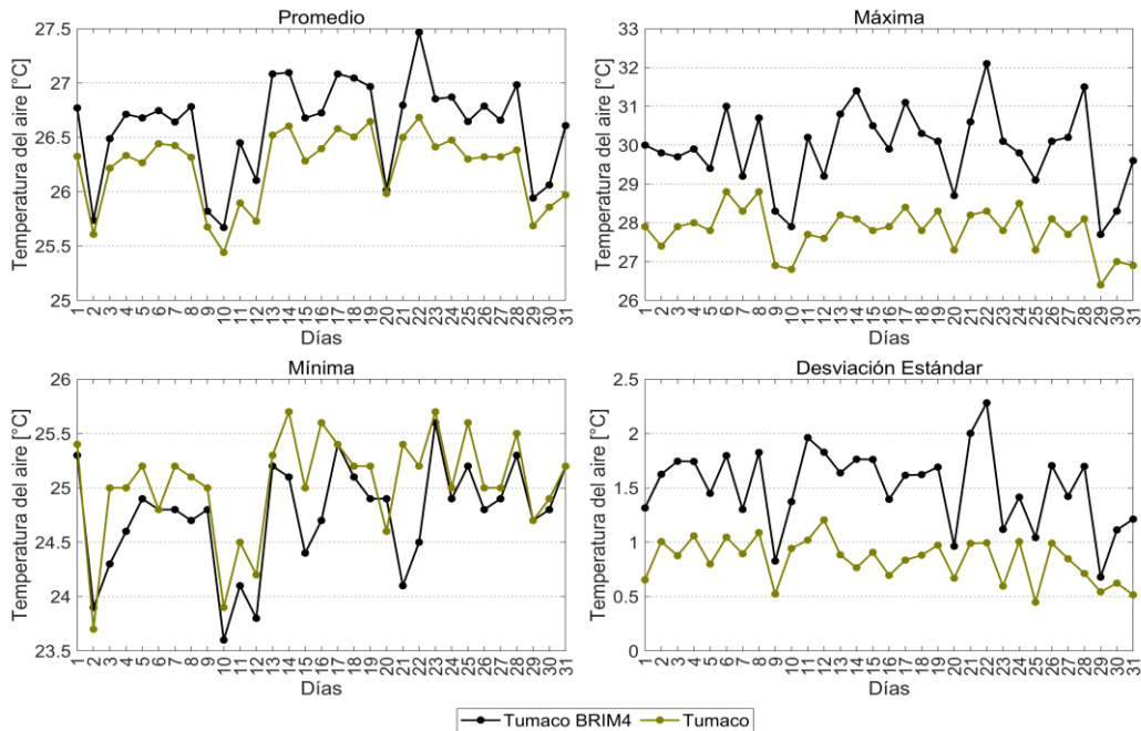
Figura 11. Comportamiento mensual de la temperatura del aire en la zona sur de la CPC.
