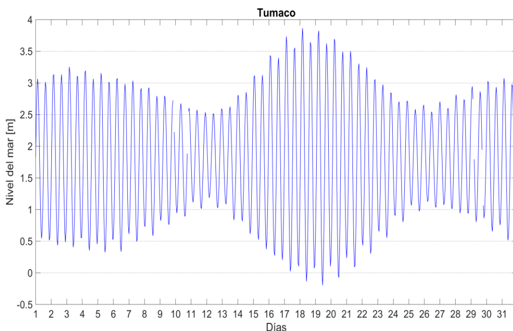
Figura 16. Comportamiento mensual del nivel del mar en la zona sur de la CPC.
