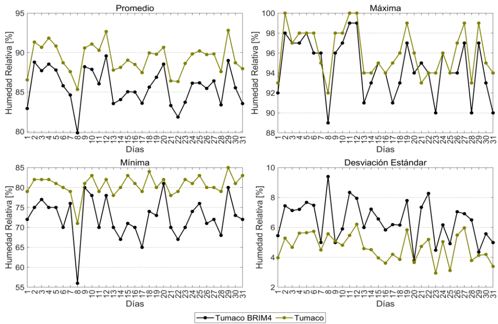
Figura 14. Comportamiento mensual de la humedad relativa en la zona sur de la CPC.
