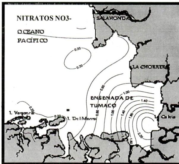
FIG.4 DISTRIBUCION ESPACIAL DE NO3-
