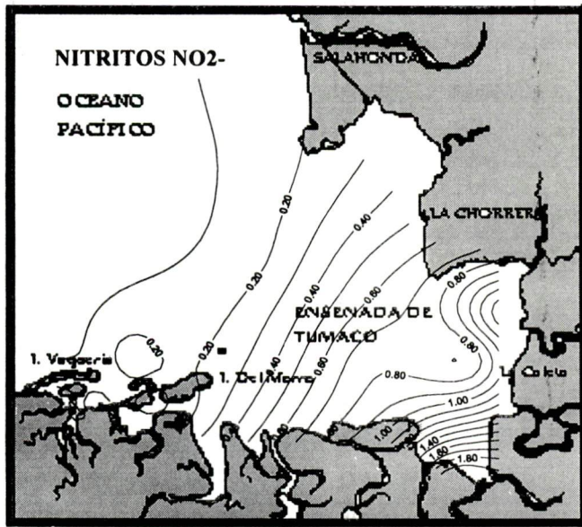
FIG.6 DISTRIBUCION ESPACIAL DE NO 2 -
