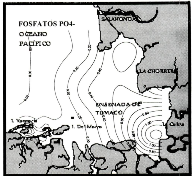
FIG.7 DISTRIBUCION ESPACIAL DE (PO 4 )-3
