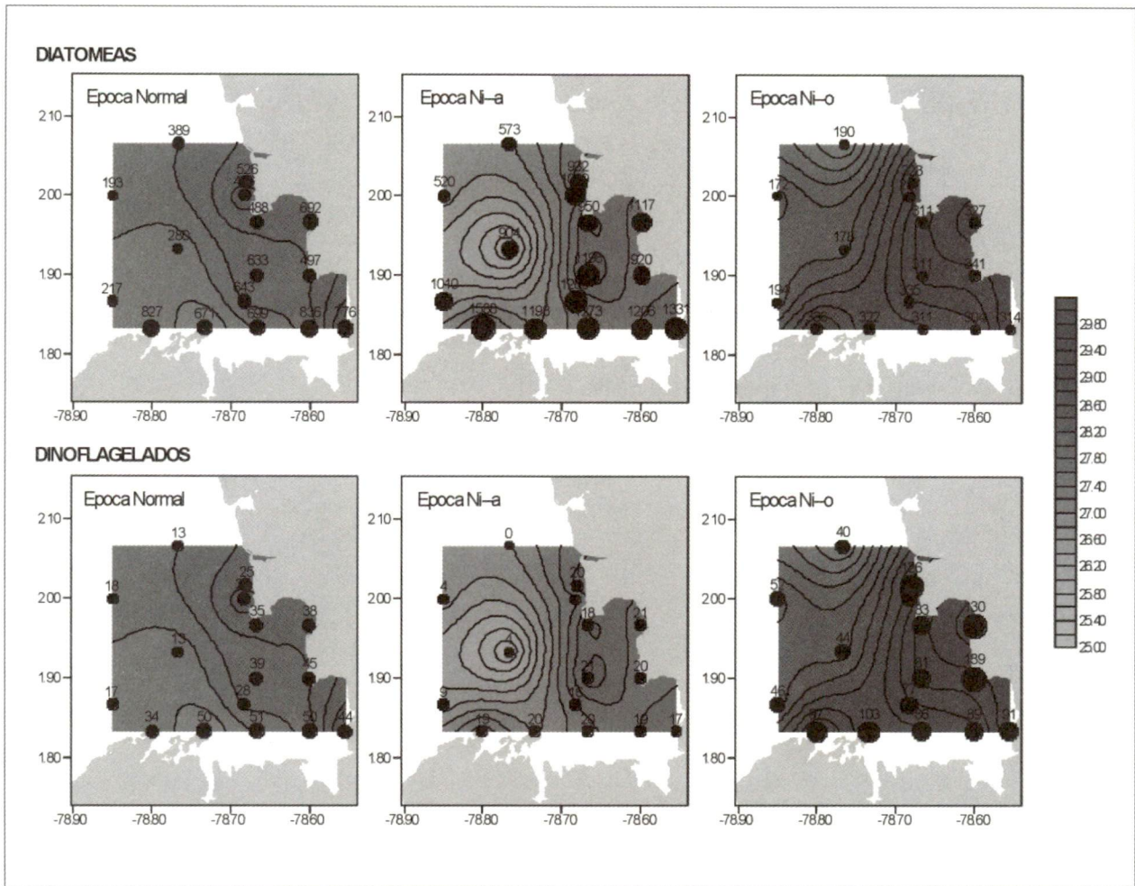
Figura 3. Distribución de la TSM (isolíneas con escala de grises) para cada época climática en relación con abundancia promedio de diatomeas y dinoflagelados (puntos negros).
