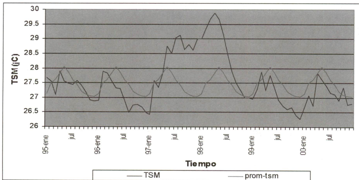
Figura 2. Variación de la temperatura superficial del mar (TSM) y promedio histórico del área de estudio para el período 1995 - 2000.
