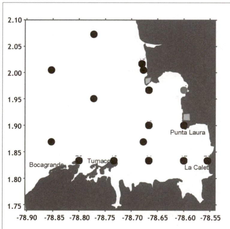
Figura 1. Ubicación de las estaciones de muestreo en el área de estudio, Pacífico colombiano.
