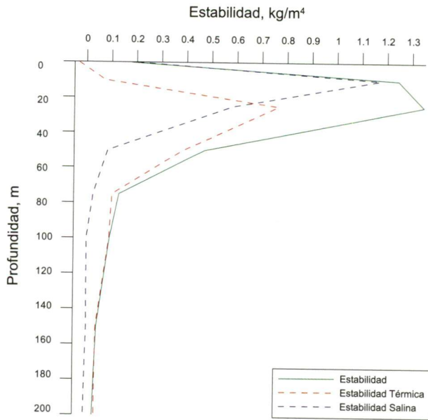
Figura 2. Perfil de estabilidad E. Estación 1. Mayo de 2000, Pacífico colombiano.
