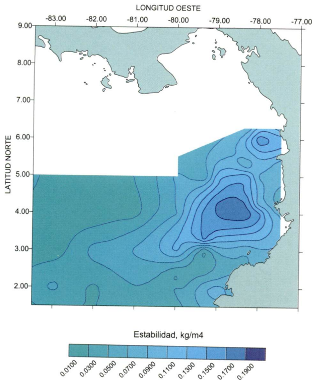
Figura 8. Estabilidad capa 100–150 m. Mayo de 2000, Pacífico colombiano.
