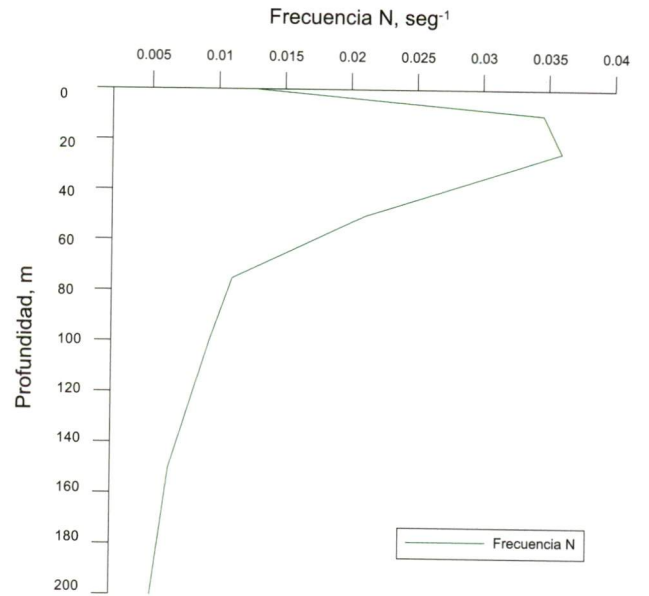
Figura 3. Perfil de frecuencia N. Estación 1. Mayo de 2000, Pacífico colombiano.
