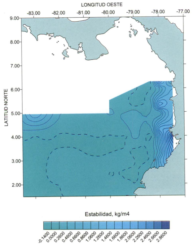
Figura 13. Estabilidad capa 0–10 m. Mayo de 2000, Pacífico colombiano.
