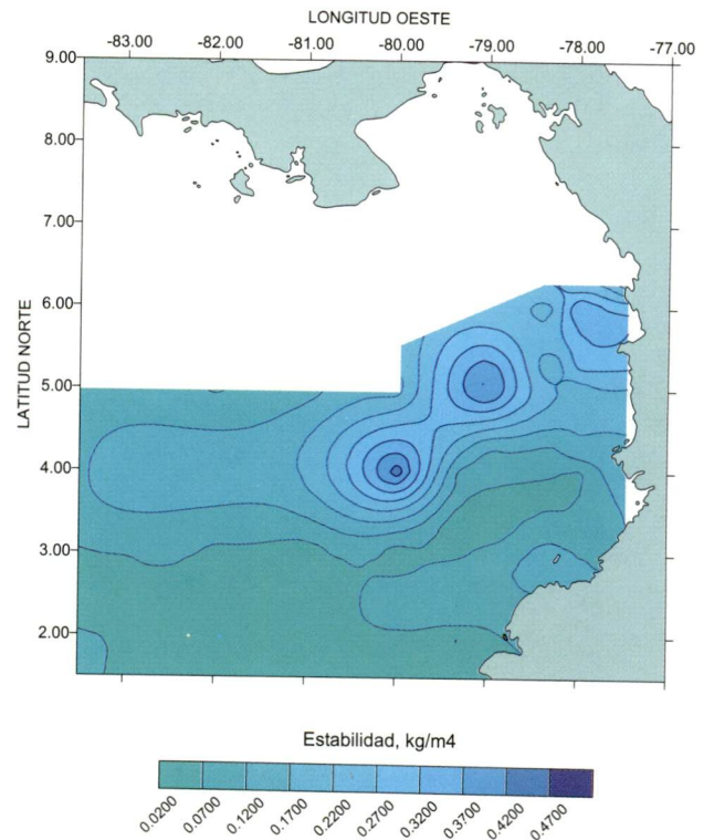
Figura 9. Estabilidad capa 75–100 m. Mayo de 2000, Pacífico colombiano.
