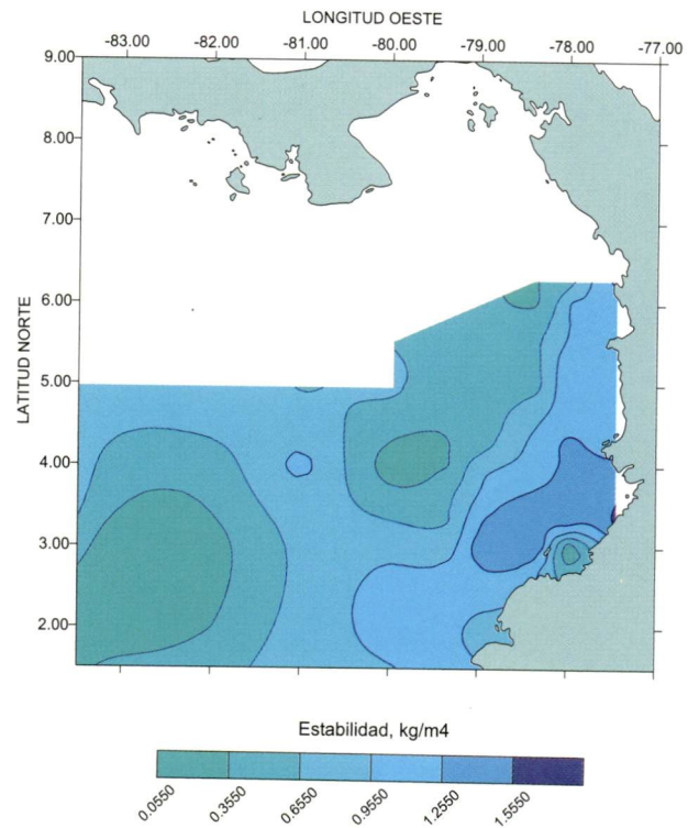
Figura 11. Estabilidad capa 25–50 m. Mayo de 2000, Pacífico colombiano.
