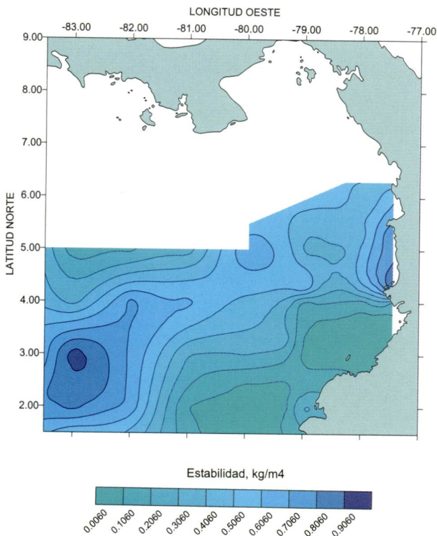
Figura 10. Estabilidad capa 50–75 m. Mayo de 2000, Pacífico colombiano.
