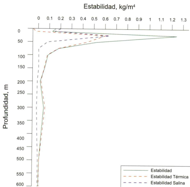
Figura 4. Perfil de estabilidad E. Estación 12. Mayo de 2000, Pacífico colombiano.
