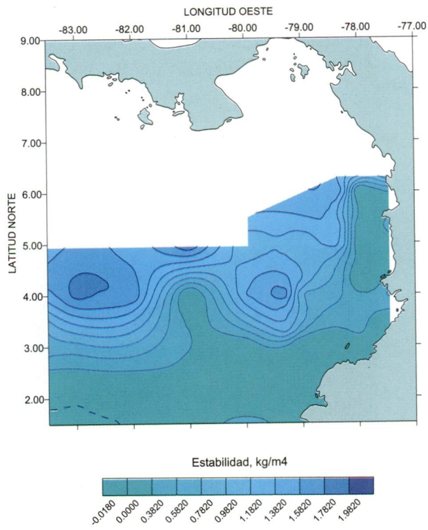
Figura 12. Estabilidad capa 10–25 m. Mayo de 2000, Pacífico Colombiano.
