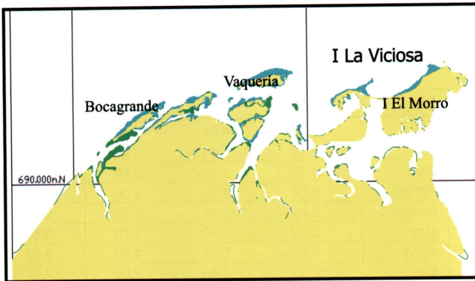
Figura 7. Comparación de las líneas de costa de 1992 y 1995. Se aprecia el predominio de procesos sedimentarios (color azul) y la reorientación de la costa hacia formas más paralelas al oleaje incidente como en el caso de la isla La Viciosa.
