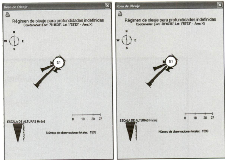
Figura 3. Régimen direccional en aguas indefinidas frente a Tumaco (izquierda) y en inmediaciones de la bahía (derecha), obsérvese la refracción que sufre el oleaje y de allí el cambio en la dirección de los principales oleajes que llegan del SSW y en la bahía predominan del SW, asimismo se observa el aumento en el porcentaje de las calmas.
