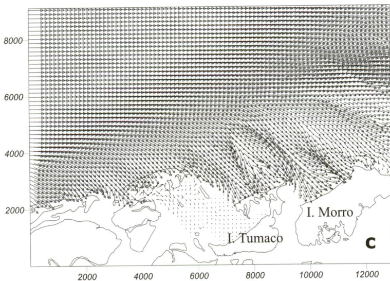
Figura 4. a) Área modelada, obsérvese las mallas anidadas para obtener mayor detalle sobre las islas de Tumaco y las direcciones predominantes del oleaje utilizadas. B) Salida del modelo de la grilla externa, obsérvese las modificaciones al oleaje causadas por la disminución de la profundidad sobre la costa. C) Resultados de la modelación en marea alta y en la grilla de detalle, obsérvese los cambios en los patrones del oleaje, las zonas de concentración y dispersión de energía.
