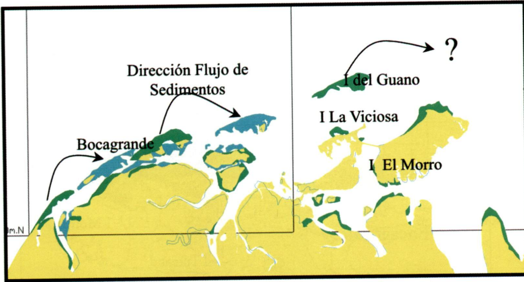
Figura 6. Comparación entre las líneas de costa de 1969 y 1995, realizada inicialmente en escala 1:250000. Se aprecian (en color azul) las zonas acresionadas y (en color verde) las zonas erosionadas incluida la isla del Guano, frente a la isla de El Morro.
